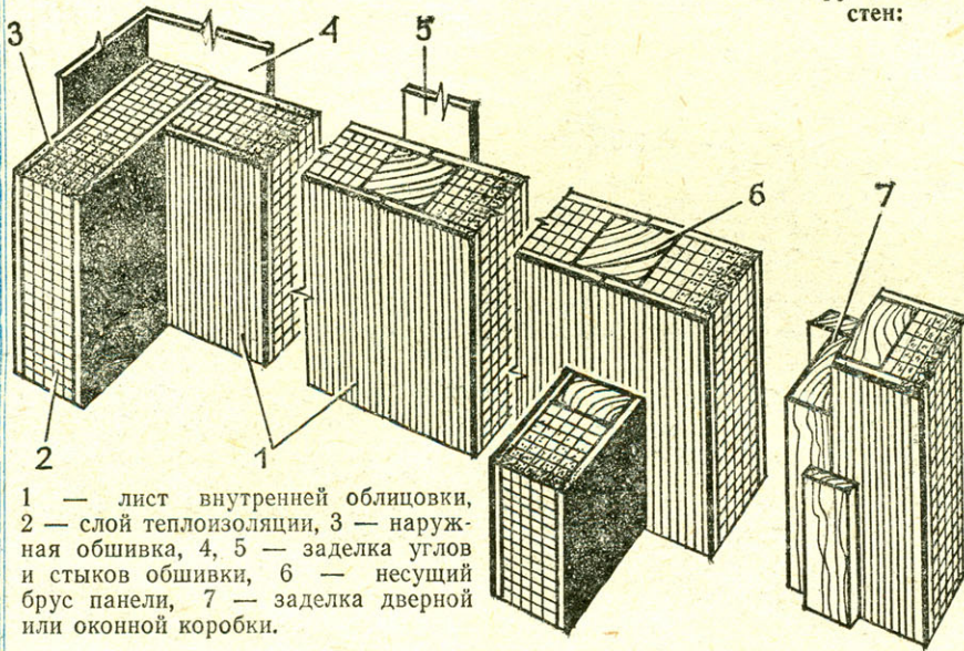
Рис. 3. Конструкция стен:
