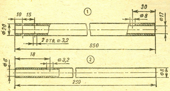
Рис. 5. Удлинительная штанга: 1 — для прибора, 2 — для игрового варианта.
