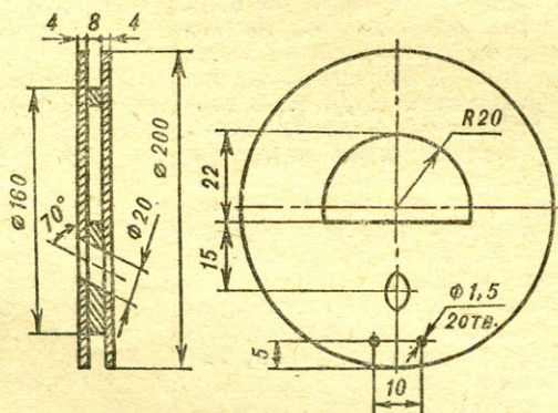
Рис. 4. Выносная головка игрового варианта прибора.
