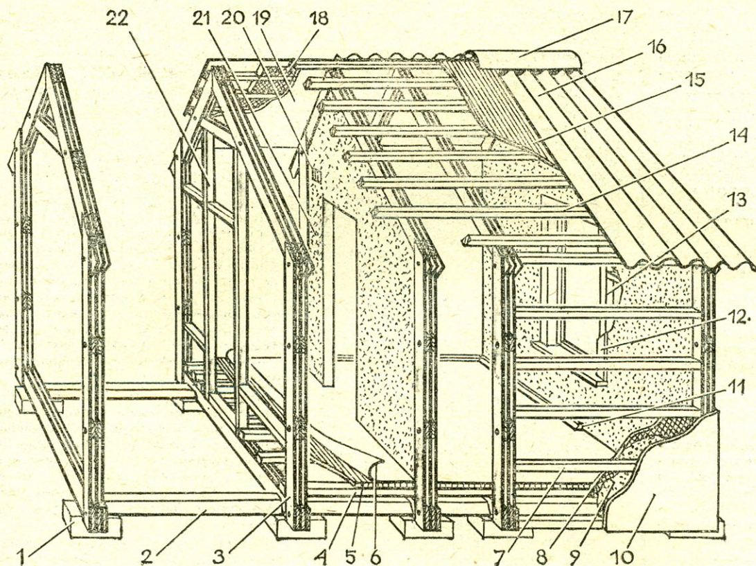
Рис. 1. Основные элементы конструкции домика-временки: 1 — фундамент, 2 — балка ростерка, 3 — рамы (несущий каркас), 4 — лаги, 5 — основание пола (доски, рейка), 6 — линолеум, 7 — обрешетка стен, 8 — лист внутренней облицовки (ДСП), 9 — теплоизоляция (шлак), 10 — лист ацеита (асбофанера), 11 — плинтус, 12 — наличник, 13 — оконная рама, 14 — обрешетка кровли, 15 — лист ДСП с гидрозащитной пропиткой, 16 — кровля (шифер), 17 — конек (жесть, шифер), 18 — утеплитель, 19 — фанера, 20 — вентиляционная решетка, 21 — перегородка, 22 — обрешетка перегородки.
