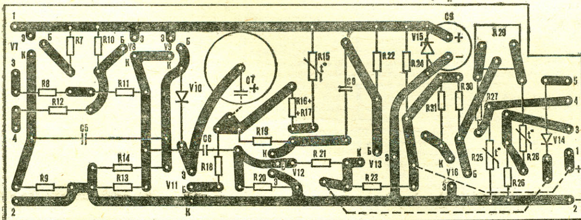
Рис. 2. Монтажная плата блока электронного опережения угла зажигания со схемой расположения деталей.
