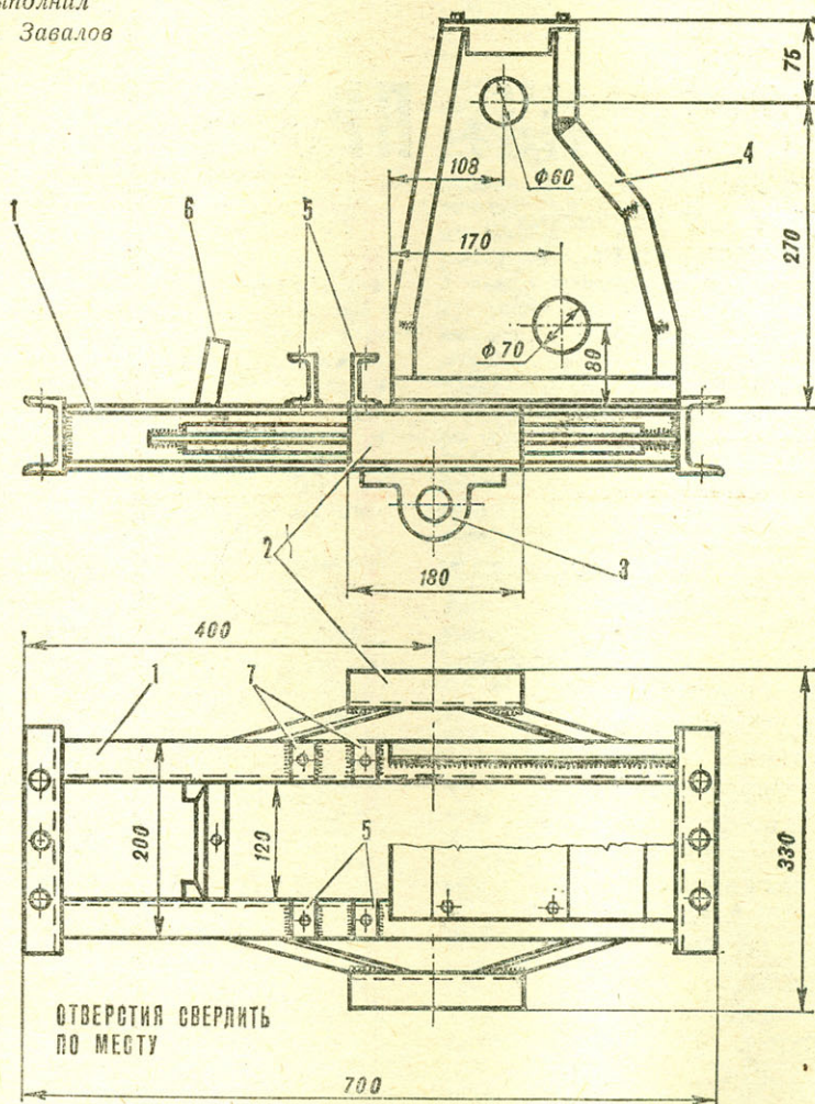
Рама мотоблока в сборе:
