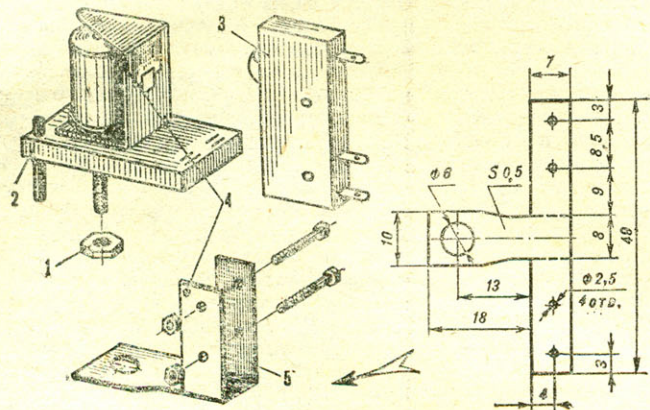
Переделка реле РСМ: 1 — гайка М3, 2 — реле РСМ, 3 — микропереключатель, 4 — места пайки проводов крепления, 5 — держатель.
