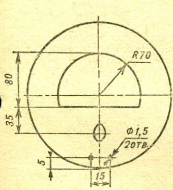
Рис. 3. Выносная головка для поиска на местности.
