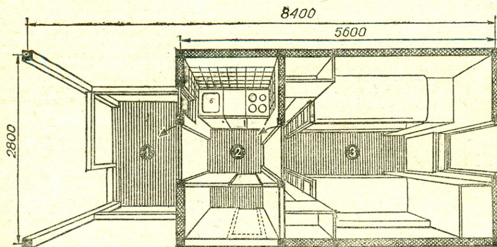
Рис. 2. План домика: 1 — веранда, 2 — кухня с кладовкой, 3 — спальня.
