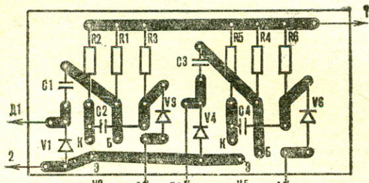
Рис. 1. Монтажная плата усилителей-формирователей со схемой расположения деталей.
