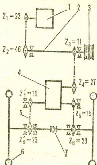
Кинематическая схема мотоблока: 1 — двигатель, 2 — промежуточный вал, 3 — двухручьевого шкив отбора мощности, 4 — дифференциал, 5 — конечная передача, 6 — колесо, 7 — механизм блокировки колес.
