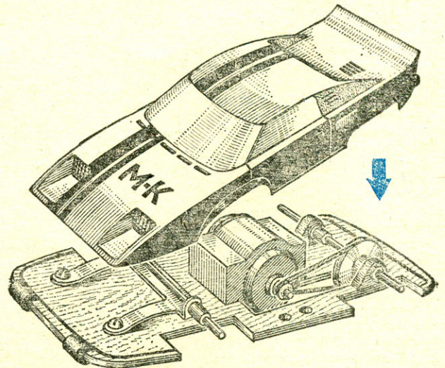
Автомодель класса ЭЛ-2 с электродвигателем МЭД и ременной передачей и ведущей оси. Подшипники ведущей оси — медные трубки, заклеенные в деревянных кронштейнах, передняя ось поддрессоренная. Полукопия спортивного автомобиля.
