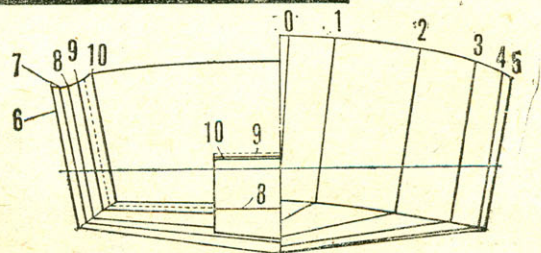
ВИД СЗАДИ
