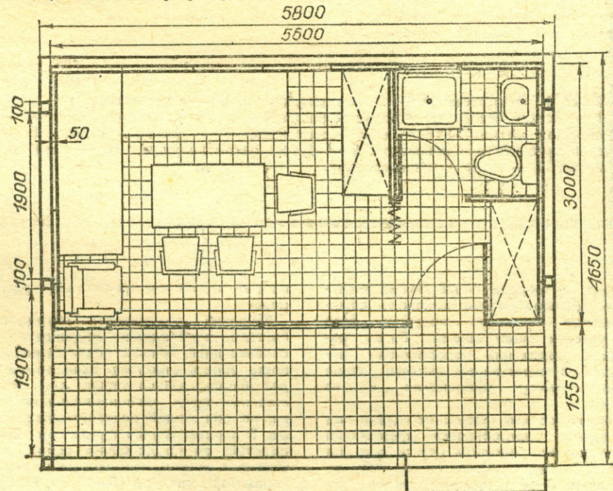
Рис. 2. План бунгало.
