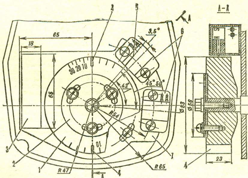
Рис. 3. Блок датчиков: 1 — измерительный диск, 2 — регулировочная шайба, 3 — усилители-формирователи, 4 — стальная пластина, 5 — метка отсчета угла опережения, 6 — датчики, 7 — основание.
