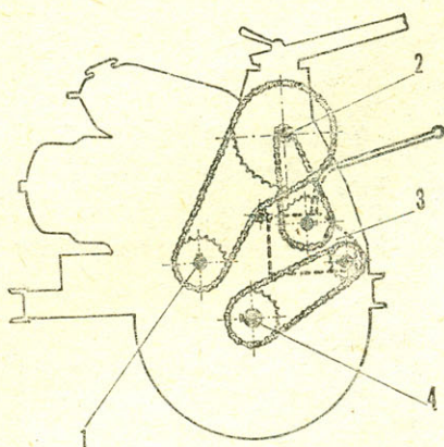
Компоновка трансмиссии: 1 — выходной вал двигателя, 2 — промежуточный вал, 3 — дифференциал, 4 — полуось колеса.
