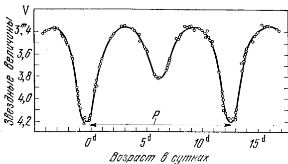
Рис. 5. Кривая изменения блеска \beta Лиры по фотоэлектрическим наблюдениям. Возраст наблюдений (время) дан в сутках. P — период переменности. Звездные величины — в V -лучах.
