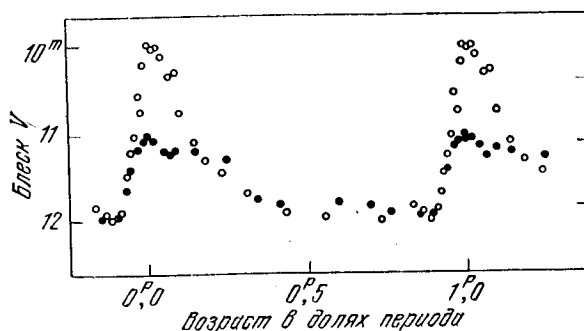
Рис. 23. Две предельные формы кривой блеска RZ Лыры как результат действия эффекта Блажко.
