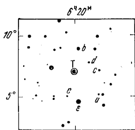
Т Единорога a = 5,81; b = 6,11; c = 6,41; d = 6,69; e = 7,28.
