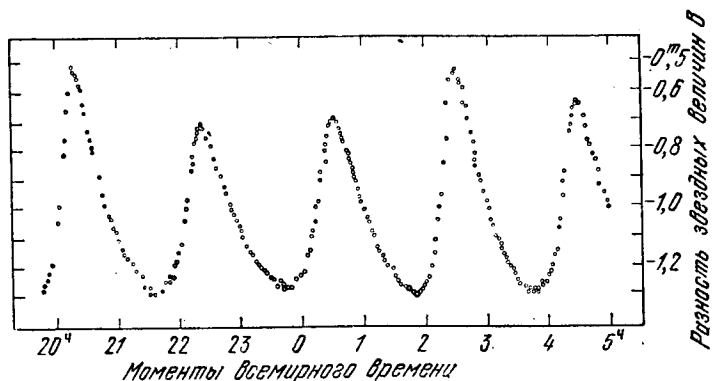
Рис. 24. Изменение блеска карликовой цефеиды АЕ Большой Медведицы на протяжении 9 часов одной ночи с 20 на 21 января 1974 г. На вертикальной оси отложены разности звездных величин переменной и звезды сравнения. Видно постепенное изменение кривой (эффект Блажко).
