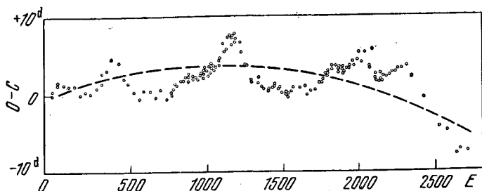
Рис. 19. График изменения O—C у цефеиды-дублье AP Геркулеса, характеризующий изменение ее периода. Периодические изменения сопровождаются вековым сокращением периода.
