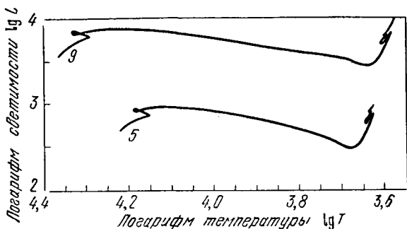
Рис. 3. Эволюционные треки звезд с малым содержанием тяжелых элементов в стадии образования гиганта.
