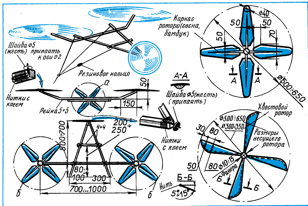
Рис. 27. Змей-вертушка Р. Фьюгэстона.
