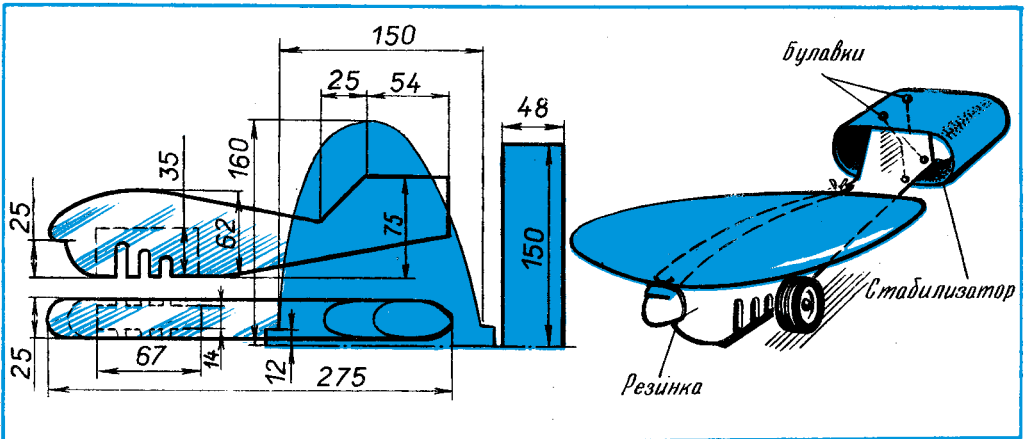
Рис. 98. Автомобиль-самолет.
