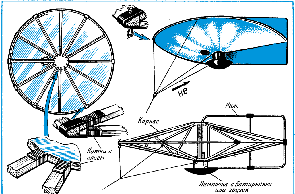
Рис. 22. Воздушный змей-диск.
