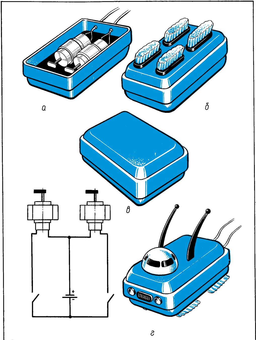
Рис. 104. Виброход из мыльницы.
