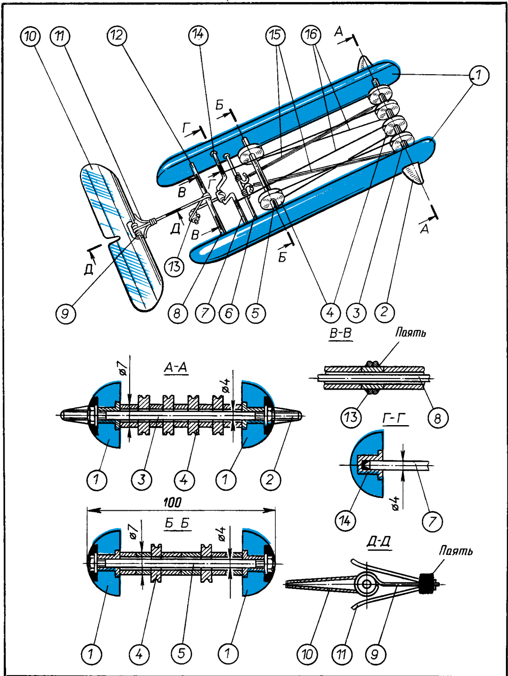
Рис. 135. Модель катамарана с плавниковым двигателем: 1 — поплавок корпуса модели; 2 — руль; 3 — передняя ось с четырьмя роликами полиспата; 4; 5 — промежуточная ось с двумя роликами полиспата; 6 — коленчатый вал; 8 — задняя ось; 9 — плавниковый стержень; 10 — плавник; 11 — упоры; 12 — втулка; 13 — шатун; 14 — подшипники; 15 — резиновые жгуты; 16 — гибкие тяги
