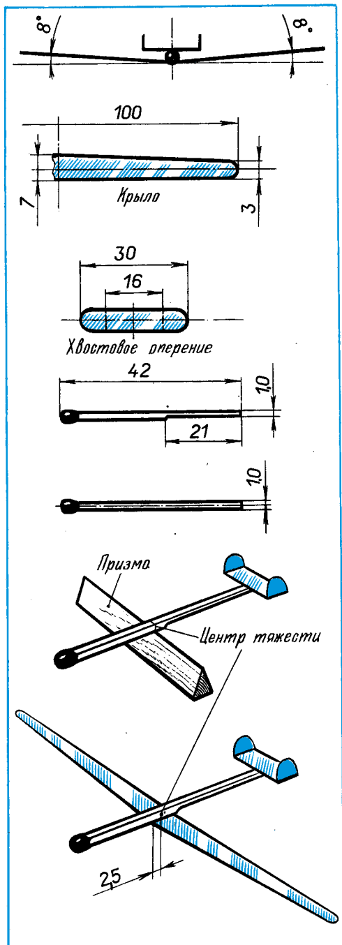
Рис. 39. Летающая спичка.
