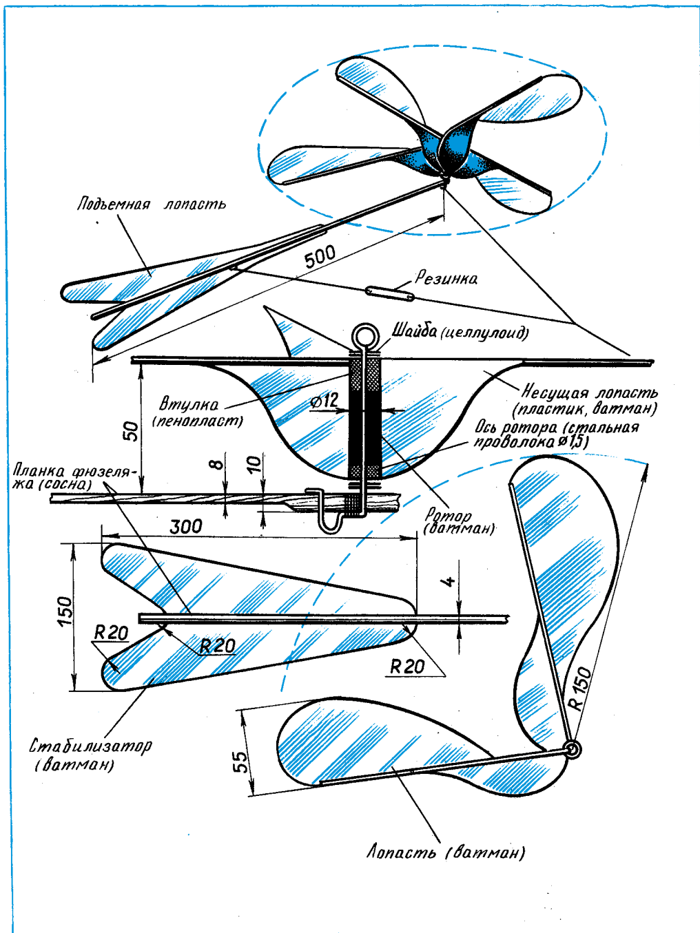
Рис. 30. Змей-автожир.
