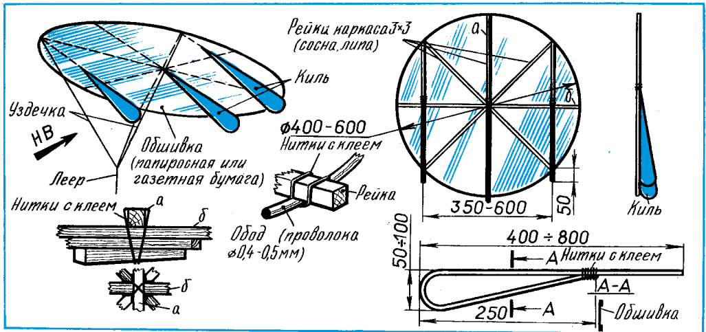
Рис. 23. Змей-дисколет.
