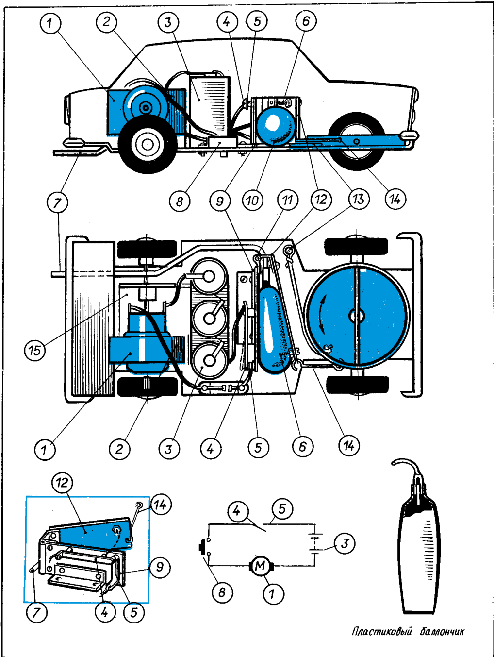
Рис. 111. Еще одна модель, управляемая сжатым воздухом.
