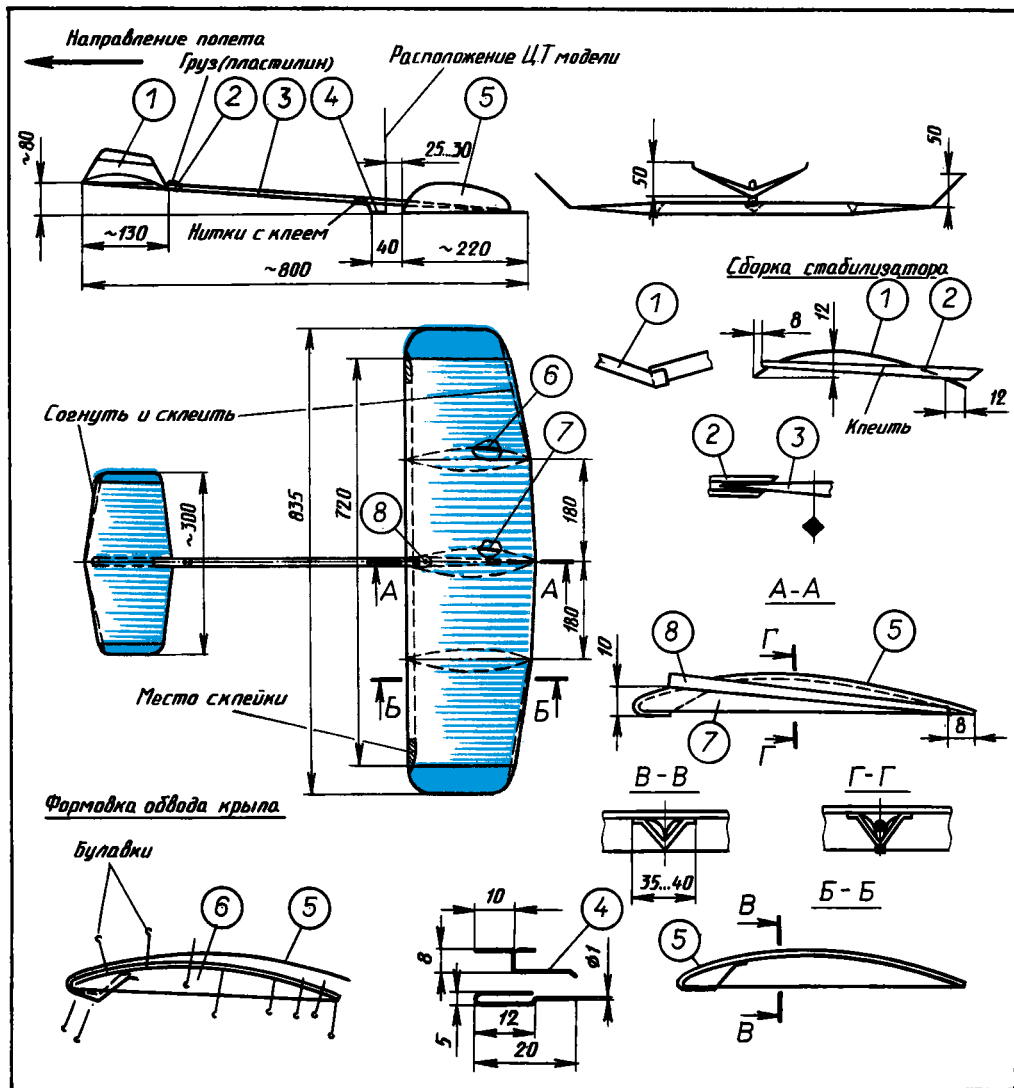
Рис. 69. Бумажный планер.
