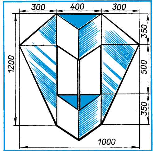
Рис. 17. Двукоробчатый змей И. Коница.
