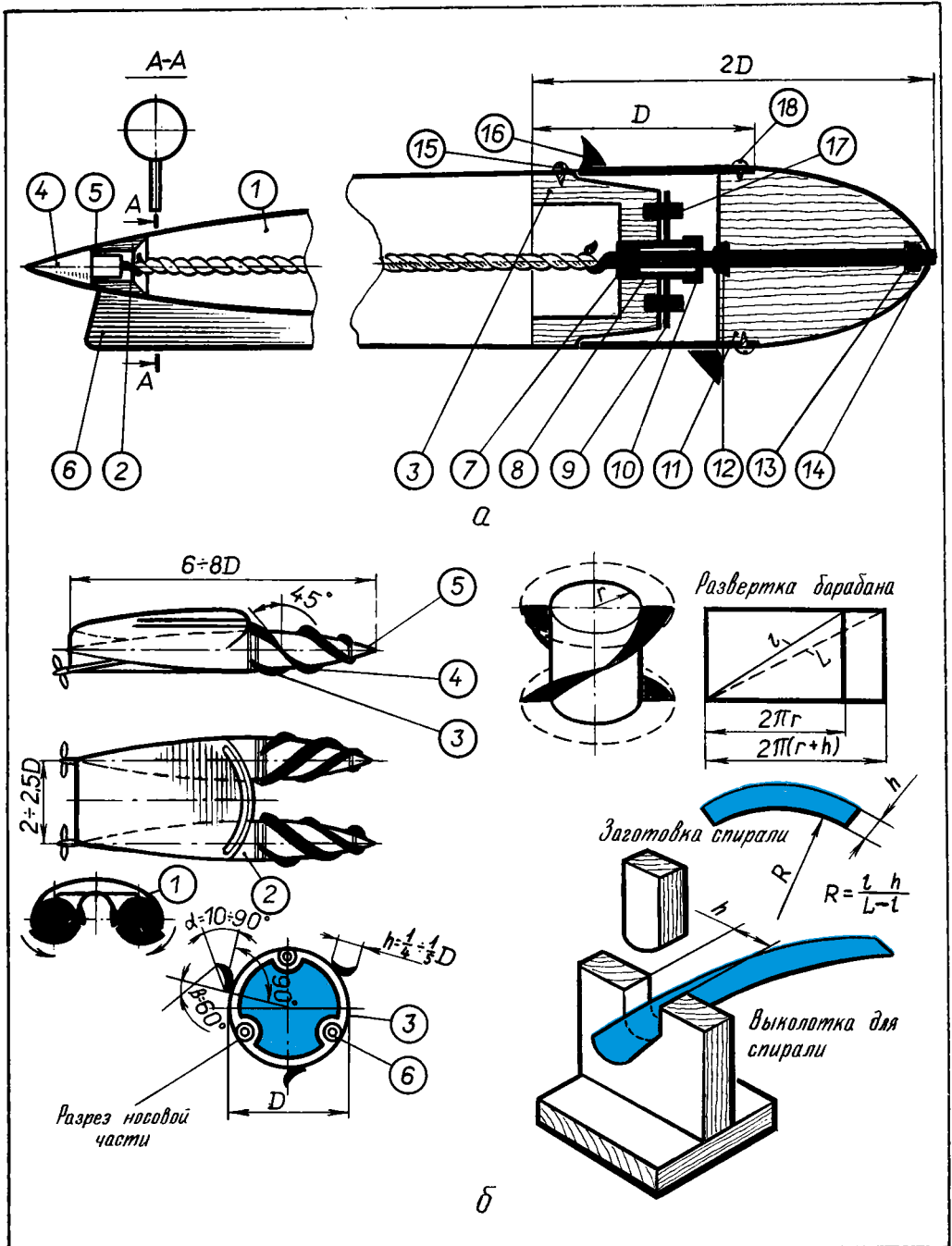
Рис. 130. Ротативное судно.
