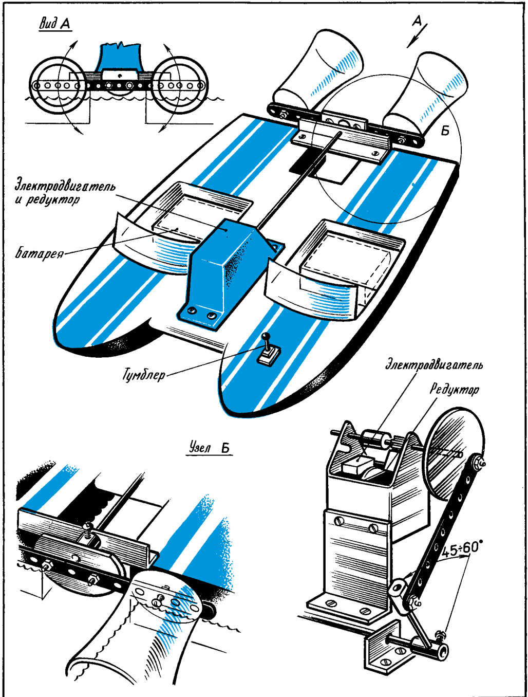
Рис. 132. Модель Р. Романова.
