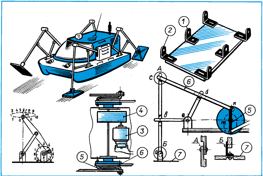
Рис. 101. Оленеход.
