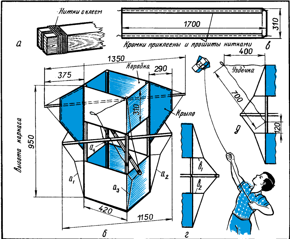
Рис. 18. Двукоробчатый змей Д. Лаврицева.
