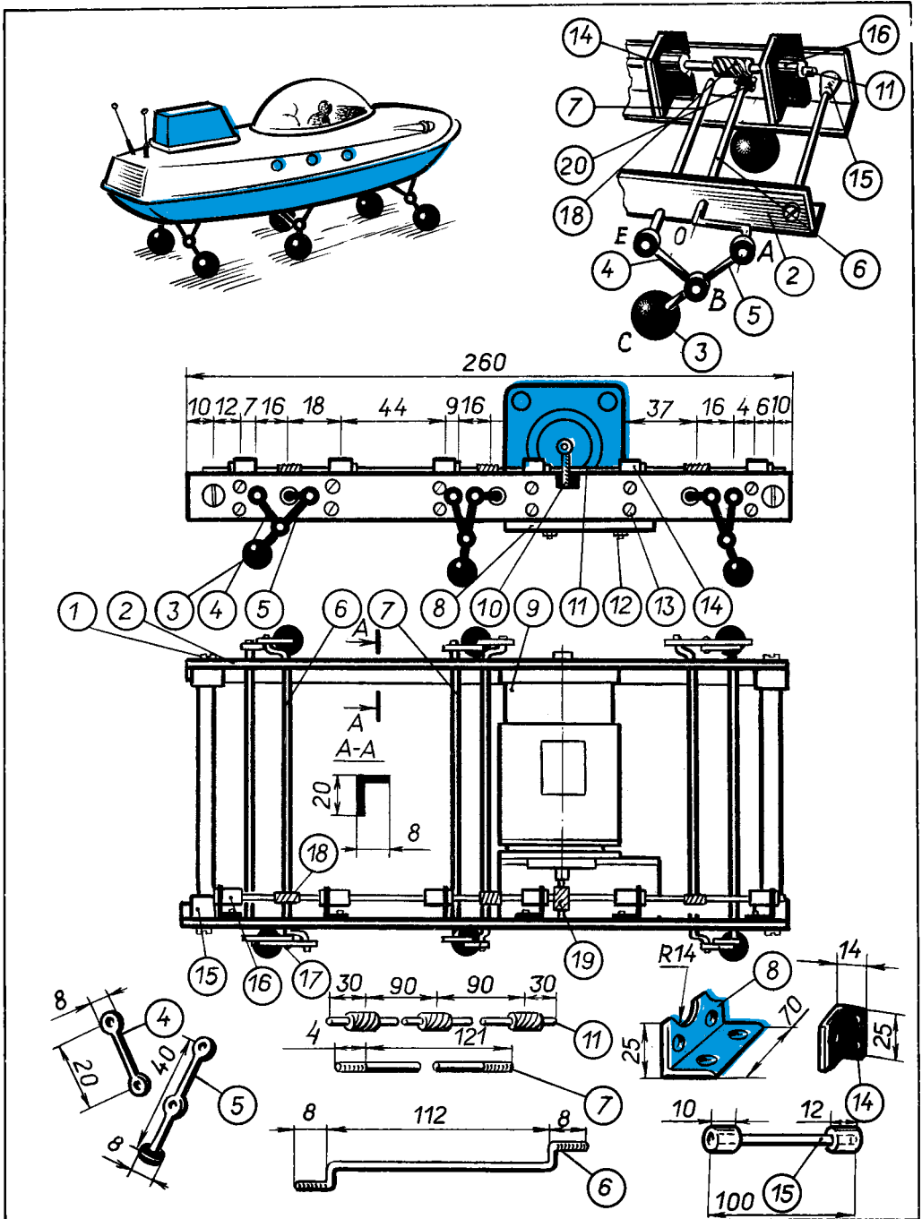
Рис. 100. Шагающая модель Г. Либерта.
