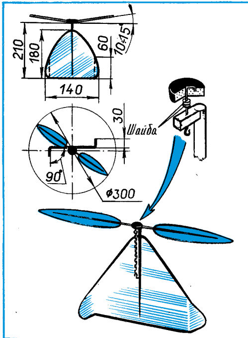
Рис. 74. Вертолет-бабочка.
