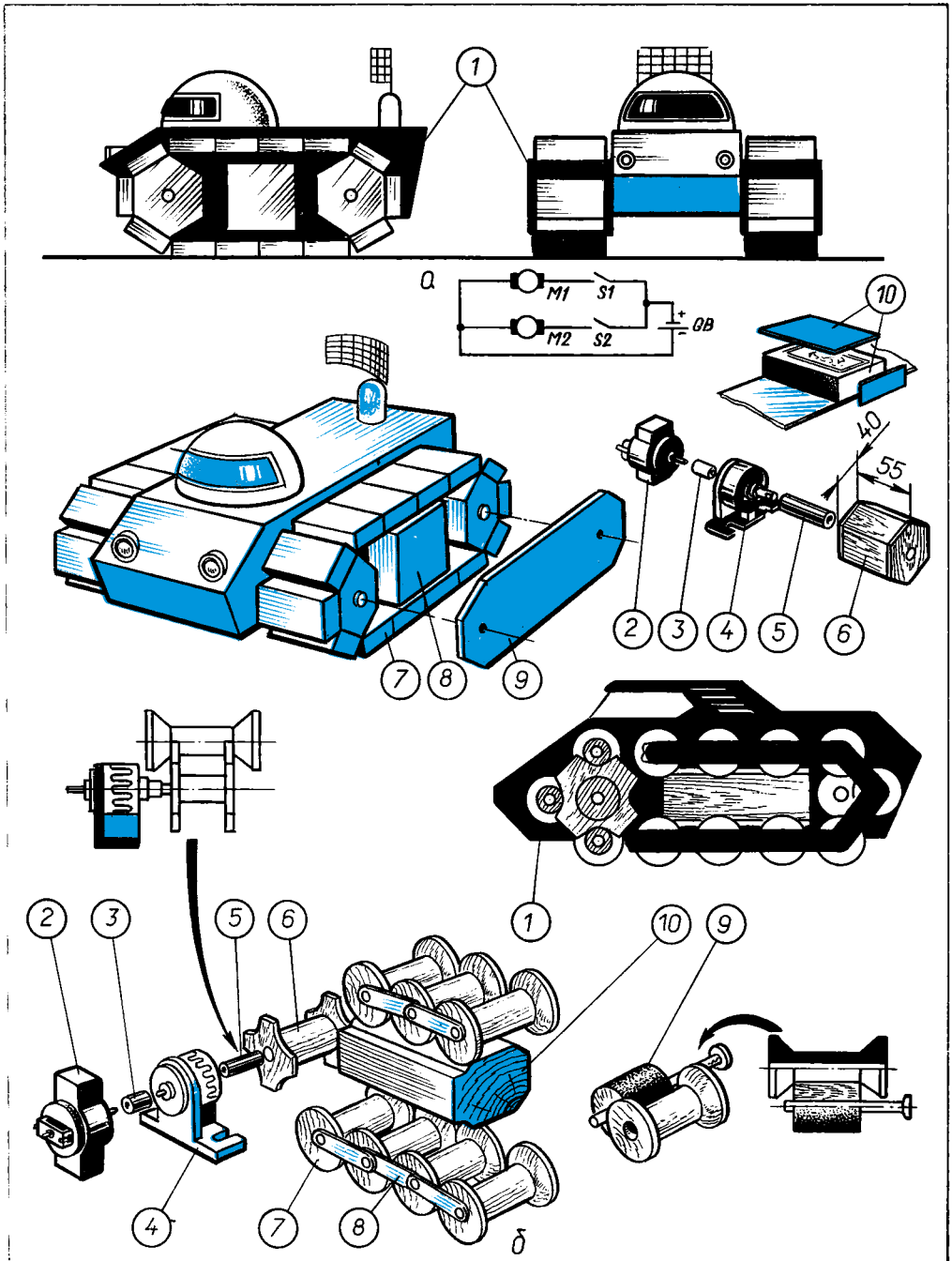
Рис. 115. Модели вездеходов В. Шпаковского.
