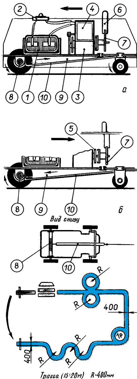
Рис. 114. Модель с механической «памятью».
