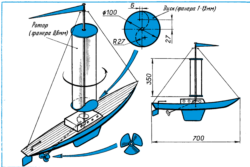
Рис. 122. Парус-двигатель.
