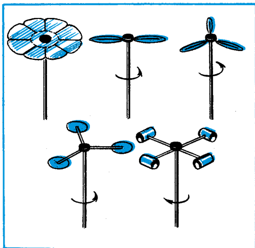
Рис. 72. Конструкции роторшютов.
