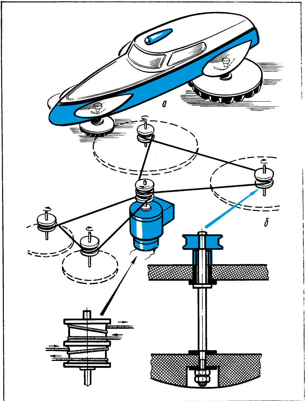
Рис. 117. Вездеход с тарельчатым двигателем.
