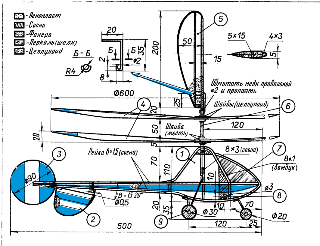
Рис. 29. Змей-вертолет А. Викторчика.
