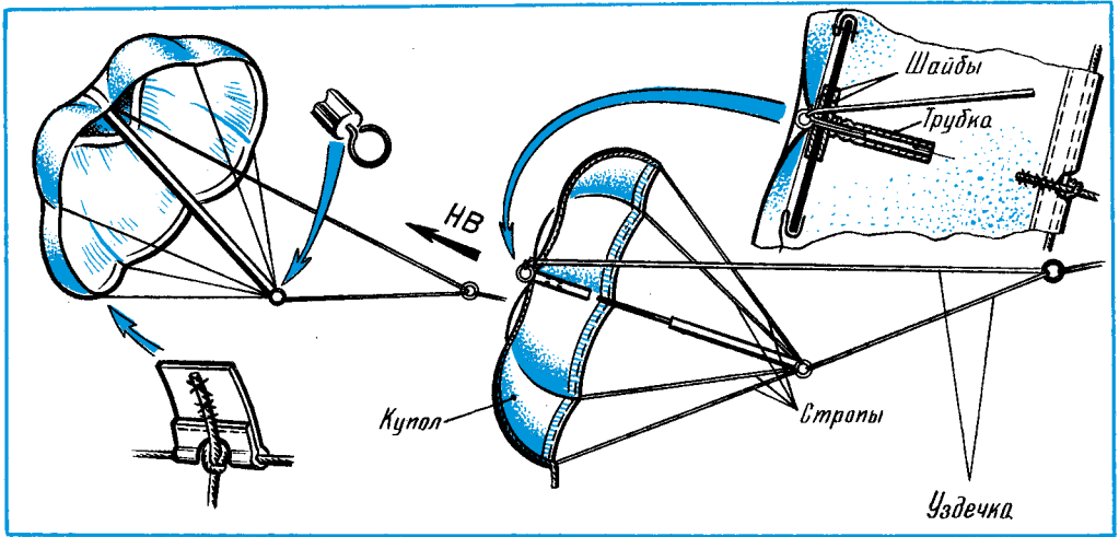
Рис. 21. Воздушный змей-парашют.
