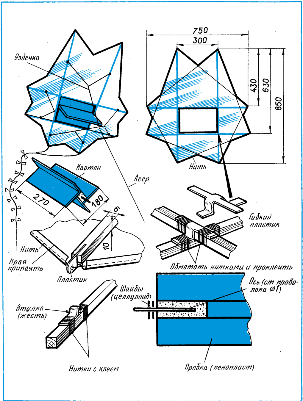
Рис. 28. Еще один змей-вертушка.
