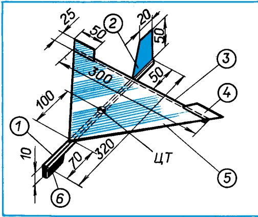
Рис. 63. Летящее крыло.
