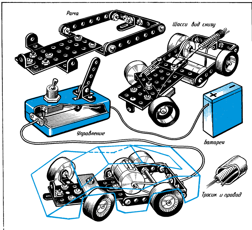
Рис. 103. Спортивный автомобиль.
