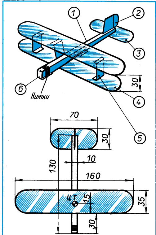
Рис. 66. Планер «биплан».
