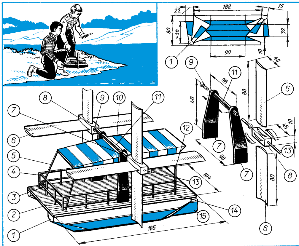
Рис. 126. Катамаран с прямоугольным парусом, вращающимся на оси.
