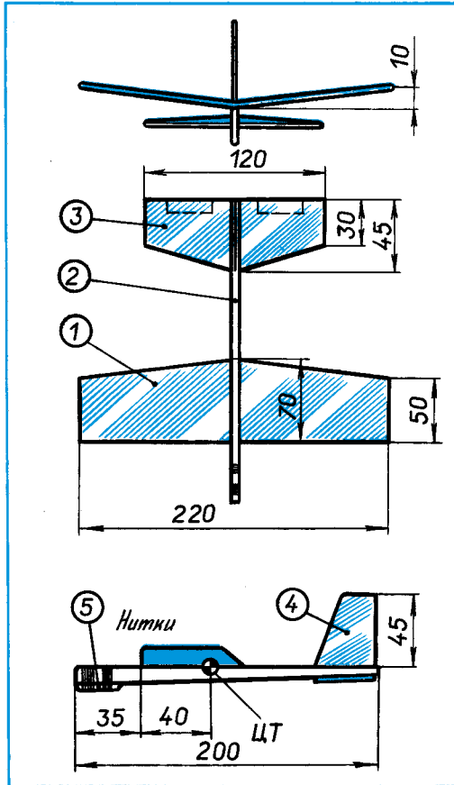
Рис. 64. Стриж.
