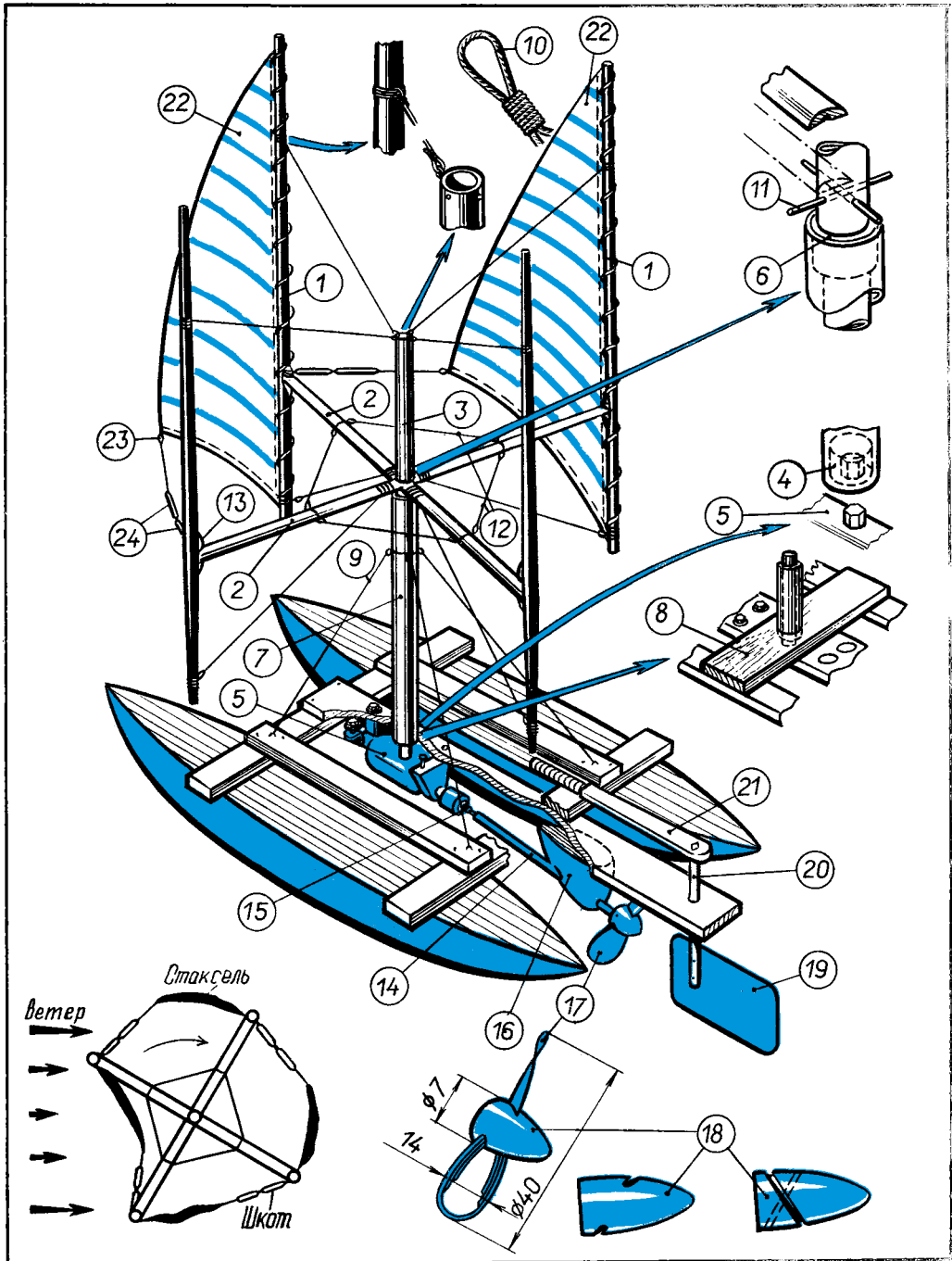
Рис. 131. Роторный катамаран.
