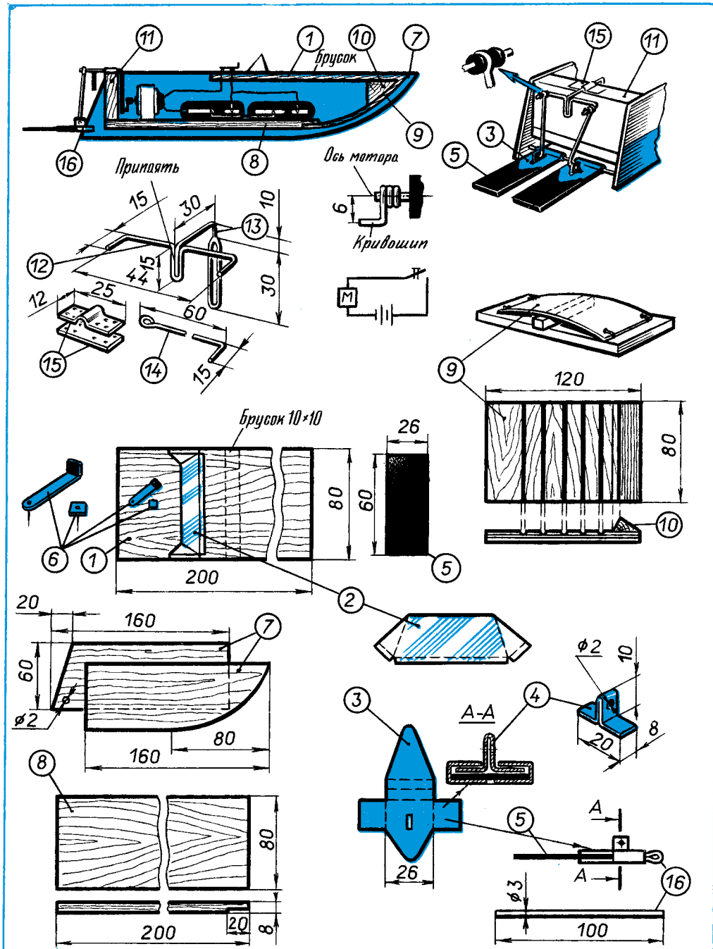
Рис. 123. Лодка с ластами.
