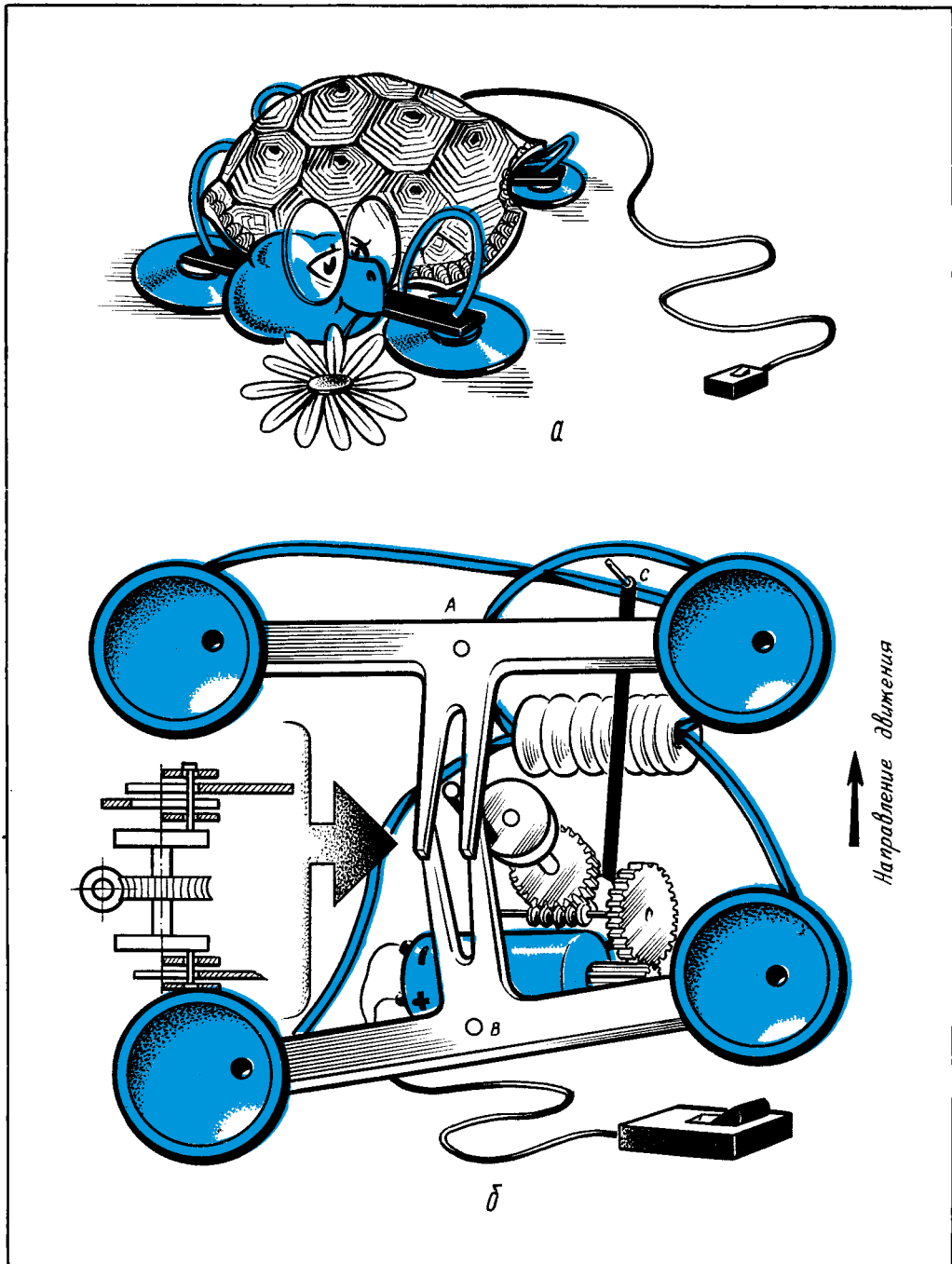
Рис. 102. Черепашкод.
