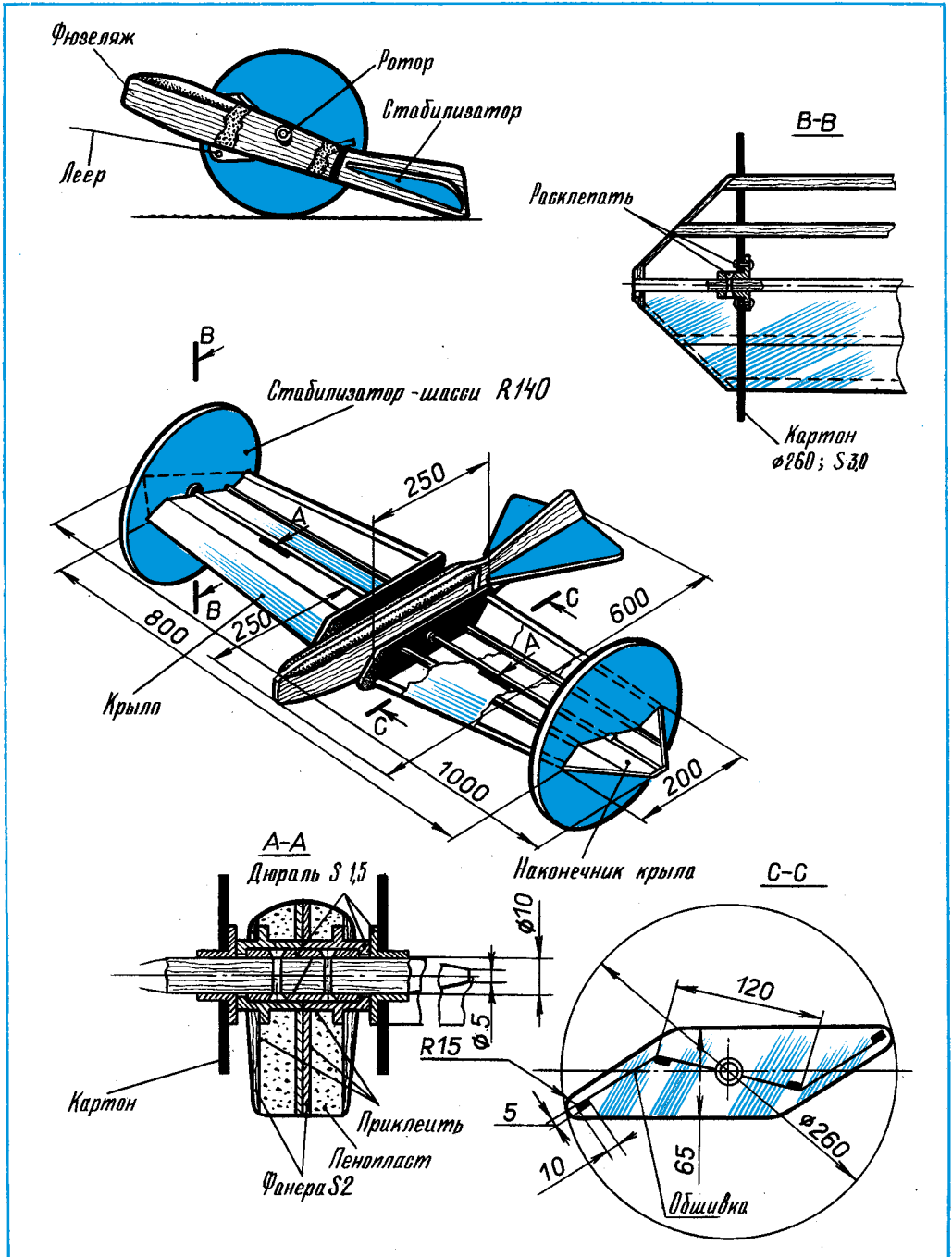
Рис. 33. Змей-самолет А. Финна.
