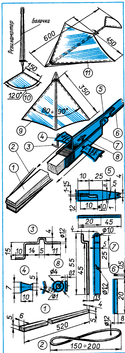
Рис. 95. Камбалолет.
