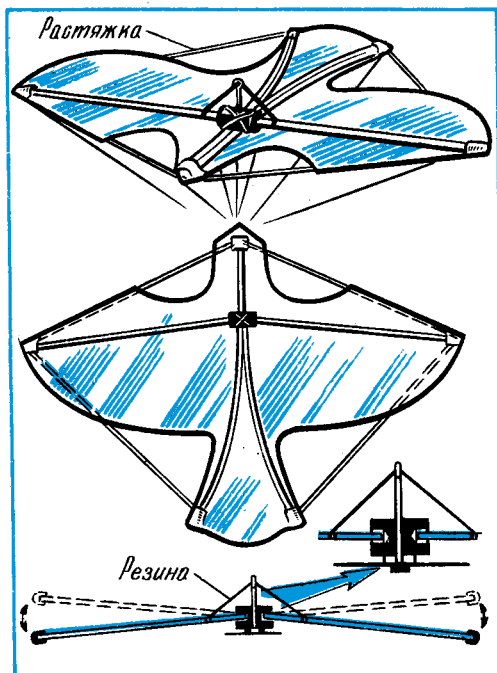
Рис. 13. Плоский воздушный змей-птица.
