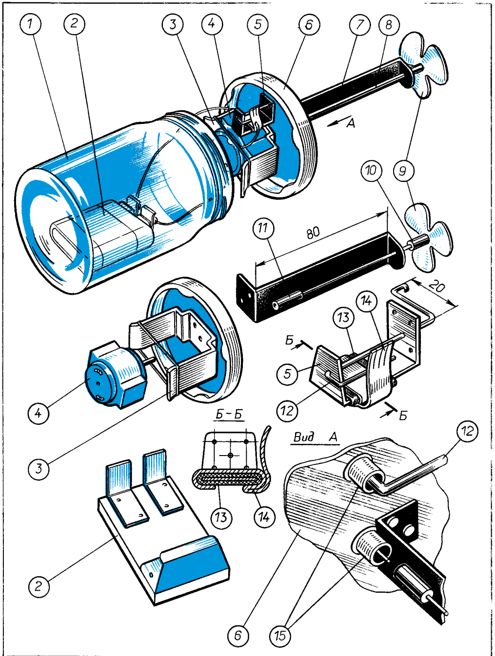
Рис. 137. Послушная торпеда.
