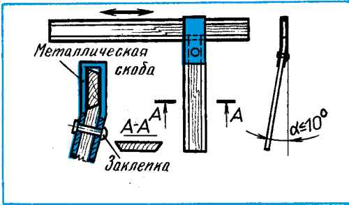
Рис. 88. Бумеранг Ч. Кливленда.
