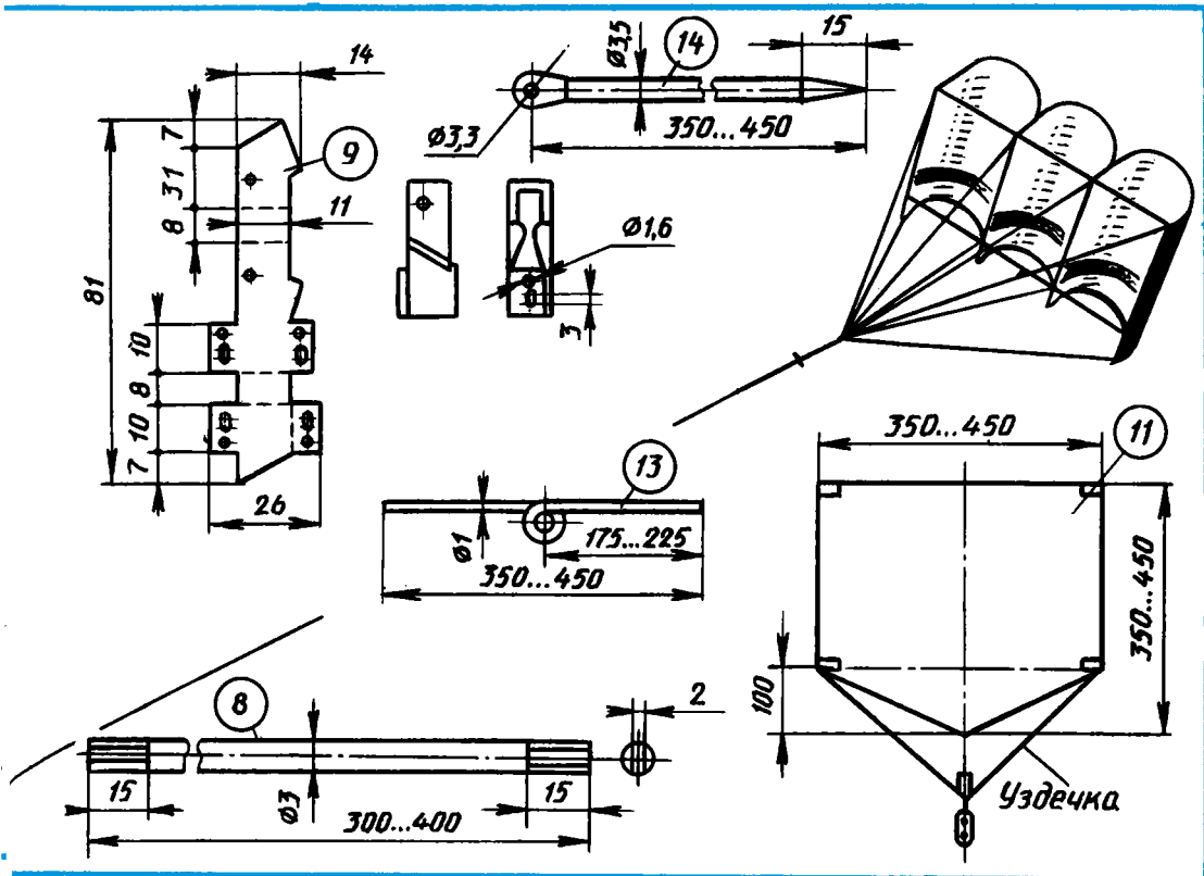
Рис. 35. Воздушный почтальон А. Заводного: 1— задняя тележка; 2— ось; 3— ролик; 4— пружинка; 5— обушок; 6— наконечник; 7— толкатель; 8— рама; 9— верхняя тележка; 10— планка; 11— парус; 12— верхний рей; 13— нижний рей; 14— мачта.
