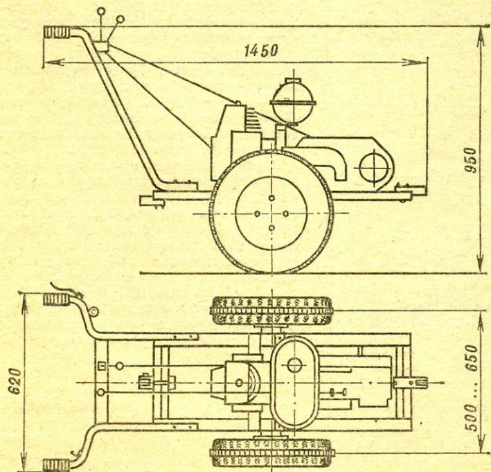
Рис. 1. Мотоблок «Сибиряк-3».
