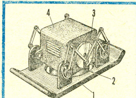
Рис. 1. Шагающий движитель: 1 — внешняя стопа-опора, 2 — внутренняя опора, 3 — кривошип, 4 — корпус.
