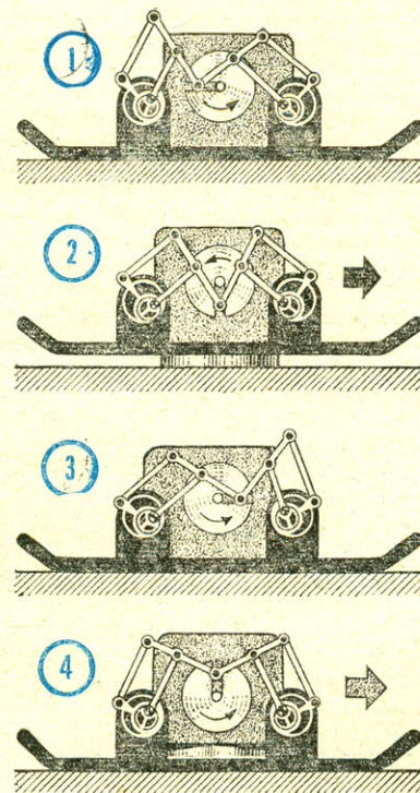
Рис. 2. Фазы работы кулачкового-рычажного механизма шагания: 1 — начало подъема внешней опоры, 2 — «зависание» на внутренней опоре при подаче внешней вперед, 3 — начало перемещения корпуса, 4 — движение корпуса вперед с опорой на внешнюю стопу.
