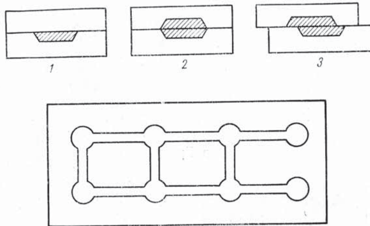
Рис. 5. Литейные формы
