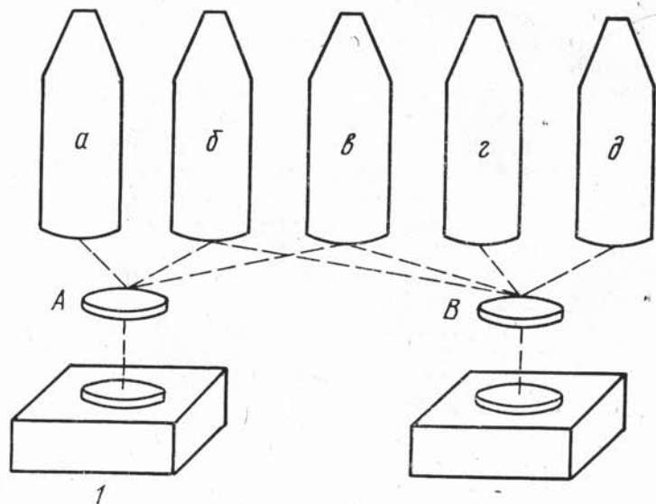
Рис. 2. Работа штемпелей
