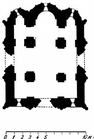
План церкви Покрова богородицы на Нерли. 1165 год.
