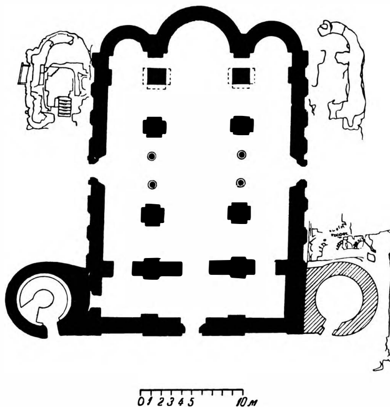
План Спасо-Преображенского собора в Чернигове. Около 1036 года.
