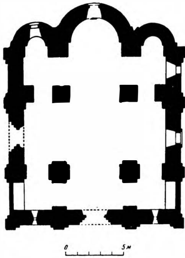
План церкви Бориса и Глеба в Кидекше. 1152 год.
