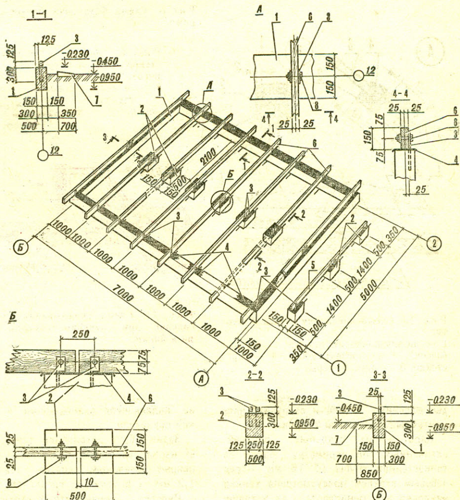
Рис. 1. Фундамент с несущими прогонами (разбивка и раскладка):
