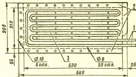
Нагреватель для воды: 1 — входной и выходной патрубки, 2 — отгибаемые части (линия загиба показана пунктиром), 3 — рабочая плоскость нагревателя.
