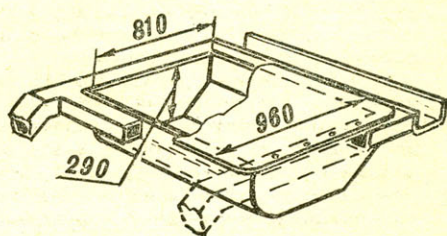
Рис. 8. Схема установки бензобака на раме.
