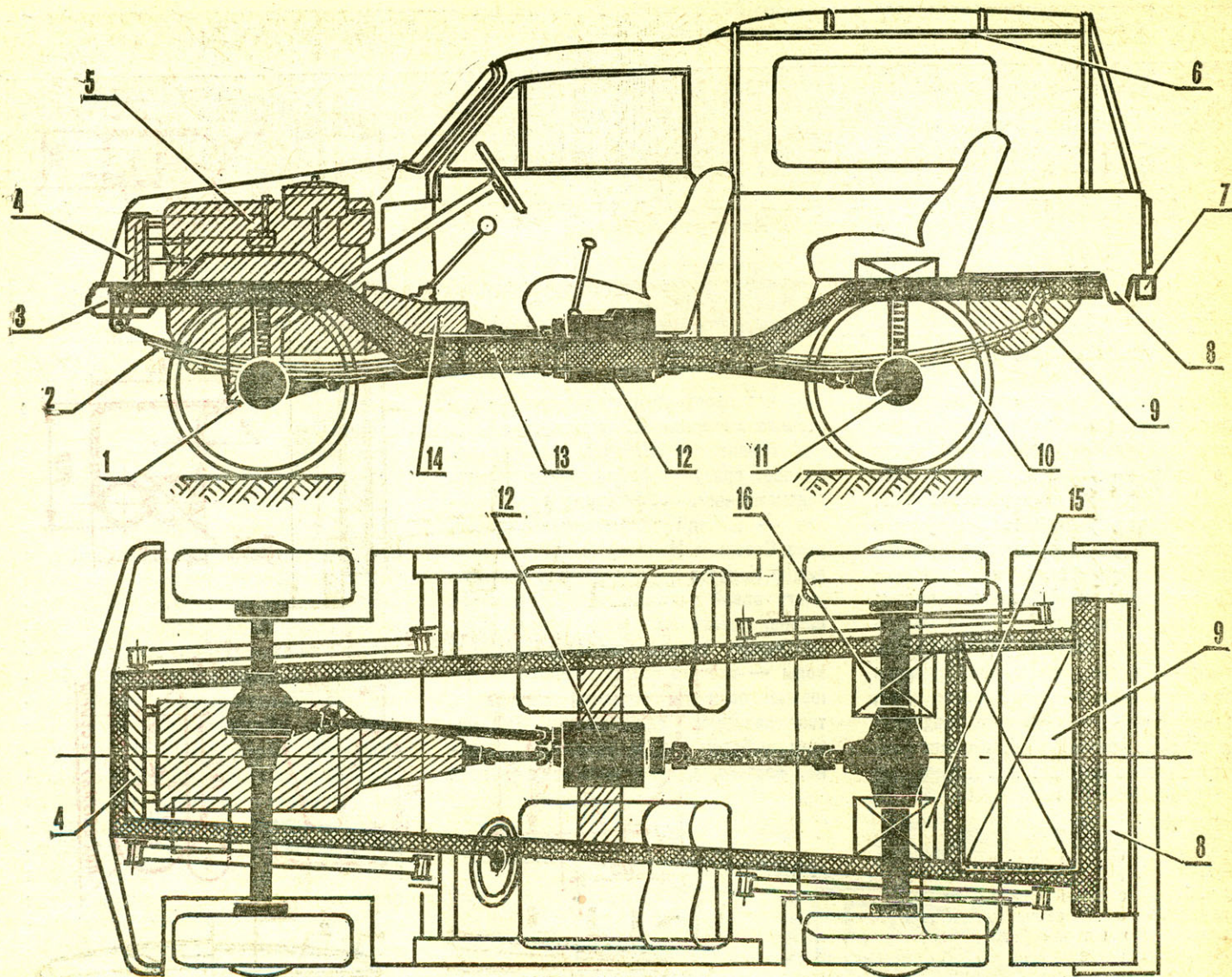
Р и с. 2. Компоновка автомобиля:
