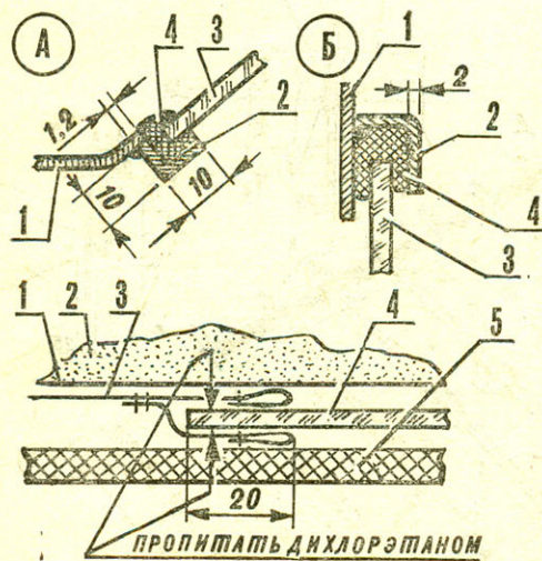
Рис. 10. Схема крепления стекла к тенту: 1 — полиэтиленовая пленка, 2 — груз (песок), 3 — брезент тента, 4 — оргстекло, 5 — лист фанеры.
