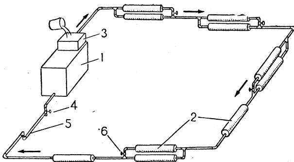
1 — Генератор тепла. 2 — Нагревательные приборы (гладкие трубы). 3 — Расширительный бак. 4 — Кран для спуска воды из системы. 5 — Проводка трубы под дверь. 6 — Запорно-регулирующий вентиль. Стрелка показывает уклон труб.
