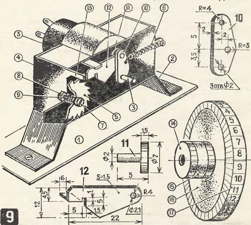
ДЕТАЛИ 10÷12 — ДЮРАЛЬ
