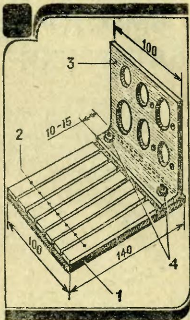
1 — плата, 2 — токопроводящие дорожки, 3 — пластина с набором стандартных отверстий, 4 — винты.
