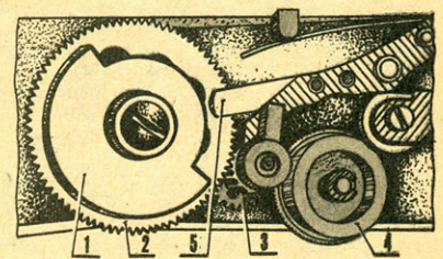
Р и с. 4. Редуктор перевода кадров:
