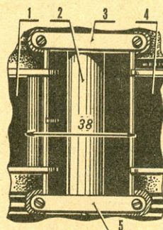
Р и с. 3. Внутренний узел стыковки «Смен-8М»:
