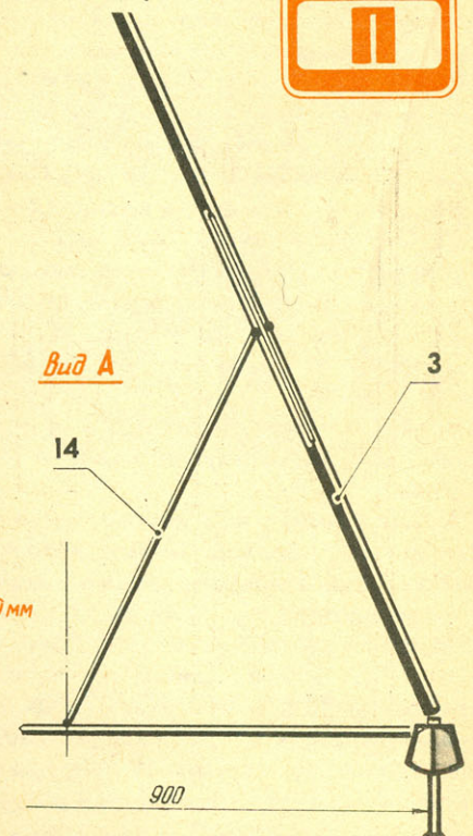
Р и с. 1. Парусная модель яхты класса «П»: 1 — стабилизатор, 2 — балка, 3 — крыло, 4 — ось вращения крыльевой системы, 5 — ось, используемая на курсе «фордевинд», 6 — киль, 7 — корпус, 8 — тяга автомата курса, 9 — трубка-подшипник баллера руля, 10 — руль, 11 — регулируемая транцевая плита, 12 — передняя поперечная балка, 13 — задняя поперечная балка, 14 — подкос (одинарный или Л-образный), 15 — носик-противовес.
