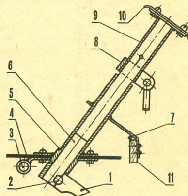
Схема рулевой колонки:
