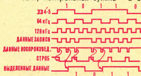
Принципиальная схема и временные диаграммы устройства сопряжения с дисководом.
