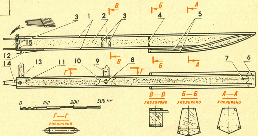
Рис. 6. Корпус (пенопластовый вариант):
