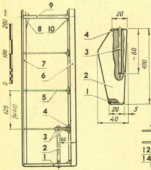
Рис. 4. Стабилизатор:
