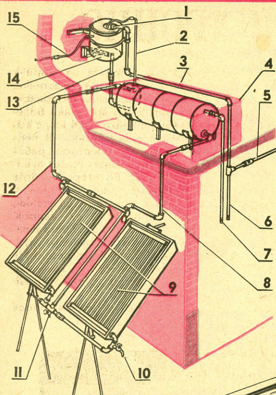
Рис. 1. Солнечный водонагреватель: 1 — поплавковый клапан аванкамеры, 2 — дренажная труба накопителя, 3 — трубопровод для подвода холодной воды к аванкамере, 4 — теплоизоляционный короб накопителя, 5 — труба ввода холодной воды, 6 — труба подвода холодной воды к смесителям; 7 — труба подвода горячей воды к смесителям, 8 — труба для подвода горячей воды к накопителю, 9 — солнечные коллекторы, 10 — сливной вентиль, 11 — вентиль для залива системы, 12 — «горячая» труба солнечного коллектора, 13 — труба подпитки накопителя, 14 — аванкамера, 15 — дренажная труба аванкамеры.
