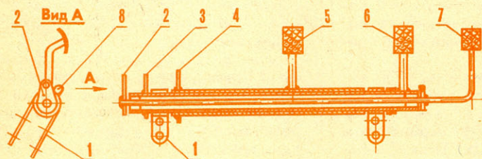
Схема педального вала:
