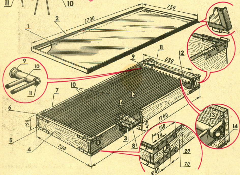
Рис. 3. Солнечный коллектор: 1 — защитное стекло, 2 — рама (стальной уголок), 3 — дно (оргалит толщиной 5 мм), 4, 7 — стенки корпуса коллектора (доска сечением 120×25 мм), 5 — стальная накладка (полоса сечением 2,5×20 мм), 6 — накладка-уголок, 8 — усиление днища (деревянный брус сечением 30×50 мм), 9 — соединительная муфта, 10 — трубка радиатора, 11 — приемная труба радиатора, 12 — хомут крепления радиатора, 13 — теплоотражатель (оцинкованное кровельное железо или белая жесь), 14 — теплоизолятор (пенопласт, стекло- или шлаковата).
