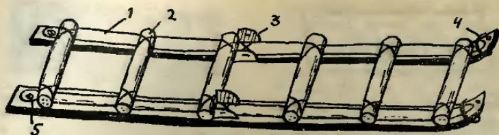
1 — лыжа, 2 — жердочка, 3 — лыжное крепление, 4 — аеревка, 5 — шуруп.
