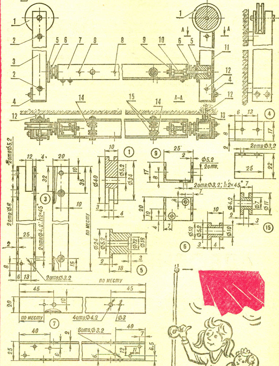
Рис. 2. Конструкция бельёвого «лифта» (левая часть):
