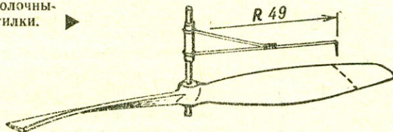
Изготовление кольцевой насадки воздушного винта:
