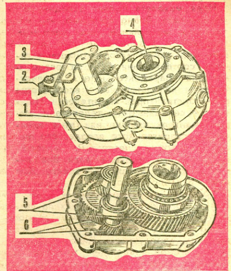
Редуктор с полым валом: 1 — корпус, 2 — тяга, 3 — быстроходный вал, 4 — тихоходный полый вал, 5, 6 — зубчатые пары с подшипниками.
