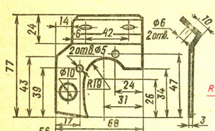
Р и с. 8. Накладка крепления на руле рычага муфты сцепления.
