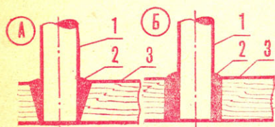
Рис. 2. Схема крепления направляющих трубок (А — первой, Б — второй): 1 — направляющая трубка, 2 — эпоксидный клей, 3 — основание.
