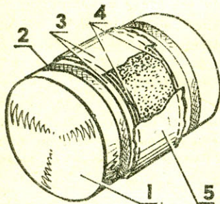
Изготовление кольцевой насадки воздушного винта:
