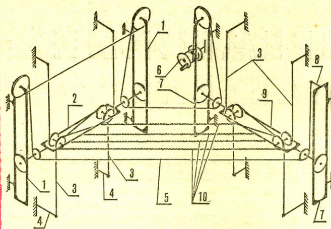
Рис. 1. Принципиальная схема проводки шнуров подъема и противовесной системы: 1 — направляющие левой части бельёвого «лифта», 2 — левая поперечина, 3 — шнуры противовесной системы, 4 — заделка шнура, 5 — шнур подъема, 6 — катушка подъема, 7 — направляющие правой части бельёвого «лифта», 8 — заделка шнура подъема, 9 — правая поперечина, 10 — бельевые веревки.
