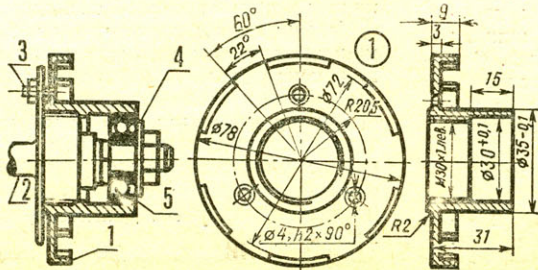
Рис. 3. Вариант крепления фланца — к стальной втулке — на резьбе:
