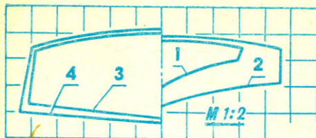
Проекция «корпус»
