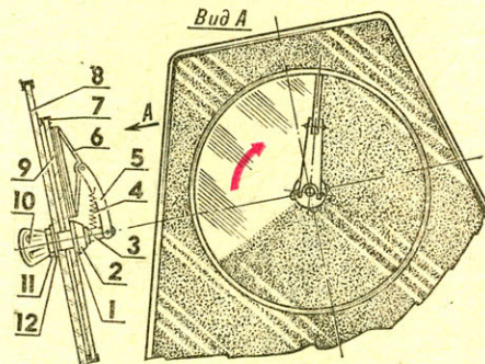
Устройство мотоциклетного стеклоочистителя: 1 — резиновая шайба, 2 — центральная втулка, 3 — ось, 4 — пружина, 5 — поводок, 6 — щетка, 7 — уплотнительное кольцо, 8 — лобовое стекло, 9 — диск из силикатного стекла, 10 — ручка привода стеклоочистителя, 11 — гайка, 12 — резиновая шайба.
