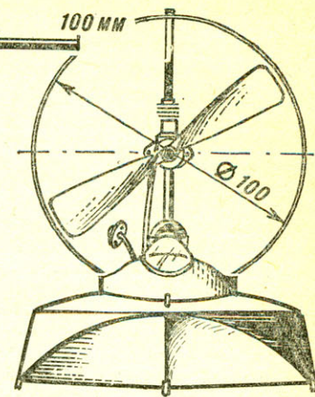
Модель глссера с воздушным винтом и двигателем на углекислом газе:
