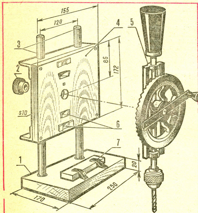
Рис. 1. Сверлильный станок:
