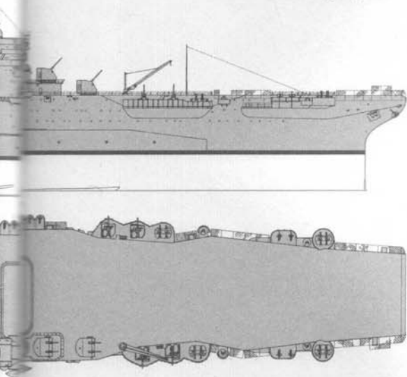
"Saratoga", 1944 г.
