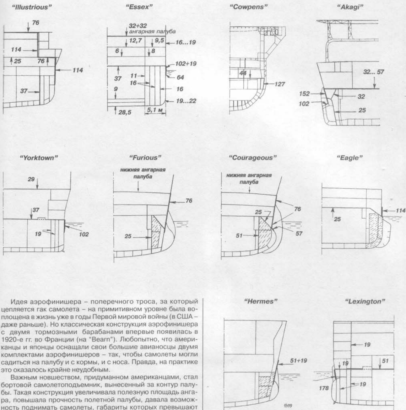
Поперечные сечения авианосцев (цифры означают толщину брони в мм)
