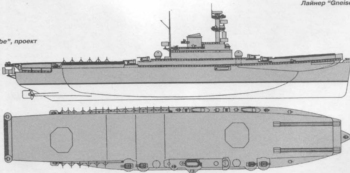
Лайнер "Gneisenau"
