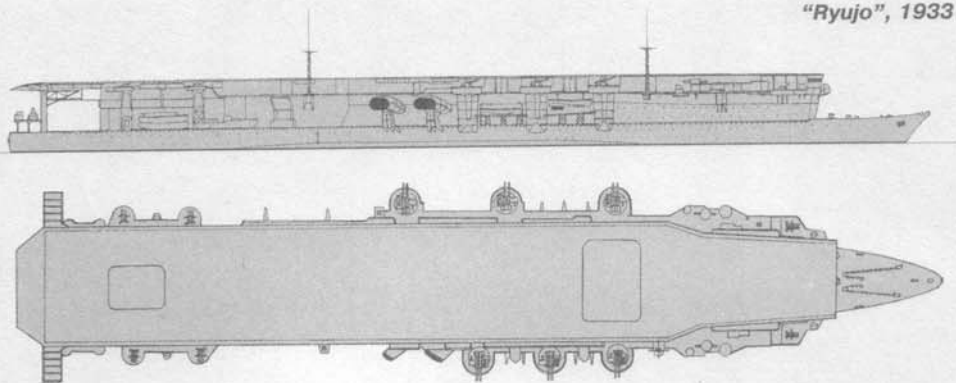
"Ryujo", 1933 г.
