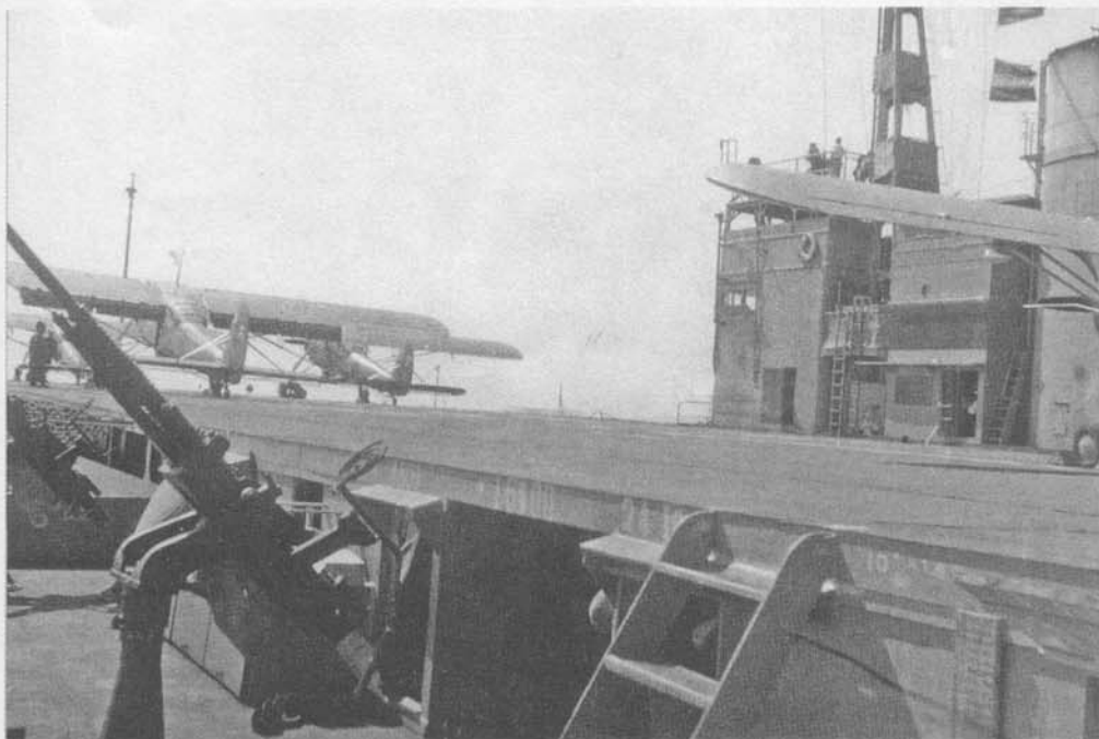
"Akitsu-Maru", 1944 г.
