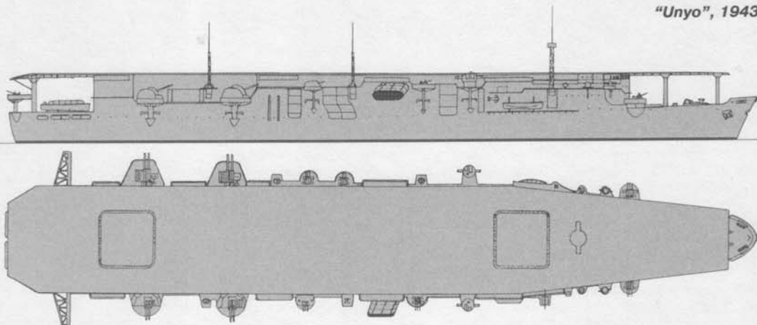
"Unyo", 1943 г.
