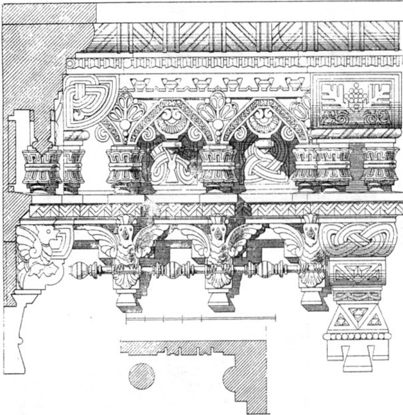
Деревянный карнизъ.
