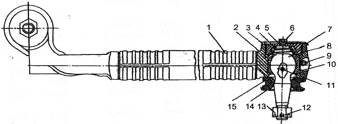
Рис. 67. Тяга продольная рулевая:
