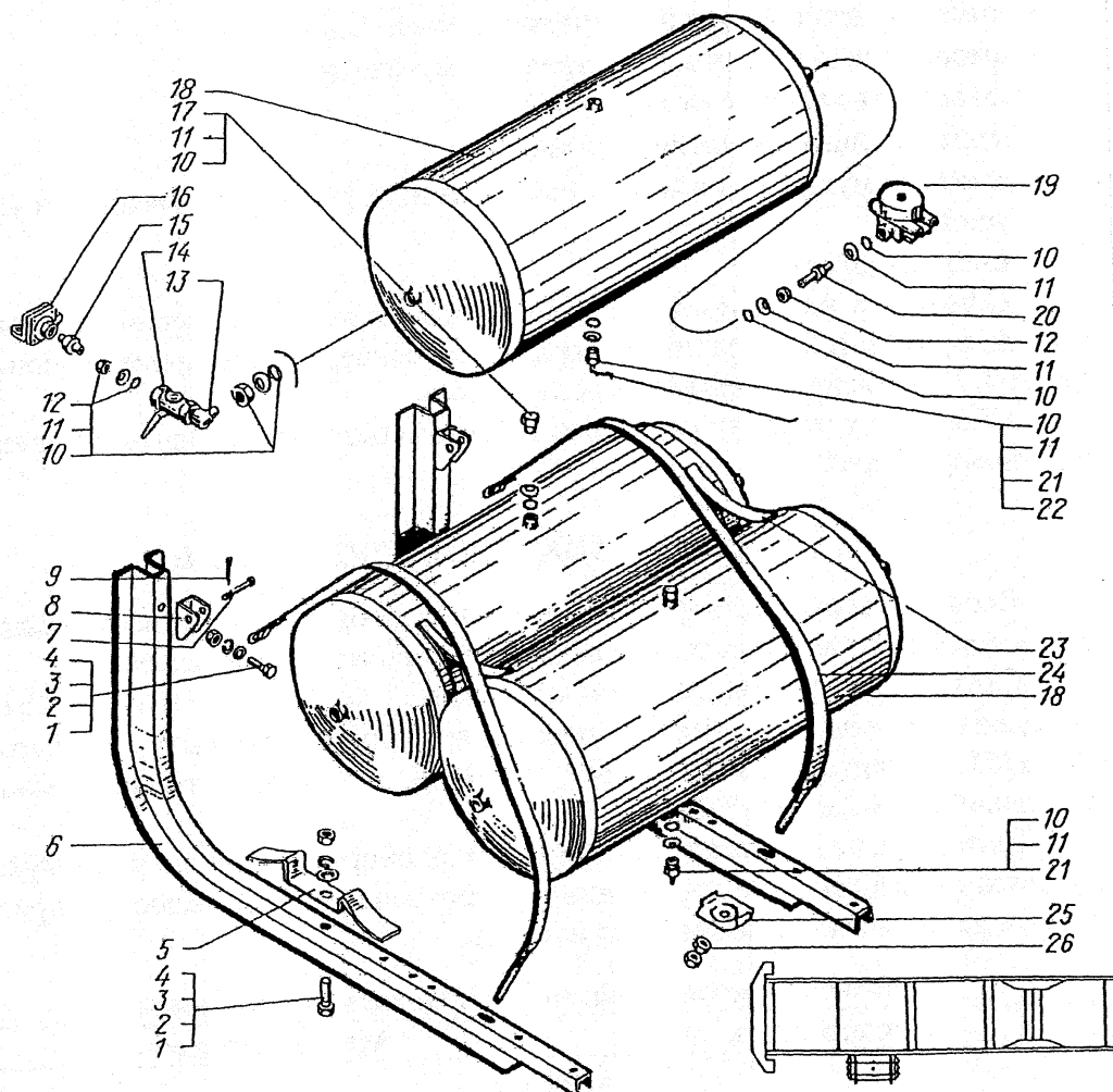
Рис. 92. Ресиверы:
