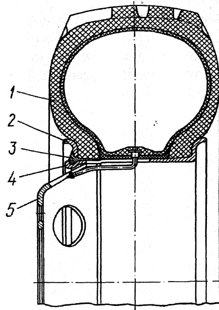
Рис. 51. Дисковое колесо:
