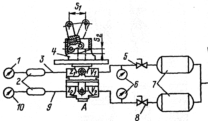
Рис. 86. Схема испытания тормозного крана: 1, 6, 10 - манометры; 2, 7 - ресиверы; 3 - первый контур; 4 - тормозной кран; 5, 8 - запорные краны; 9 - второй контур; S1 - ход рычага; S2 - ход толкателя
