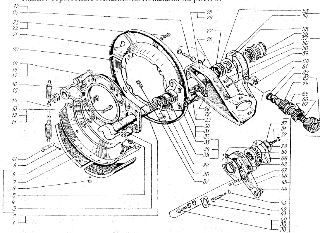
Рис. 90. Механизмы тормозные задних колес:
