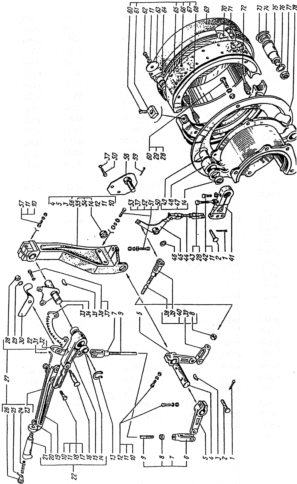
Рис.91. Управление стояночной тормозной системой
