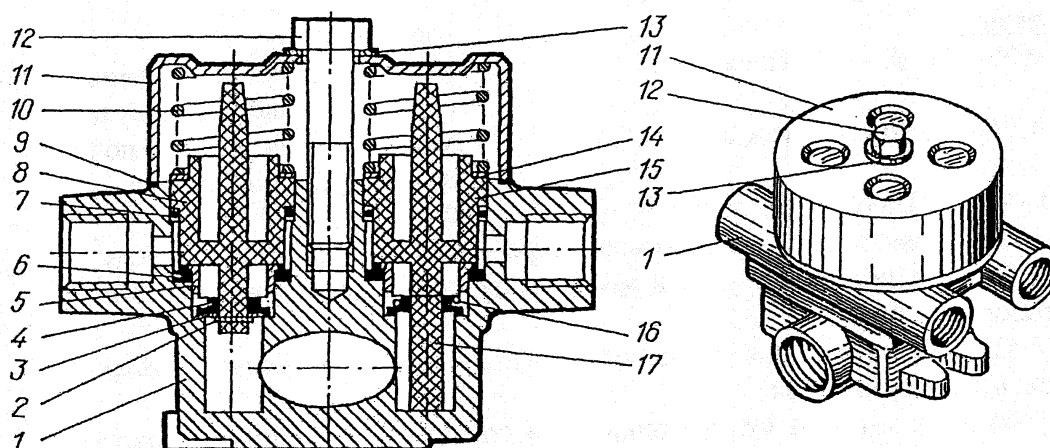
Рис. 88. Клапан защитный четырехконтурный:
