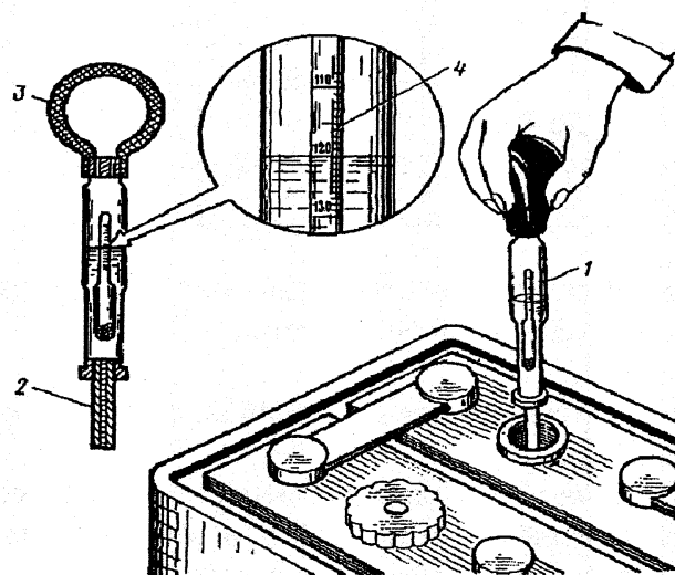
Рис. 97. Замер плотности электролита ареометром: 1 - корпус ареометра; 2 - трубка; 3 - резиновая груша; 4 - шкала ареометра
