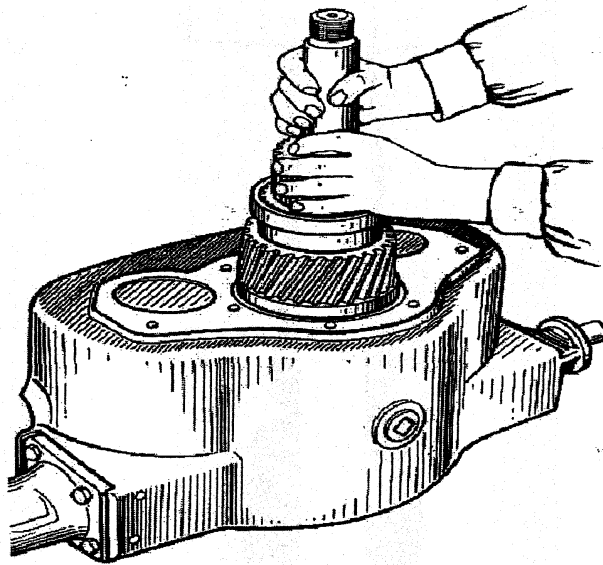
Рис. 24. Установка промежуточного вала в задний картер
