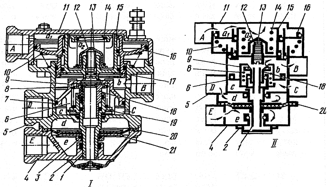
Рис. 77. Клапан управления тормозами прицепа с двухпроводным приводом: 1 - нижний поршень; 2 - выпускное отверстие; 3 - гайка; 4 - нижний корпус; 5 - средний корпус; 6 - средний поршень; 7 - уплотнительное кольцо; 8 - пружина клапана; 9 - тарелка пружины; 10 - пружина верхнего большого поршня; 11 - верхний корпус; 12 - тарелка пружины; 13 - регулировочный винт; 14 - пружина верхнего малого поршня; 15 - верхний малый поршень; 16 - верхний большой поршень; 17 - упорное кольцо; 18 - клапан; 19 - упорное кольцо; 20 - диафрагма; 21 - шайба диафрагмы
