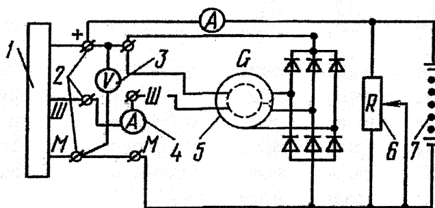
Рис. 99. Схема для проверки уровня настройки регулятора напряжения: 1 - регулятор напряжения; 2 - выводы; 3 - вольтметр; 4 - амперметр; 5 - генератор; 6 - реостат; 7 - аккумуляторная батарея; "Ш" и "М" - клеммовые выводы
