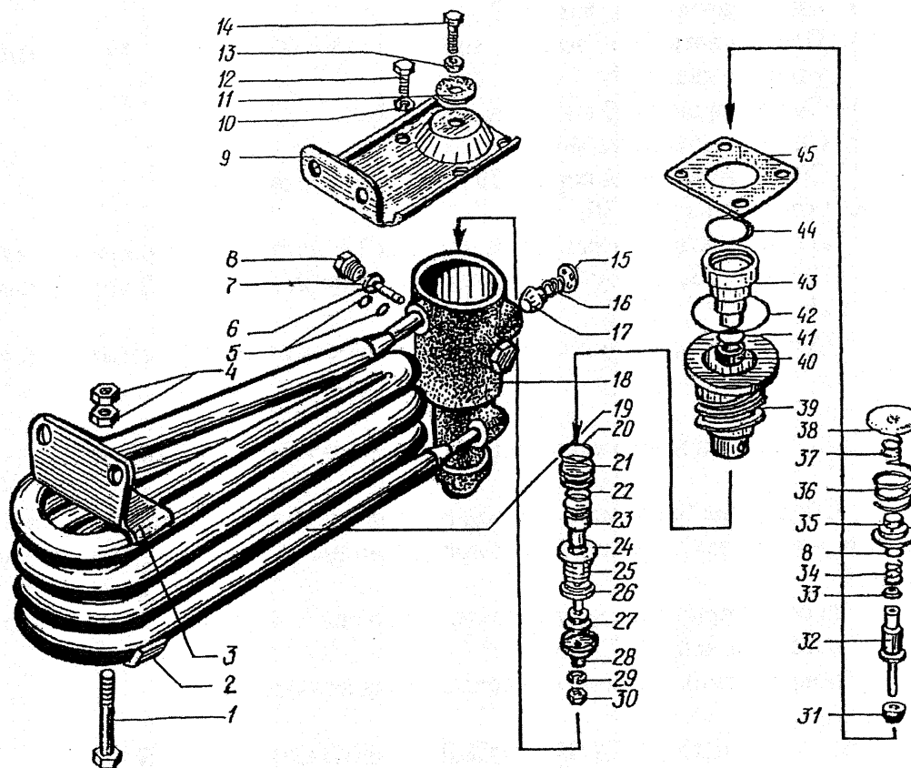
Рис. 83. Влагомаслоотделитель:
