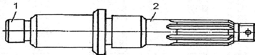
Рис. 19. Расположение шеек вала привода заднего моста: 1 - шейка под передний подшипник; 2 - шейка под задний подшипник
