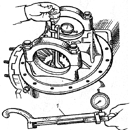
Рис. 36. Проверка затяжки подшипников динамометрической рукояткой: 1 - динамометрическая рукоятка
