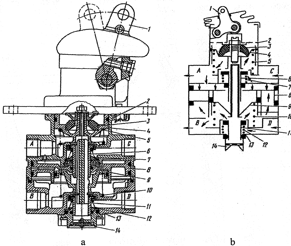
Рис. 73. Двухсекционный тормозной кран:
