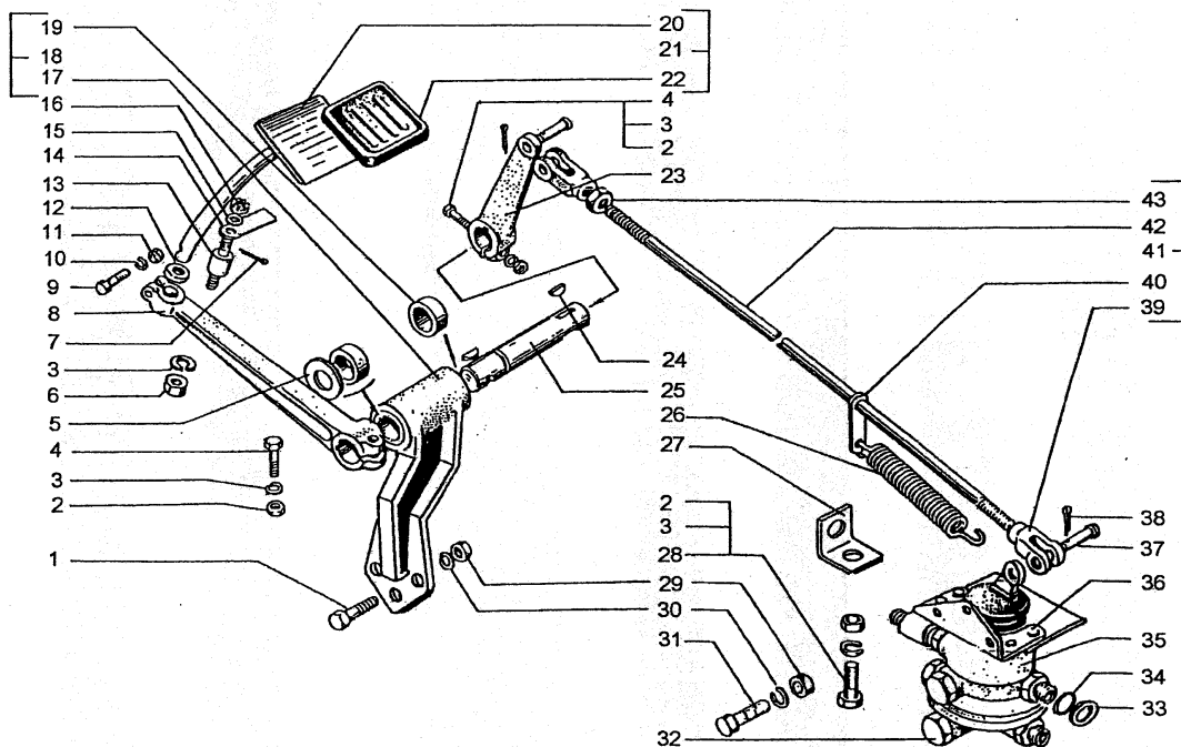
Рис. 72. Педаль тормозная и привод управления двухсекционным тормозным краном:
