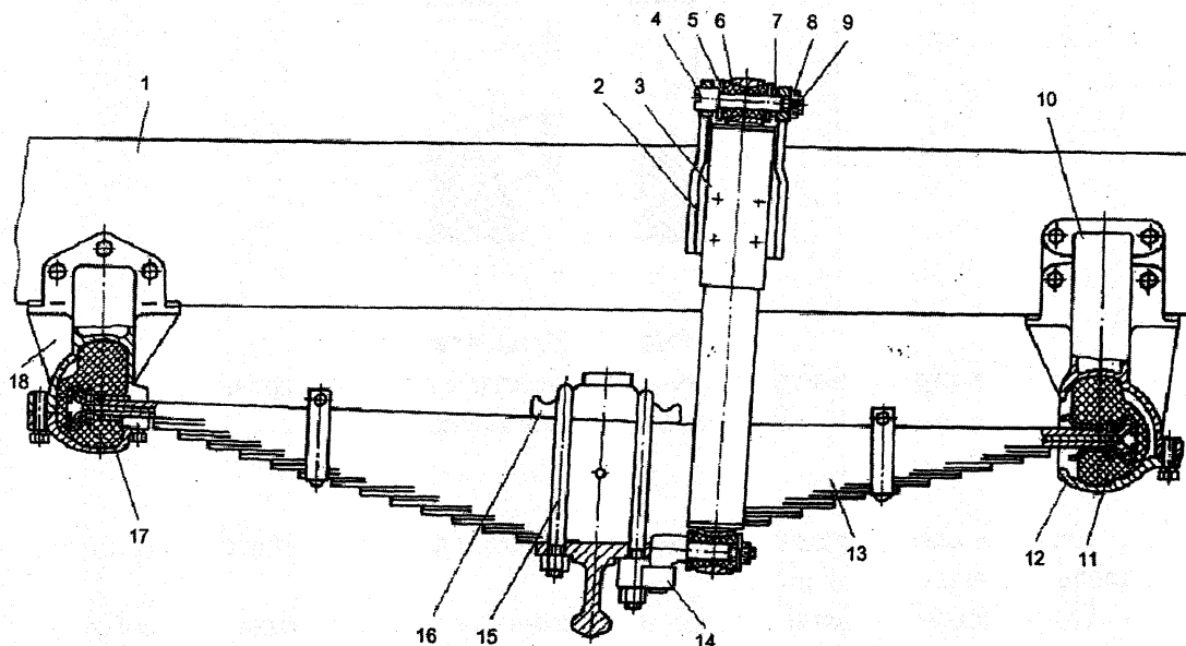
Рис. 43. Передняя подвеска:
