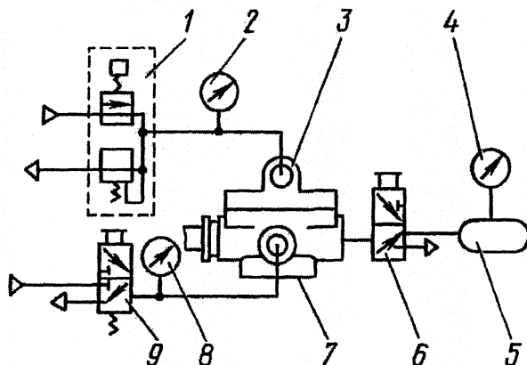
Рис. 82. Схема испытания ускорительного клапана:
