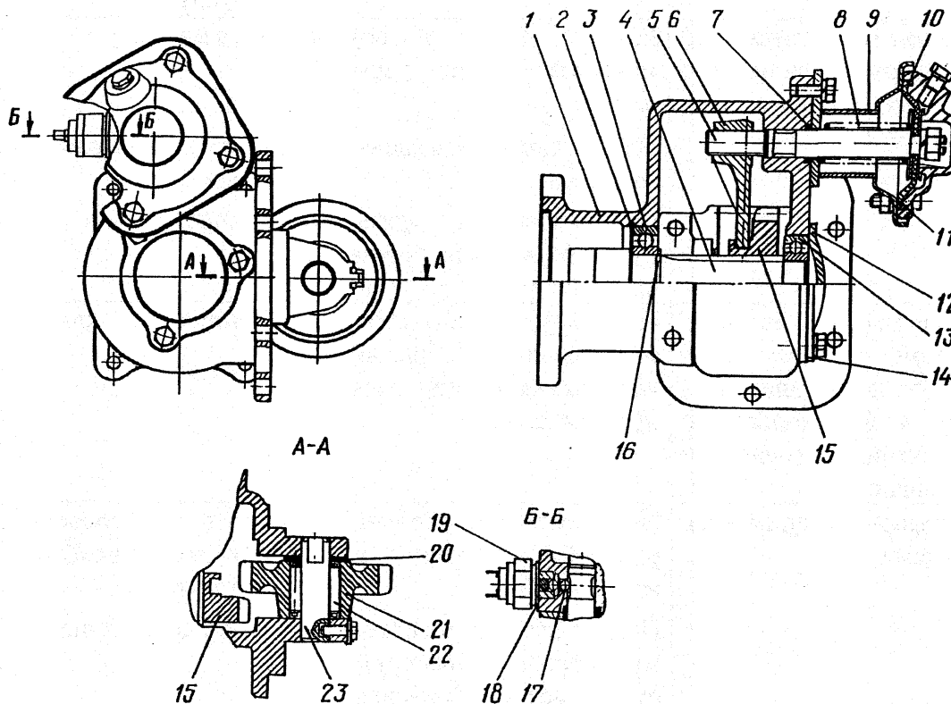
Рис. 103. Коробка отбора мощности:
