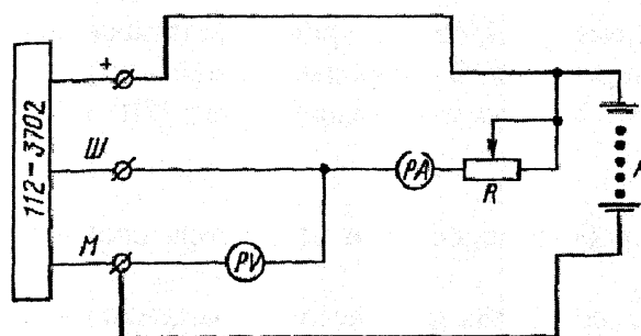
Рис. 98. Схема для проверки падения напряжения между выводами "М" и "Ш" генератора:
