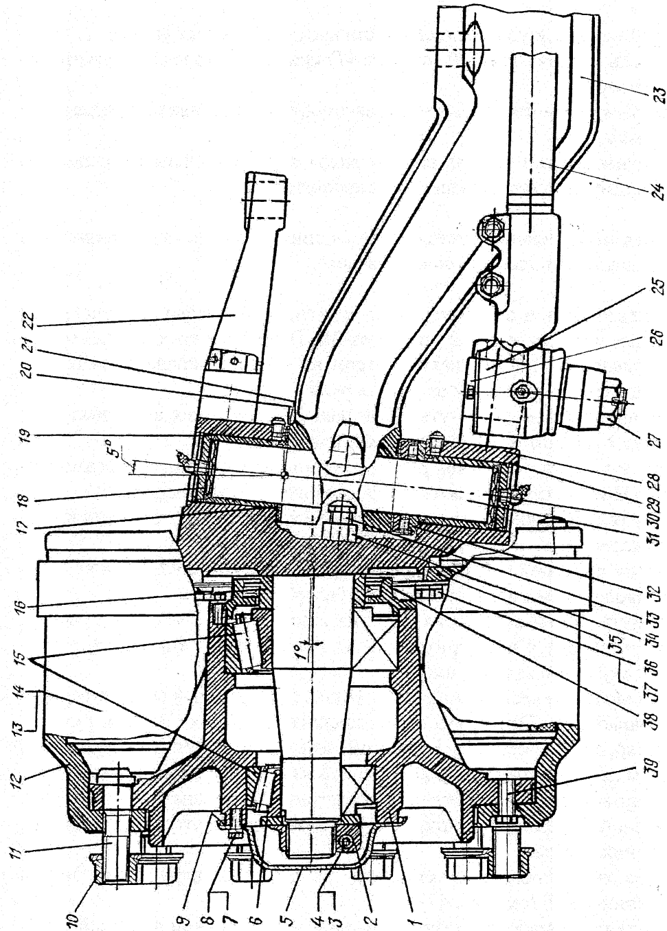
Рис. 47. Передняя ось
