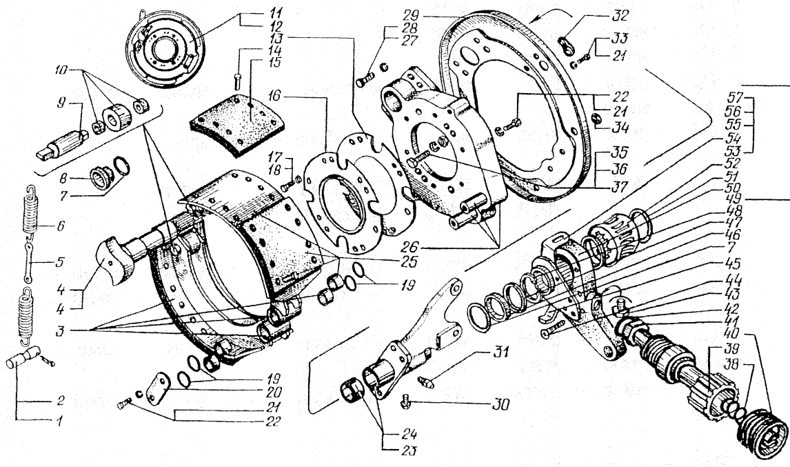
Рис. 89. Механизмы тормозные передних колес:
