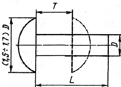
Рис. 40. Определение длины заклепки
