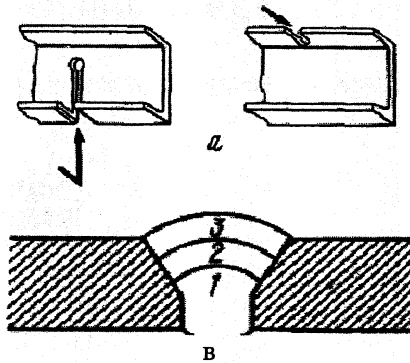
Рис. 42. Наплавка: а - направление наплавки (соответствует форме стрелки); в - трехслойная наплавка
