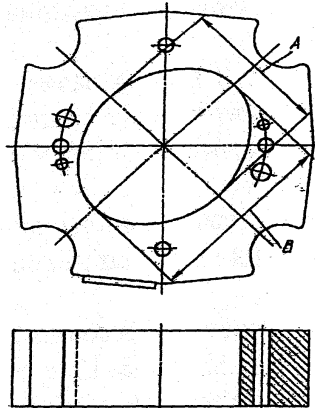
Рис. 61. Статор
