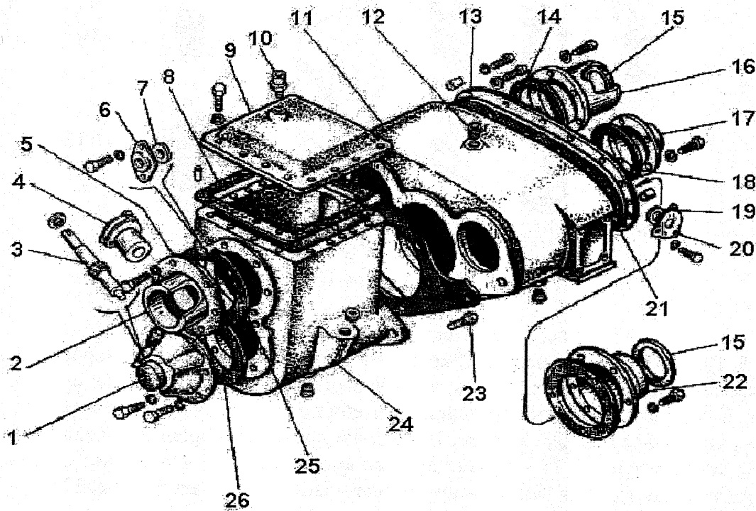
Рис.9. Раздаточная коробка:
