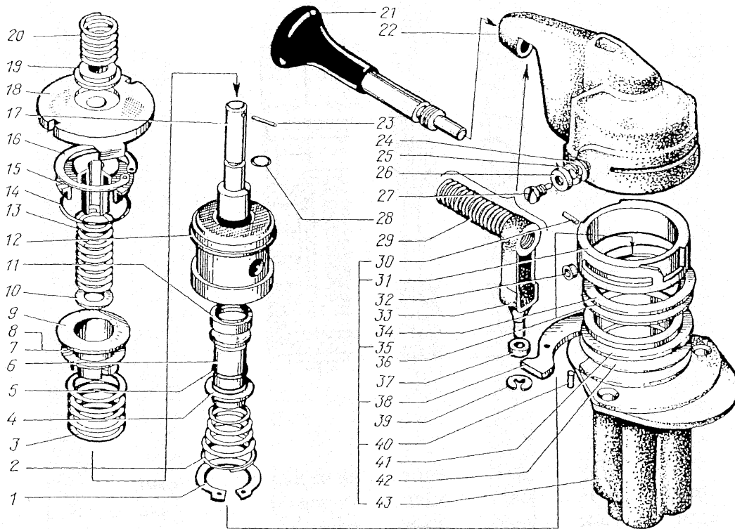
Рис. 76. Кран тормозной обратной действия с ручным управлением: 1, 16, 39 - кольцо упорное; 2, 3, 13, 20, 29 - пружина; 4, - шайба опорная; 5, 14, 28 - кольцо O-образное; 6 - корпус клапана; 7, 8, 10, 19, 24, 25, 26, 34, 36, 41, 42 - шайба; 9 - тарелка пружины; 11 - кольцо клапана; 12 - поршень; 15, 33 - направляющая; 17 - шток; 18 - колпачок направляющий; 21 - рукоятка; 22 - крышка; 23, 30, 40 - штифт; 27 - винт; 31 - кольцо; 32 - ролик; 35 - корпус крана в сборе; 37 - втулка; 38 - стопор; 43 - корпус
