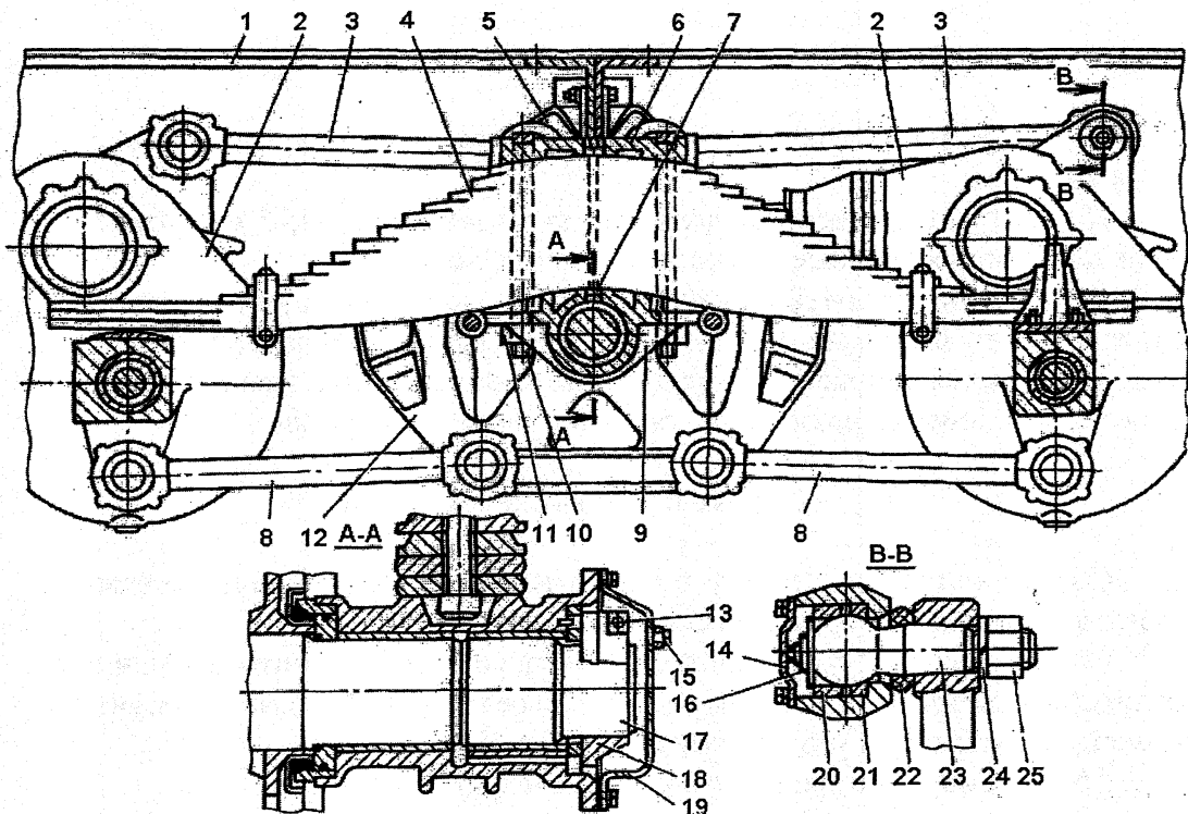
Рис. 46. Задняя подвеска
