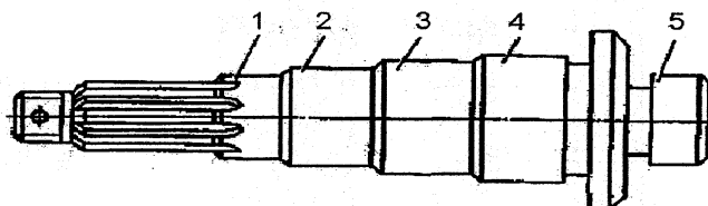
Рис. 17. Расположение шеек первичного вала раздаточной коробки:
