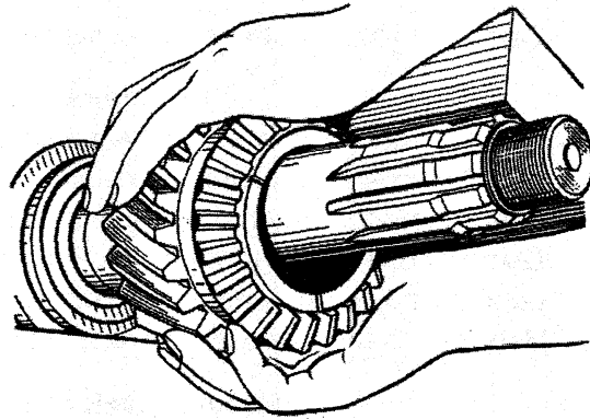
Рис. 15. Снятие шестерни привода заднего моста
