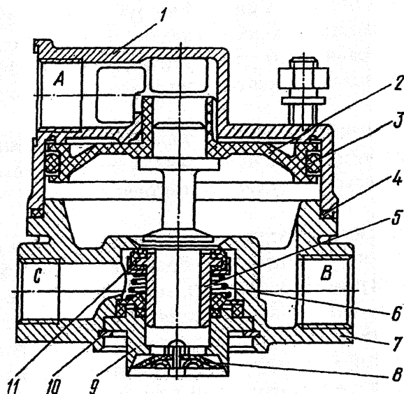
Рис. 74. Ускорительный клапан:
