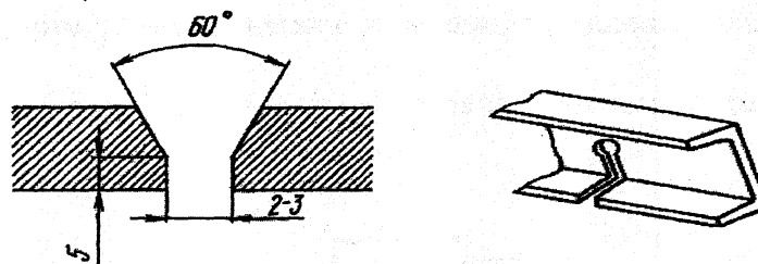
Рис. 41. Разделка трещин под наплавку
