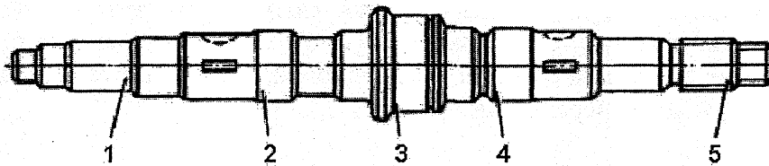
Рис. 18. Расположение шеек промежуточного вала раздаточной коробки: 1 - шейка под передний подшипник; 2 - шейка под шестерню высшей передачи; 3 - шейка под средний подшипник; 4 - шейка под шестерню привода заднего моста; 5 - шлицевая шейка под задний подшипник
