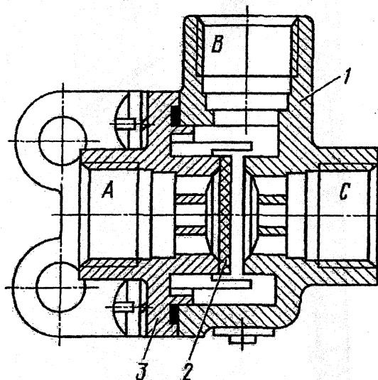
Рис. 75. Двухмагистральный перепускной клапан: 1 - корпус; 2 - мембрана; 3 - крышка; А - к ускорительному клапану; В - к полостям тормозных камер; С - к пневматическому крану
