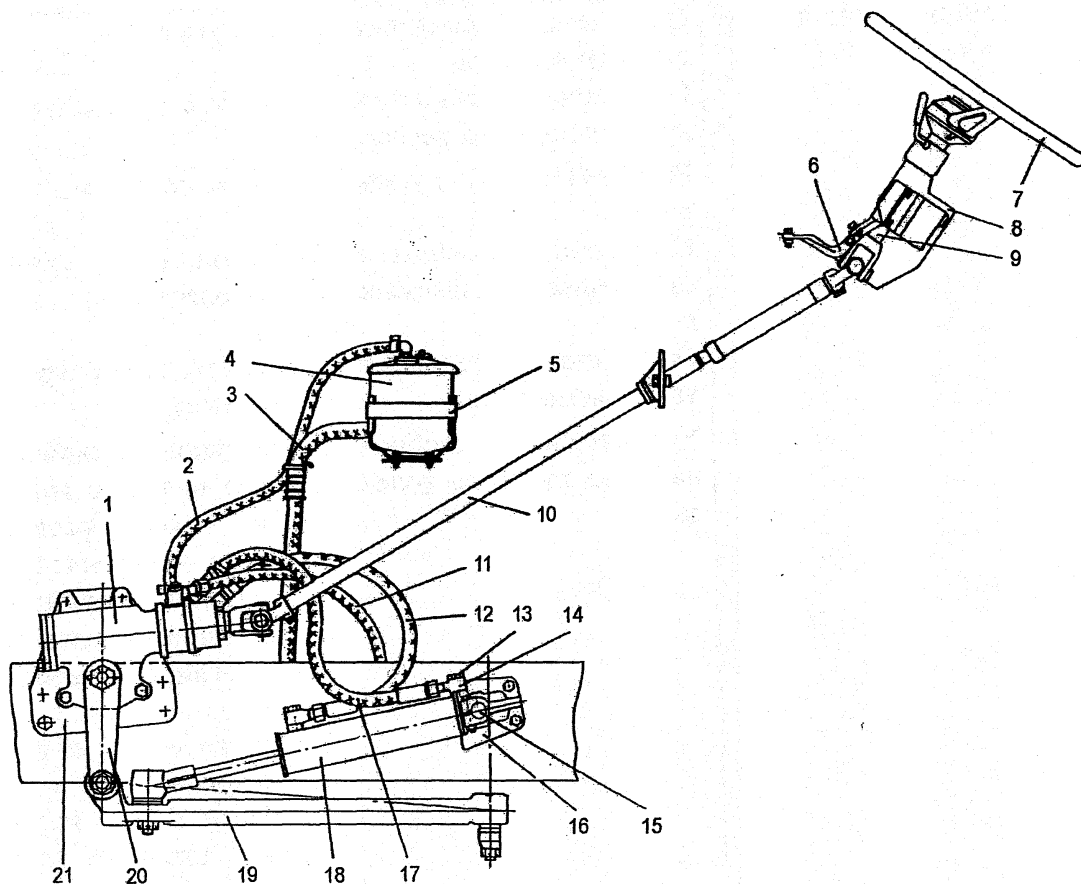
Рис. 52. Рулевое управление
