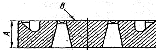
Рис. 62. Распределительный диск
