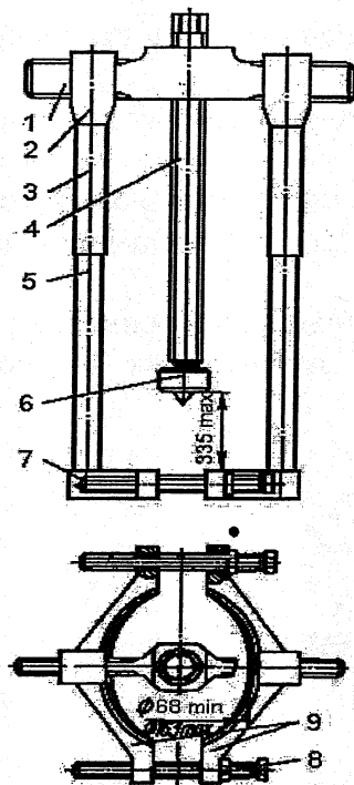
Рис. 10. Съемник для снятия подшипников и шестерен раздаточной коробки:
