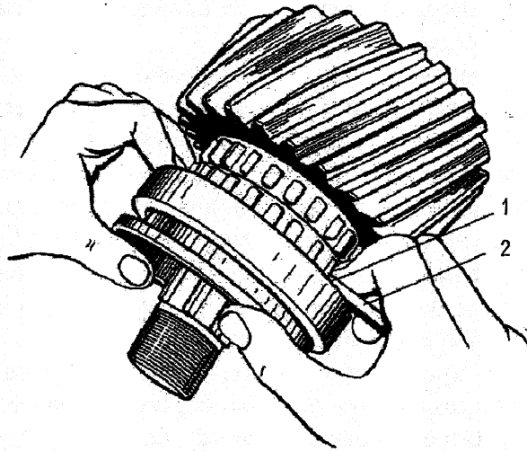
Рис. 26. Установка пружин и шариков-фиксаторов муфты блокировки дифференциала:
