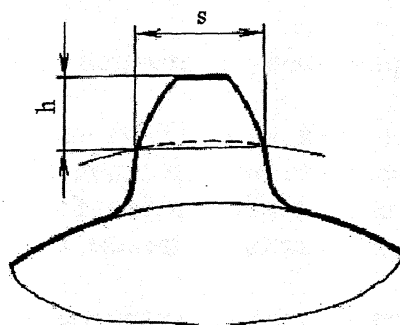
Рис. 20. Сечение зуба цилиндрических шестерён
