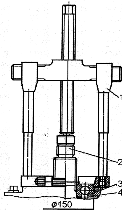
Рис. 11. Выпрессовка переднего подшипника первичного вала:
