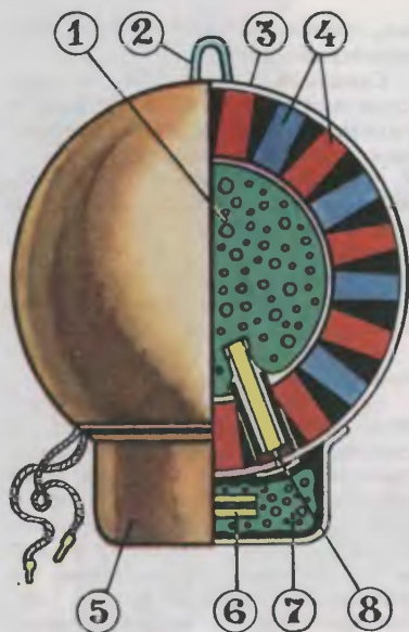
Фейерверочный снаряд для салютов: 1 — мешочек с порохом; 2 — петля для переноса снаряда; 3 — полусферический корпус снаряда; 4 — пирозлемент; 5 — станан вышибного заряда; 6 — электровоспламенитель; 7 — вышибной заряд; 8 — замедлитель.
