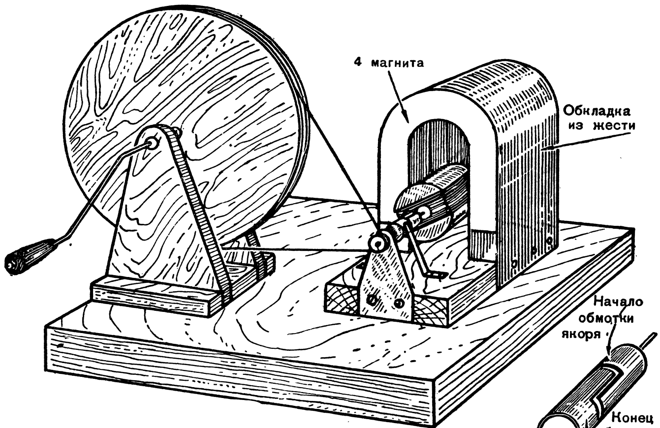
Рис. 1. Общий вид динамомашины
