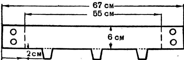
Рис. 4. Выкройка для обоймы из жести
