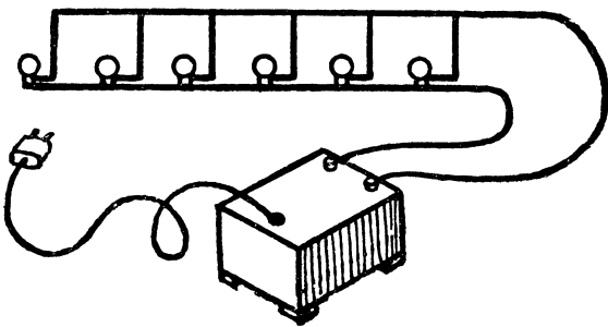
А. Соединение лампочек с одновременным зажиганием
