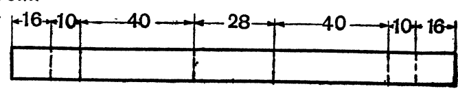
Рис. 10. Выкройка для первой нижней пластины сердечника электромагнита
