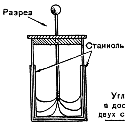
Рис. 3. Лейденская банка
