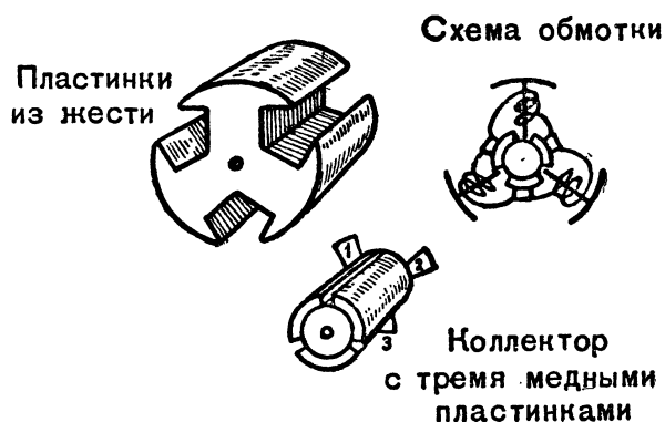
Устройство 3-полюсного якоря.
