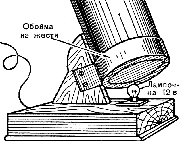
Рис. 5. Общий вид калейдоскопа с подставкой и лампочкой
