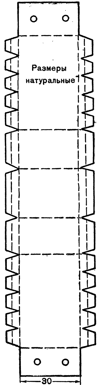
Рис. 2.6 Выкройка для верхней пластины сердечника
