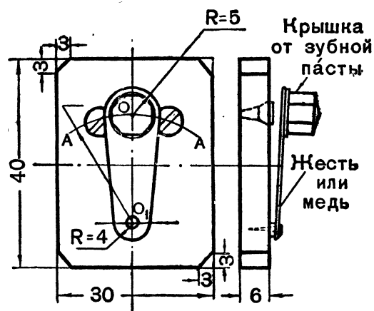
Рис. 2. Чертеж выключателя к электрическому фонарику
