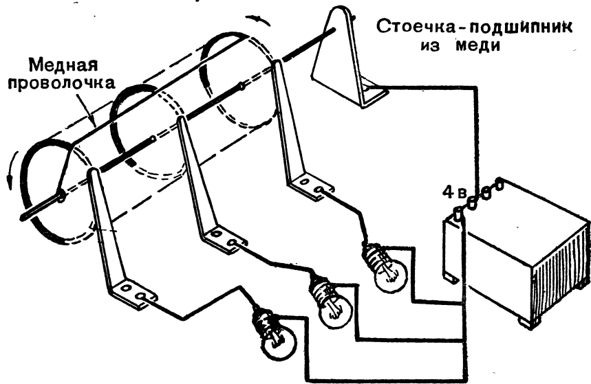
Рис. 1. Схема переключателя
