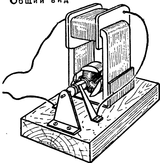
Рис. 1. Общий вид
