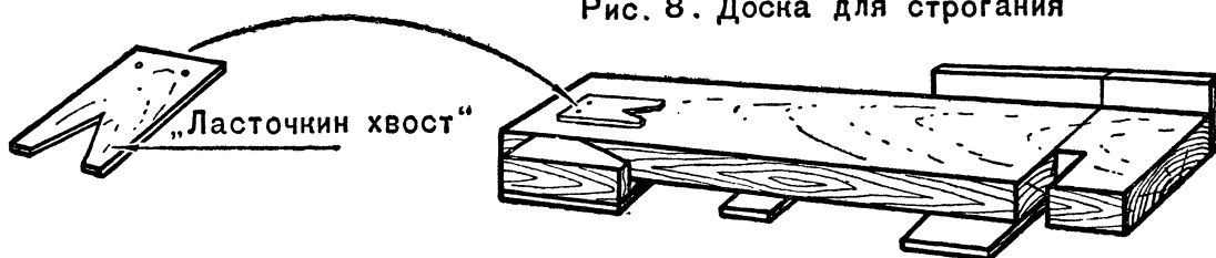
Рис. 8. Доска для строгания
