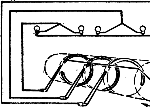
Рис. 2. Схемы соединений лампочек Б. Соединение лампочек с последовательным зажиганием
