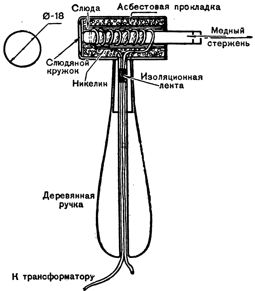
Рис. 2. Разрез паяльника
