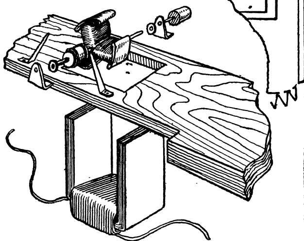
Рис. 4. Установка двигателя
