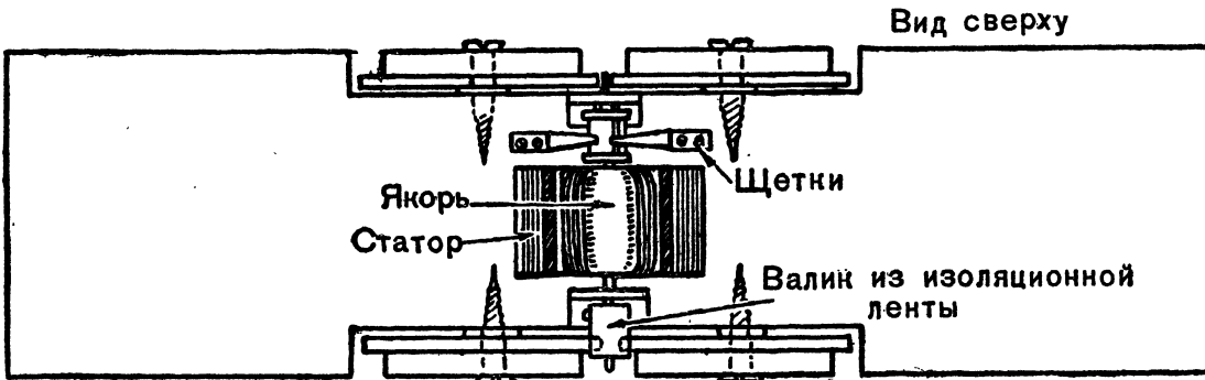
Рис.3. Устройство электродвигателя
