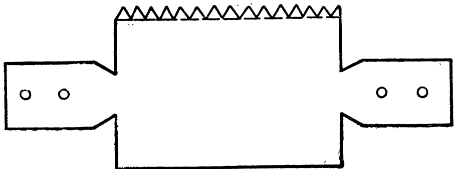
Рис. 3. Выкройка покрышки из жести
