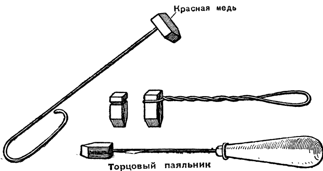
Рис. 19. Самодельные паяльники
