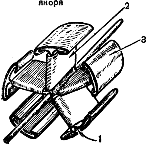
Собранный сердечник якоря
