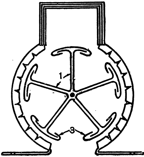
Собранный сердечник статора
