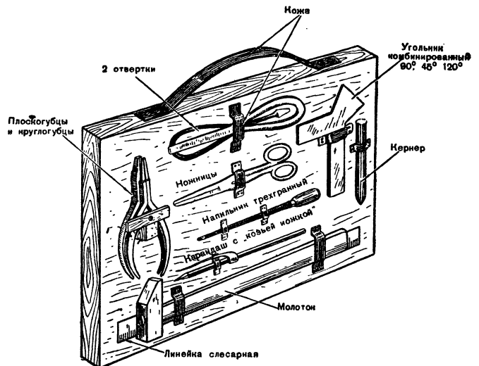
Рис. 15. Переносная монтажная готовальня
