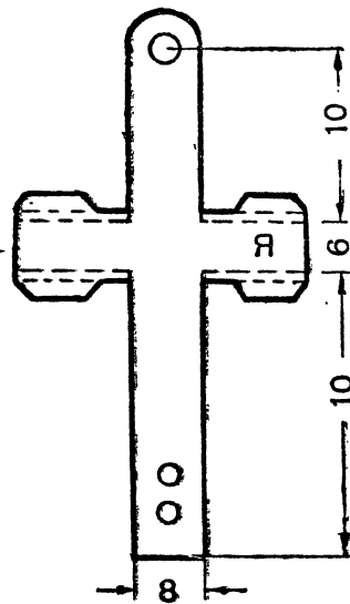
Рис. 3-Б. Части якоря и его сборка
