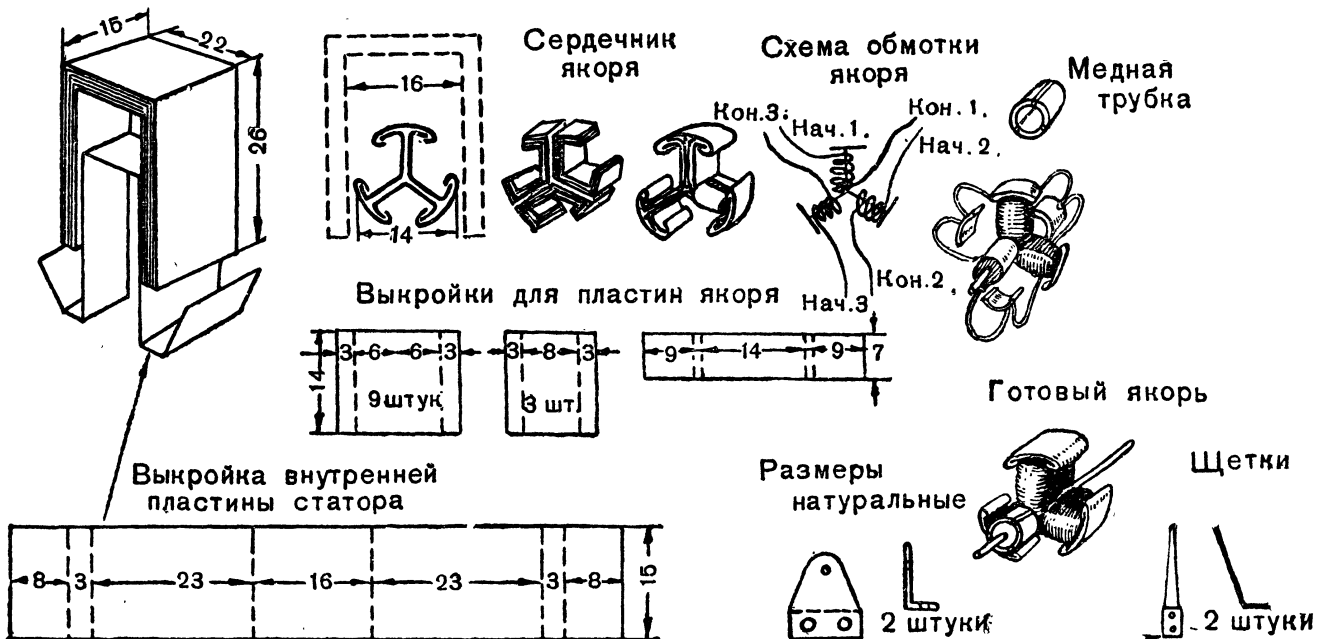
Рис.3. Устройство электродвигателя
