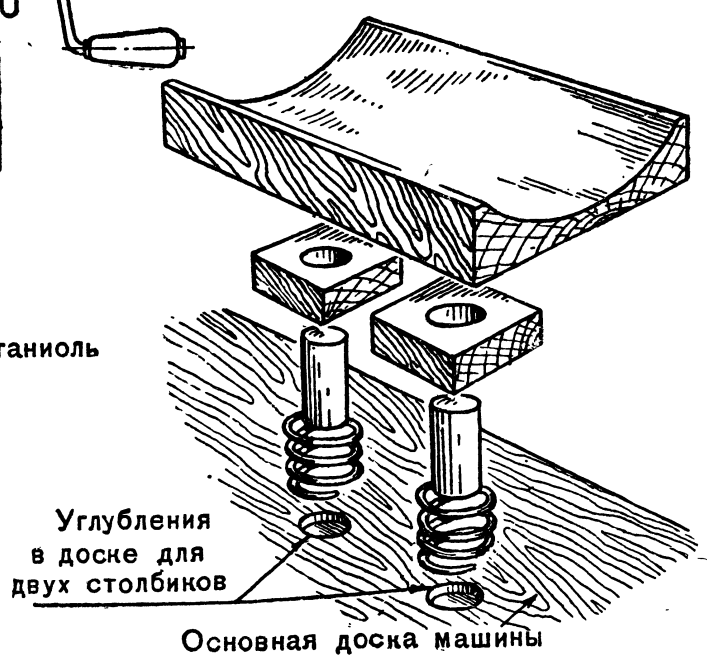
Рис. 2. Сборка подушки
