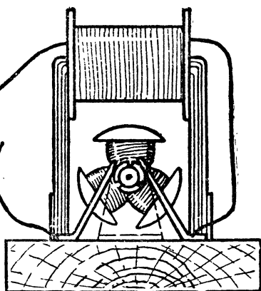
Вид сбоку
