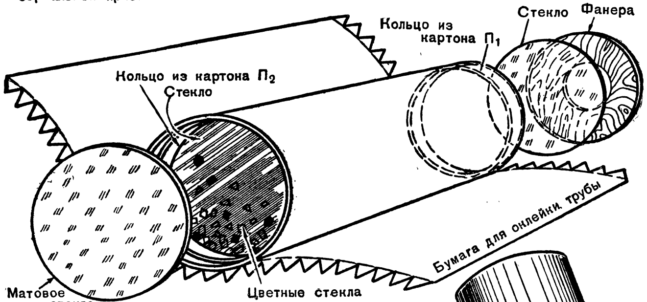
Рис. 3. Сборка калейдоскопа
