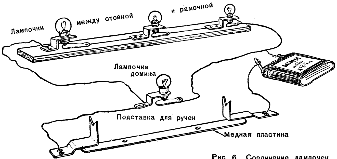
Рис 6. Соединение лампочек
