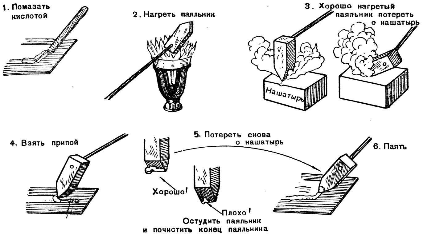
Рис. 20. Как правильно паять
