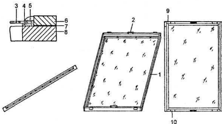
Рис. 30. Парниковые рамы, изготовленные собственными руками:
