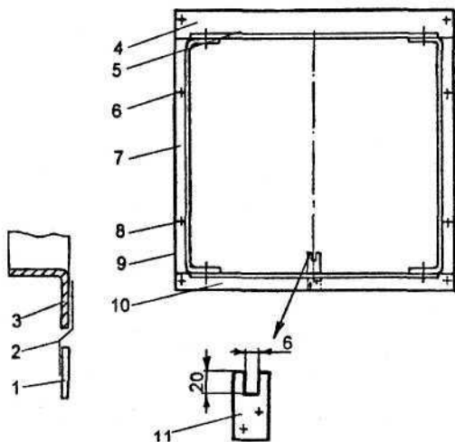
Рис. 14. Технология изготовления коробки для форточки в крыше и стене:
