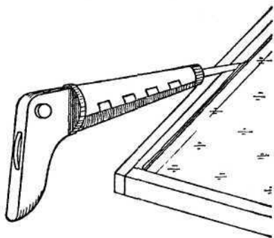
Рис. 24. Замазка, наносимая специальным шприцем
