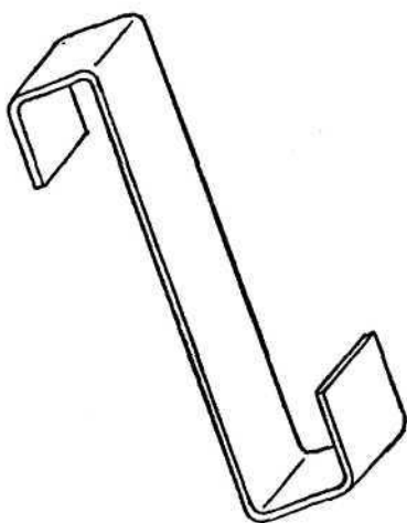
Рис. 19. S-образные крючки для фиксации стекол, установленных внахлест
