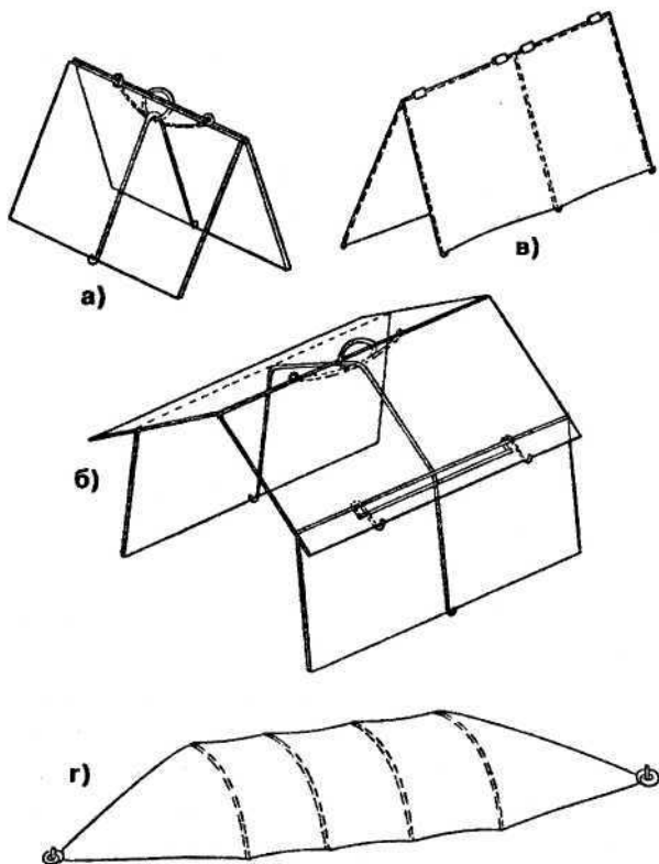
Рис. 33. Пленочные укрытия:
