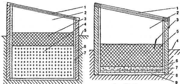
Рис. 32. Парник с электрообогревом:
