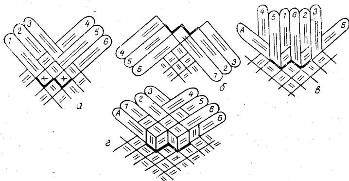
Рис. 12. Прибавка зигзагом с разведенными концами.
