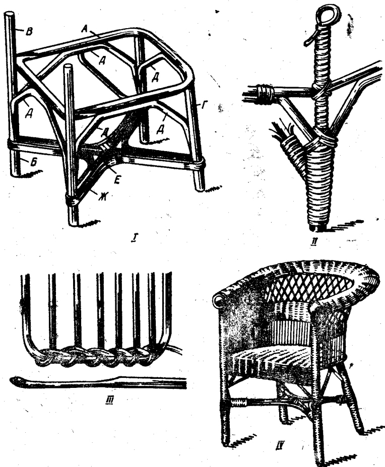
Рис. 56. Изготовление основных узлов плетеного кресла: I — каркас (остов): а — рамка, б — ножка передняя, в — стойка подлокотника, г — задняя ножка, д — упоры, е — крестовина, ж — пластина; II — способ оплетки передней ножки со стойкой и упором; III — способ крепления основы сиденья на рамку каркаса, IV — кресло в готовом виде.
