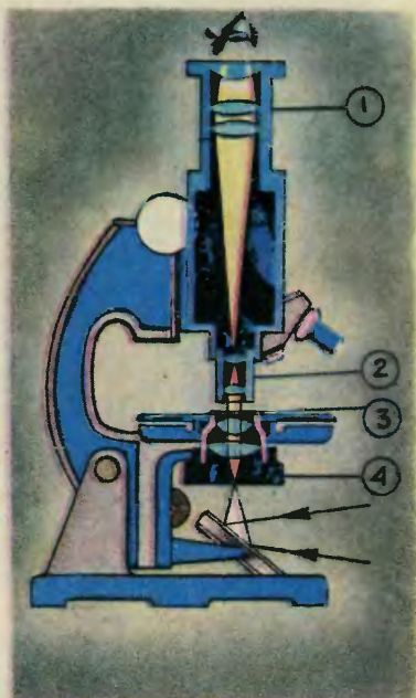
Схема оптического микроскопа: 1 — окуляр; 2 — объектив; 3 — объект исследования; 4 — осветительная система.
