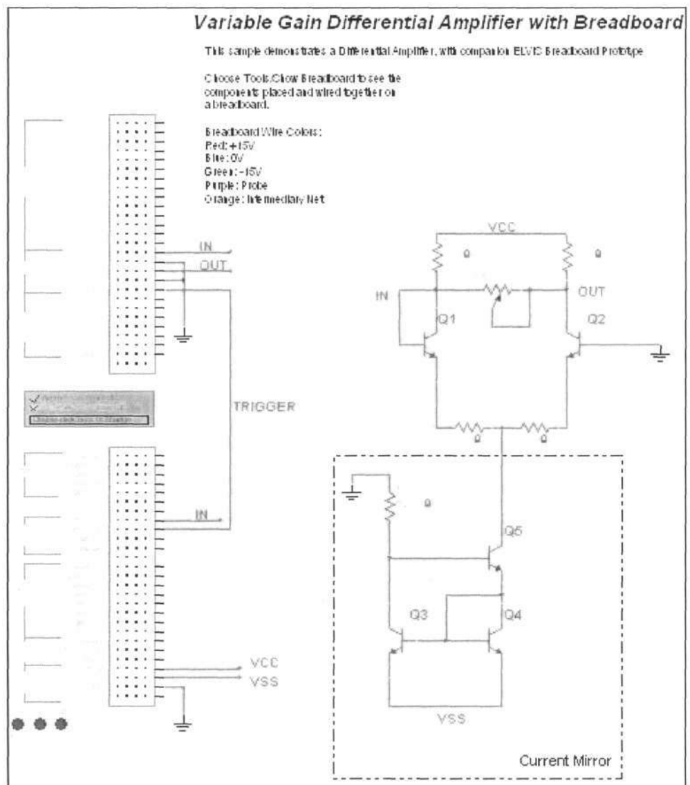
Рисунок 67 - Схема 3D ELVIS
