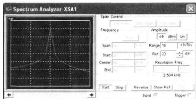
Рисунок 44 — Лицевая панель спектрального анализатора. Function Generator Front Panel
