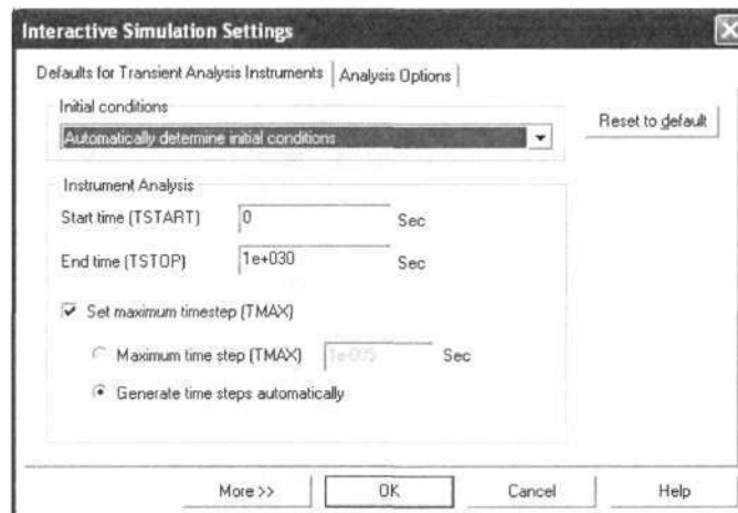
Рисунок 28 — Настройки интерактивной эмуляции
