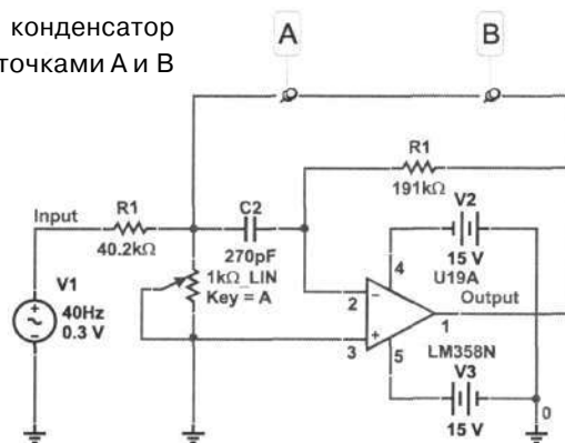
Рисунок 20 — Полосовой фильтр
