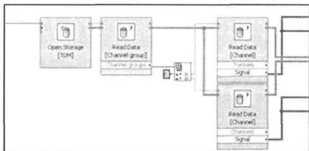
Рисунок 62 — Загрузка нескольких графиков из файла .TDM.
