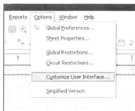
Рисунок 7 — Настройка меню
