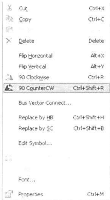
Рисунок 14 — Поворот компонента
