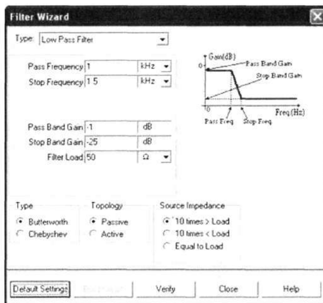
Рисунок 22 — Диалоговое окно мастера фильтров (Filter Wizard)
