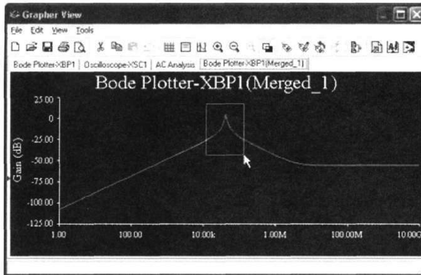
Рисунок 56 — Увеличение масштаба наложенных графиков
