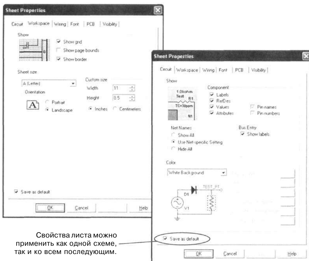
Рисунок 5 — Свойства листа
