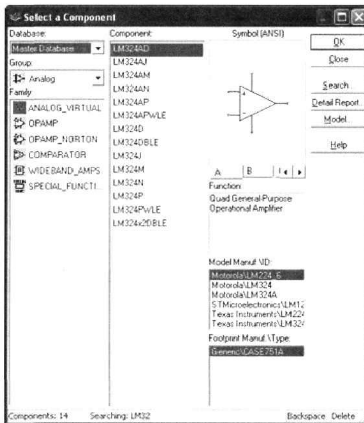
Рисунок 12 — Проводник компонентов
