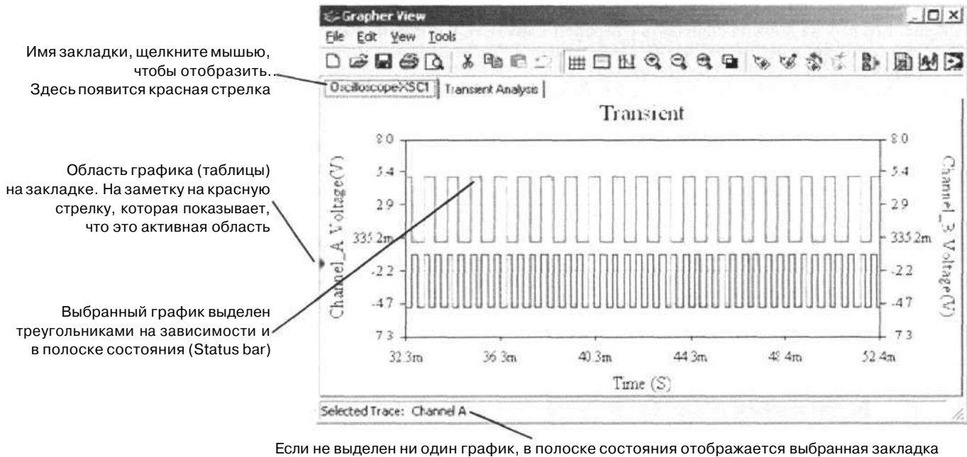
Рисунок 49 — Плоттер
