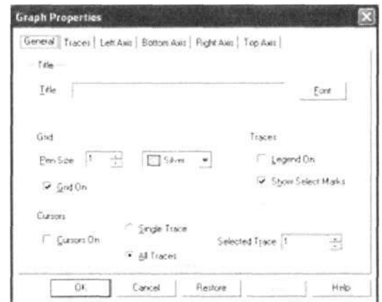
Рисунок 51 — Свойства графика
