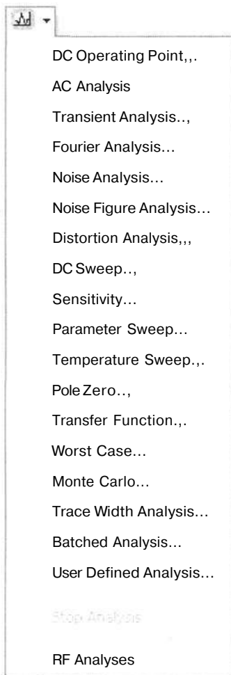
Рисунок 47 — Функции анализа
