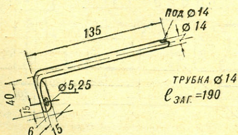
РИС. 29. ПОДКОС БАГАЖНИКА.
