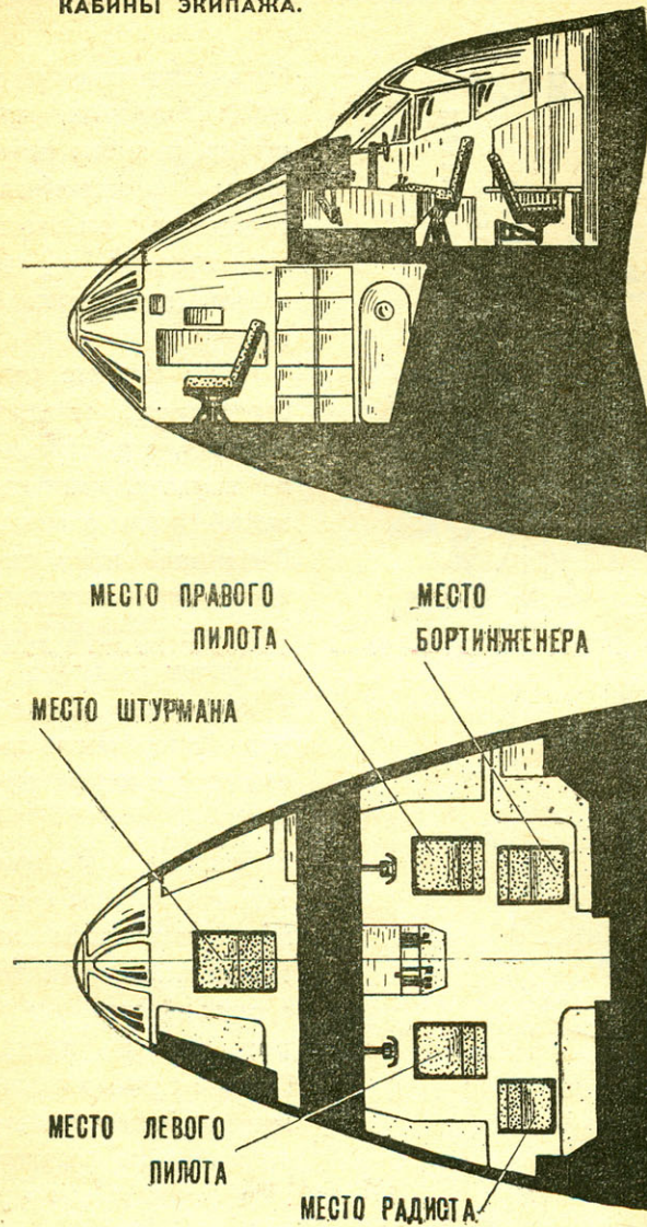
РИС. 3. КОМПОНОВКА КАБИНЫ ЭКИПАЖА.
