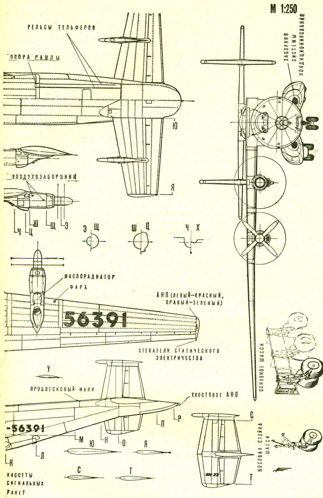
МОДЕЛИ-КОПИИ САМОЛЕТА АН-22.
