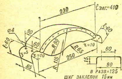
РИС. 34. КРЫЛО ПРИЦЕПА.
