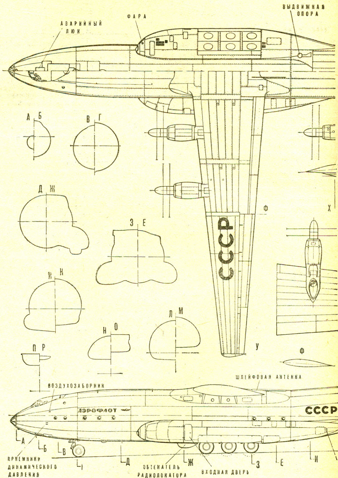
РИС. 2. КОНСТРУКТИВНО-КОМПОНОВочная СХЕМА
