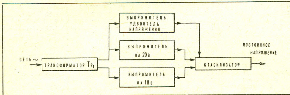
РИС. 1. БЛОК-СХЕМА СТАБИЛИЗАТОРА.
