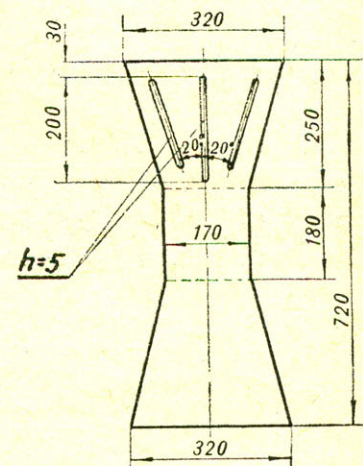
ДЕТ. 4. ПОДУШКА СИДЕНЬЯ
