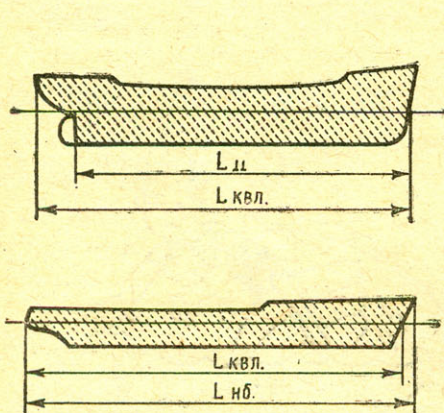
РИС. 1. ГЛАВНЫЕ РАЗМЕРЕНИЯ КОРАБЛЯ.
