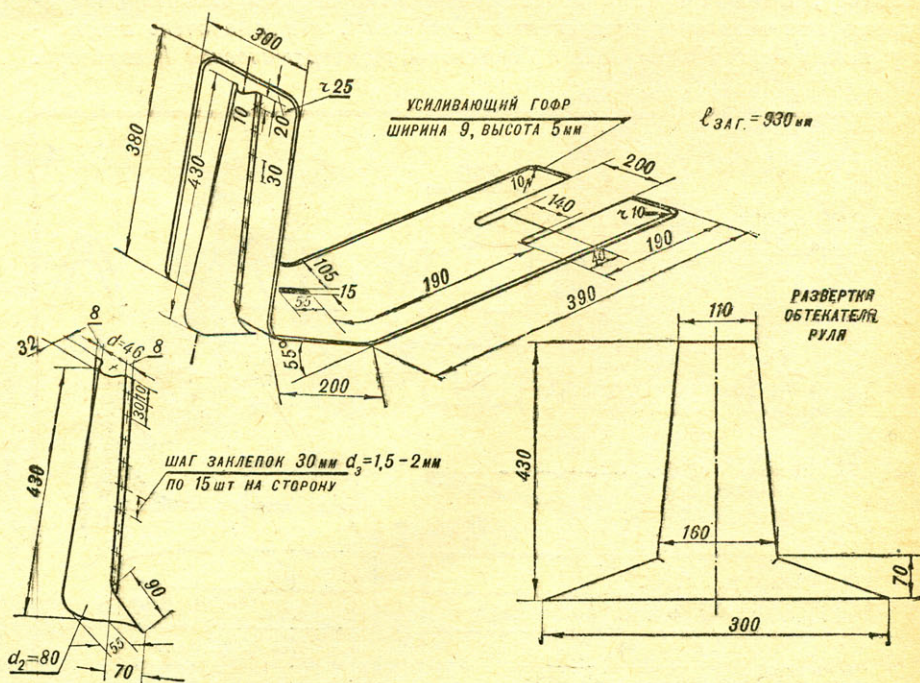
РИС. 20. ОБЛИЦОВКА.
