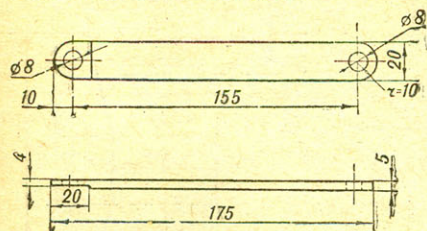
РИС. 34. КРЫЛО ПРИЦЕПА.
