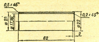
РИС. 17. ВТУЛКА РАСПОРНАЯ.
