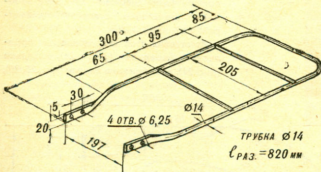
РИС. 28. БАГАЖНИК.
