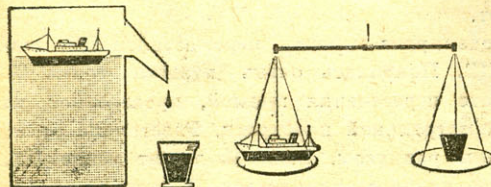
▼ РИС. 2. ОПРЕДЕЛЕНИЕ ВОДОИЗМЕЩЕНИЯ.
