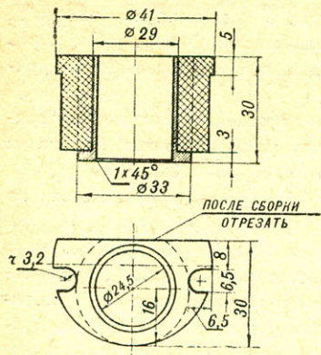
РИС. 21. ЦЕНТРИРУЮЩАЯ ВТУЛКА.
