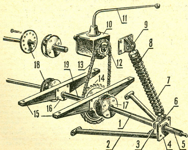
РИС. 3. ЗАДНИЙ МОСТ:
