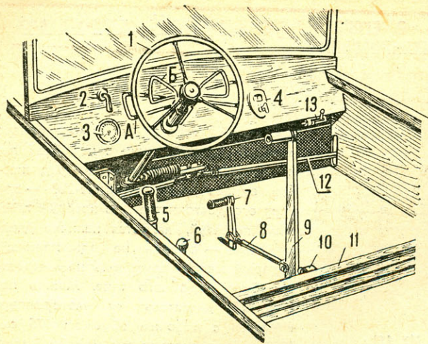
РИС. 2. РАСПОЛОЖЕНИЕ ОРГАНОВ УПРАВЛЕНИЯ АВТОМОБИЛЕМ В КАБИНЕ ВОДИТЕЛЯ:
