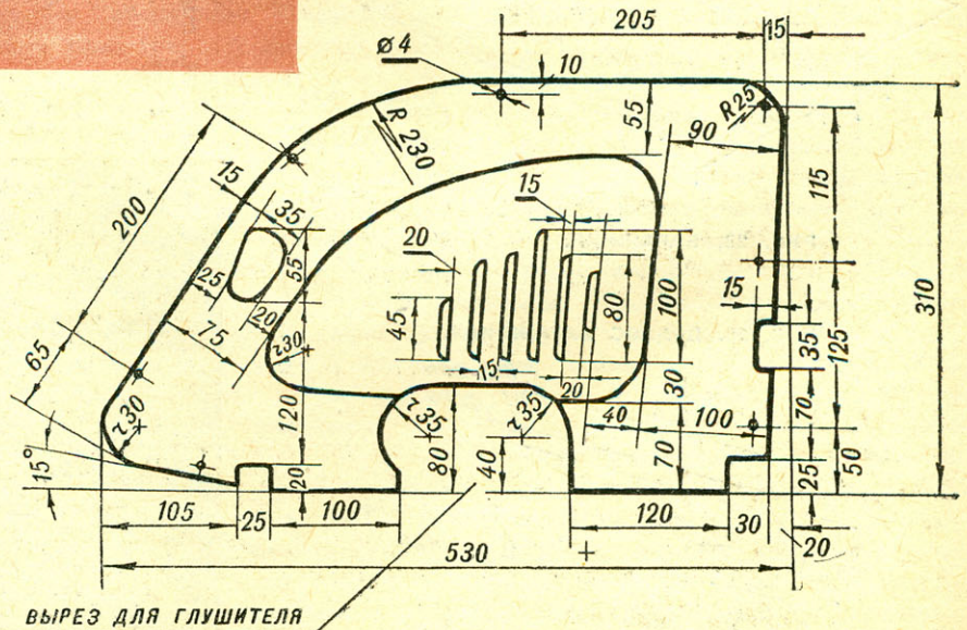
ВЫРЕЗ ДЛЯ ГЛУШИТЕЛЯ
