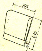
ДЕТ. 3. СПИНКА
