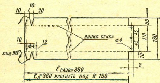
РИС. 27. БРЫЗГОВИК ВЕДУЩЕГО КОЛЕСА.
