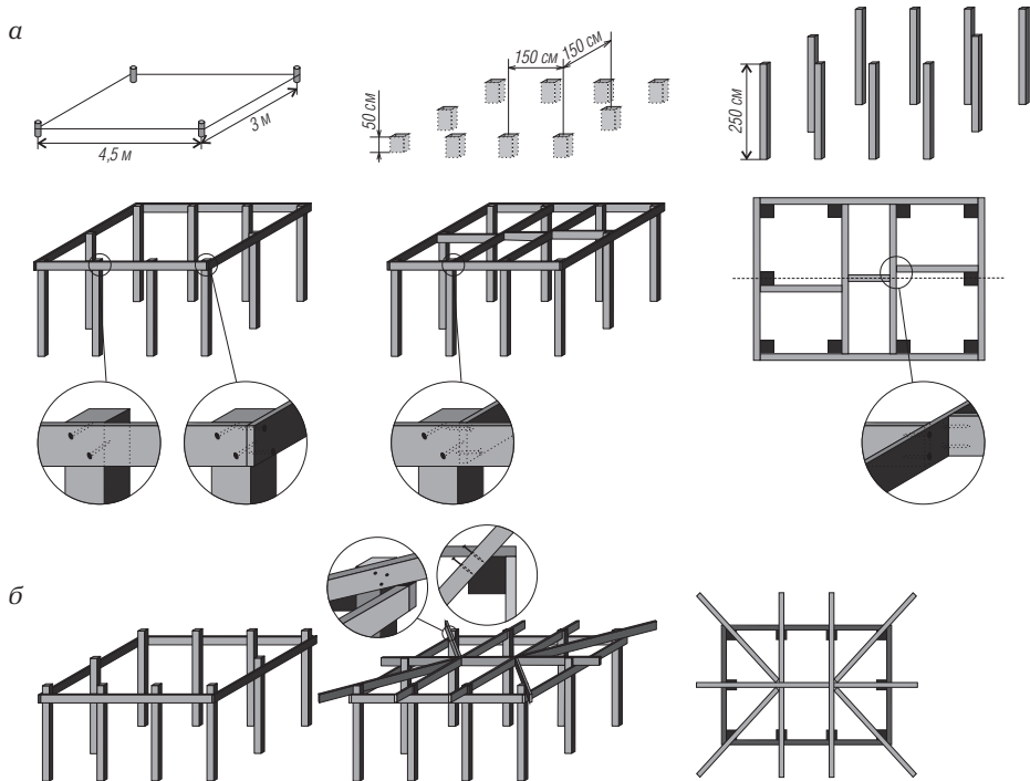
Рис. 16.19. Монтаж несущей конструкции беседки: а — без выпуска балок перекрытия; б — с выпуском балок перекрытия
