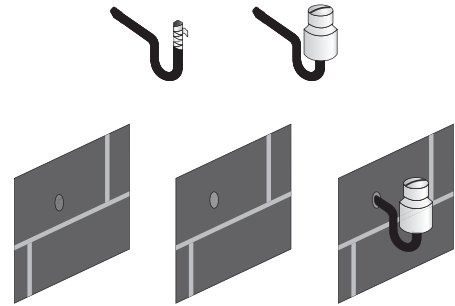
Рис. 13.13. Установка изолятора в монолитную стену
