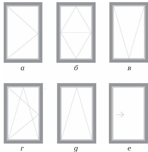
Рис. 6.10. Открывание окон: а — распашное; б — откидное верхней и нижней частей одновременно (поворот по оси в центральной части створки); в — откидное верхней части створки; г — поворотно-откидное; г — откидное нижней части створки; е — сдвижное
