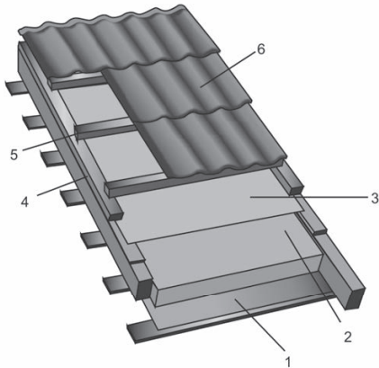
Рис. 5.27. Схема крыши деревянного дома с отапливаемым чердаком или мансардным этажом: 1 — пароизоляция; 2 — утеплитель (минеральная вата); 3 — ветровлагозащитная мембрана; 4 — контрорешетка; 5 — поперечная обрешетка; 6 — черепица
