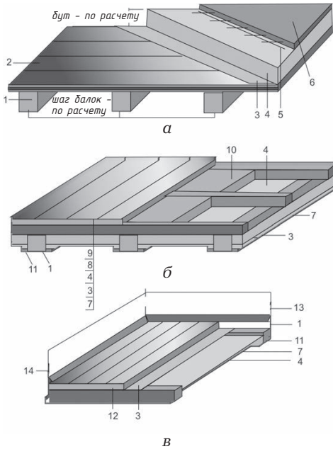
Рис. 5.1. Виды деревянных перекрытий: а — чердачное перекрытие с утеплением по верхней обшивке; б — перекрестное чердачное утепление; в — нащиповальное перекрытие с межбалочным утеплением: 1 — балки перекрытия; 2 — обшивка из досок; 3 — пароизоляция; 4 — первый слой утеплителя; 5 — арматурная сетка; 6 — паропроницаемая стяжка; 7 — деревянный (гощатый) накат; 8 — перекрестный каркас; 9 — обшивка из досок (либо паропроницаемая армированная стяжка); 10 — второй слой утеплителя; 11 — черепной брусок; 12 — деревянный пол; 13 — плинтус; 14 — щель воздухообмена
