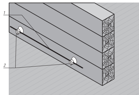
Рис. 8.9. Прокладка кабеля в доме с деревянными стенами: а — открытая проводка в кабель-канале: 1 — кабель-канал; 2 — кабель силовой; б — скрытая проводка на роликах: 1 — кабель; 2 — ролики
