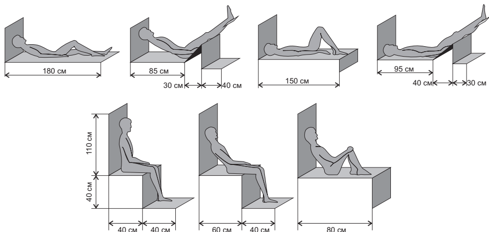
Рис. 15.4. Конструкции полок
