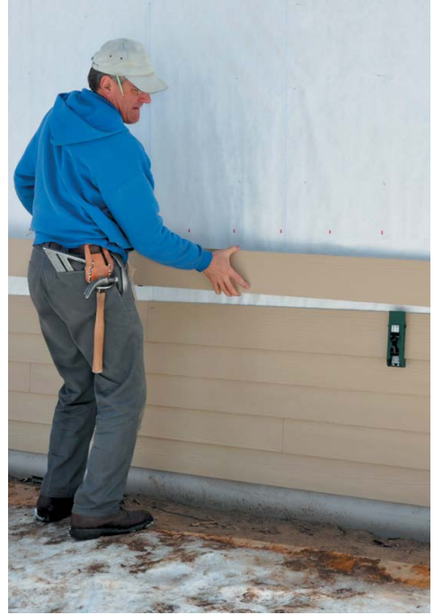
Рис. 43. Установка очередных ламелей
