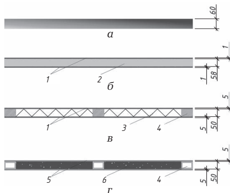
Рис. 6.19. Конструкции каркасных дверей: а — дверное полотно из массива; б — дверное полотно из МДФ; в — каркасное дверное полотно; г — дверь металлическая утепленная: 1 — шпон; 2 — МДФ; 3 — гофрированный картон; 4 — каркас; 5 — металл; 6 — утеплитель
