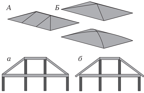
Рис. 16.20. Вальмовая (А) и шатровая (Б) кровли наслонного (а) и висячего (б) типов
