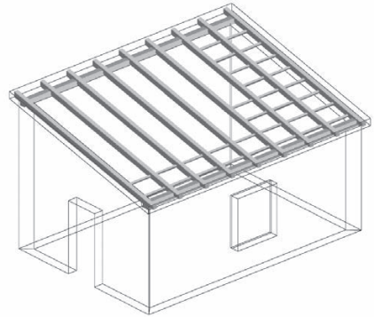
Рис. 5.6. Односкатная крыша
