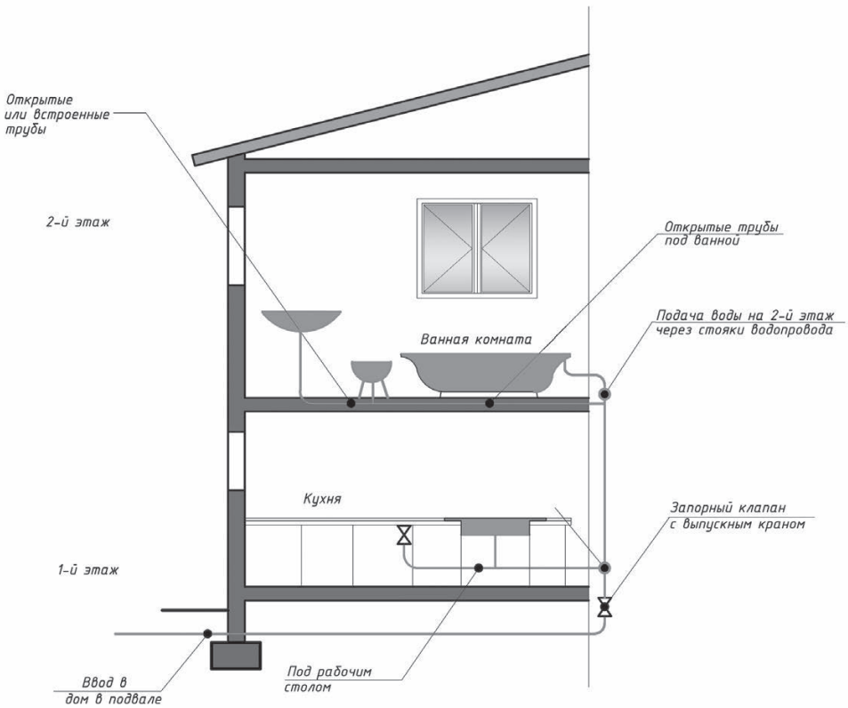
Рис. 9.18. Распределение воды в доме
