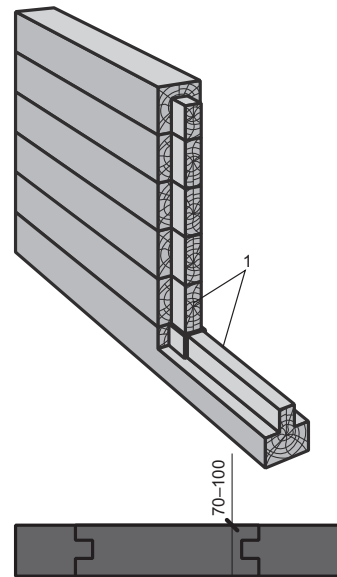
Рис. 4.14. Подушка с подоконной доской и гребнем (1)
