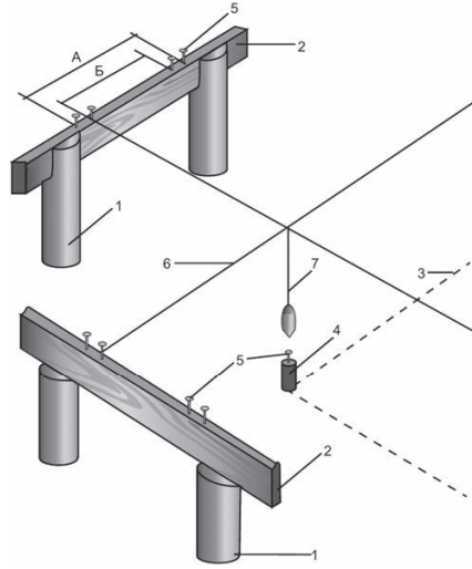
Рис. 2.10. Устройство обноски: а — ширина стены; б — ширина фундамента; 1 — столбики; 2 — доска; 3 — разметка наружных граней стен; 4 — кольшеч; 5 — гвозди; 6 — проволока или шпагат; 7 — отвес
