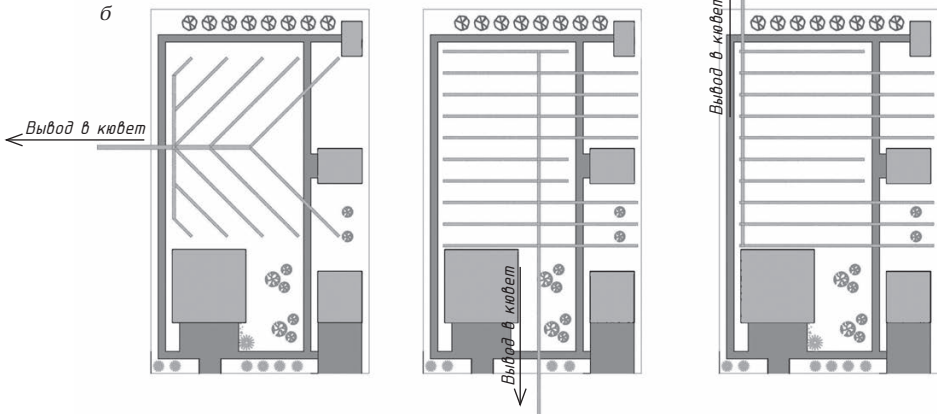
Рис. 2.3. Дренажные траншеи: а — схема размещения дренажных труб; б — схема устройства дренажа
