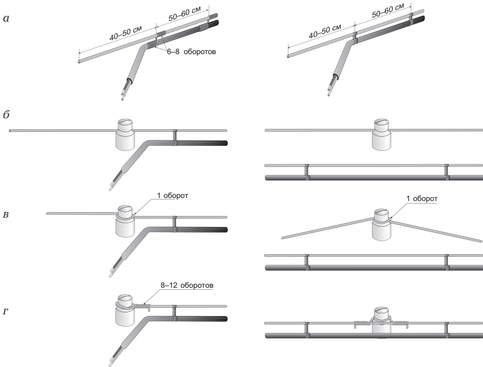
Рис. 13.11. Усиление кабеля и крепление к изоляторам: а — одножильным проводом; б — металлическим хомутом; в — крепление к последнему изолятору; г — крепление к промежуточному изолятору
