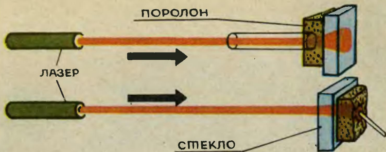
Схема опыта для демонстрации проникновения луча сквозь непрозрачный материал. В первом случае материал сдавливают стеклянной трубкой, во втором — надавливают с внешней стороны стеклянной палочкой.
