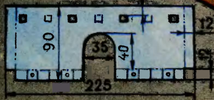
Выкройка топки
