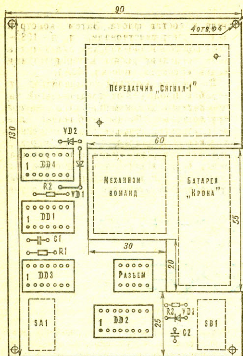
Рис 5. Схема расположения элементов на монтажной плате передатчика.
