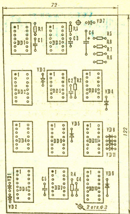
Рис 6. Схема расположения элементов на монтажной плате приемника.
