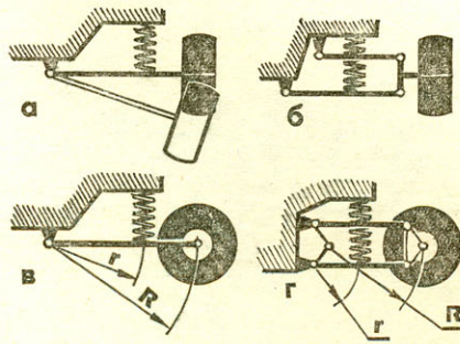
Рис. 1. Кинематические схемы основных типов независимых подвесок: а — однорычажная с поперечным рычагом, б — двухрычажная с поперечными рычагами, в — однорычажная с продольным рычагом, г — двухрычажная с продольными рычагами, д — с косым рычагом.
