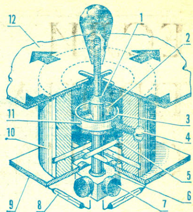
Рис. 3. Механизм подачи команд: 1 — рукоятка управления, 2 — втулка, 3 — кольцо, 4 — винт М3, 5 — стальная пружина, 6 — магнитодержатель, 7 — магнит, 8 — пластина, 9 — цилиндрический каркас, 10 — шпилька, 11 — корпус передатчика, 12 — корпус передатчика.
