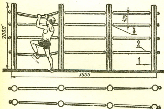
«Лианы»: 1 — стойки, 2 — обрезки резинового шланга, 3 — тросы.
