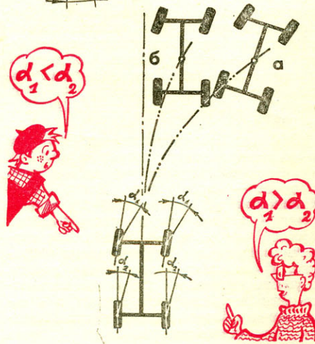
Рис. 3. Траектория движения автомобиля в зависимости от увода колес: а — угол увода передних колес меньше угла увода задних, б — угол увода передних колес больше угла увода задних.
