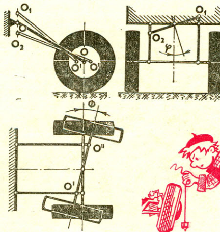
Рис. 5. Кинематическая схема зависимой подвески на двух продольных рычагах. ( O_1 и O_2 — крайние положения верхних шарниров рычагов при крене автомобиля на угол \varphi ; O' и O'' — положение нижних шарниров рычагов).
