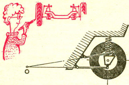
Рис. 4. Кинематическая схема зависимой подвески на четырех продольных рычагах.
