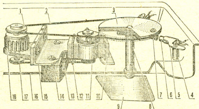
Рис. 4. Машинка привода руля: 1 — верхний шкив редуктора, 2, 13 — резиновые кольца, 3 — шкив руля, 4 — втулка, 5 — скоба, 6 — геркон, 7 — магнит, 8 — втулка оси руля, 9 — перо руля, 10 — электродвигатель, 11 — шкив электродвигателя, 12 — скоба, 14 — подставка, 15 — угольник, 16 — корпус судна, 17 — нижний шкив редуктора, 18 — редуктор.
