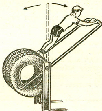
«Кузнечик»: 1 — рама, 2 — груз-противовес, 3 — стойка, 4 — ось.
