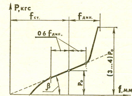
Рис. 6. График зависимости деформации упругого элемента подвесок f от усилия P .
