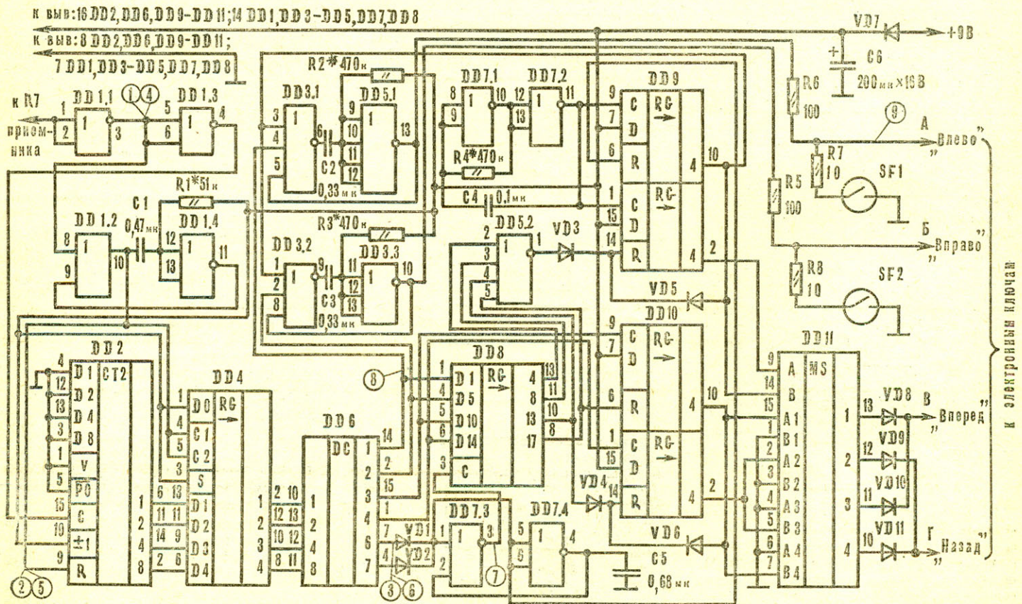
Рис. 1. Принципиальная схема дешифратора: DD1, DD7 K561LE5, DD2 K561HE11, DD3 K176LE10, DD4 K176HP3, DD5 K176LE6, DD6 K176ИД1, DD8 K176HP10, DD9, DD10 K176HP2, DD11 K561LC2, VD1 — VD11 Д9В.
