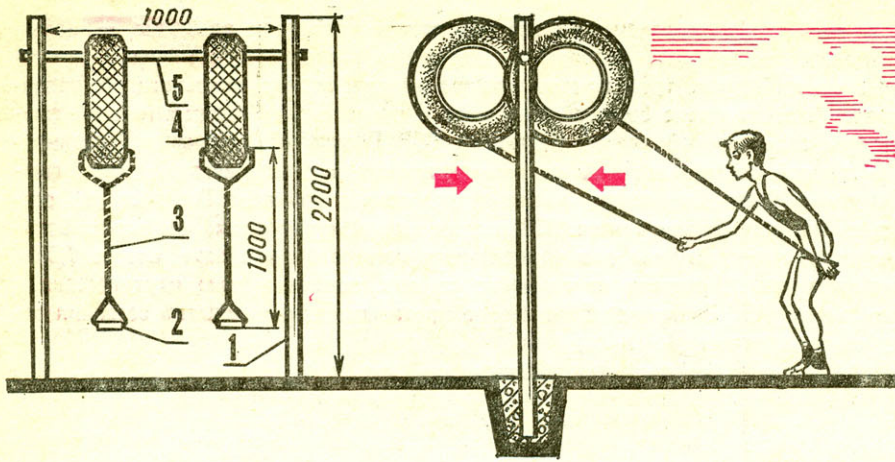
«Колокола»: 1 — стойка, 2 — ручка, 3 — трос, 4 — «колокол» из покрышки, 5 — перекладина.
