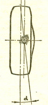
Рис. 2. Возникновение увода колеса автомобиля.
