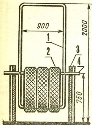
«Кузнечик»: 1 — рама, 2 — груз-противовес, 3 — стойка, 4 — ось.
