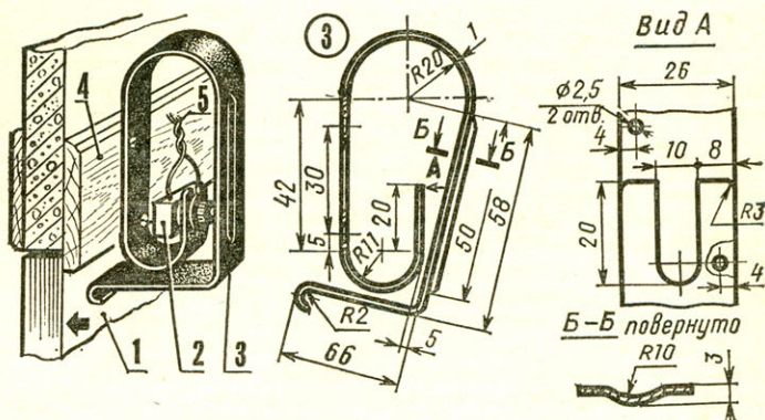
Автоматический выключатель: 1 — дверь, 2 — кнопочный выключатель, 3 — пластина-пружина, 4 — наличник, 5 — электропровода.
