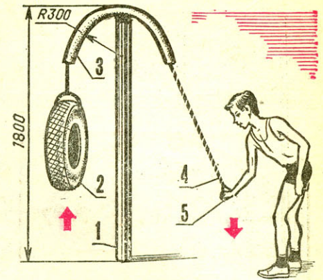
«Лесопилка»: 1 — стойка, 2 — покрышка, 3 — втулка, 4 — трос, 5 — ручка.
