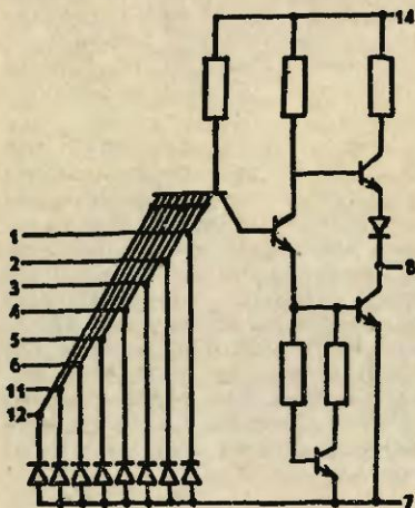
Рисунок 1. Принципиальная схема базового элемента серий К155, КМ155.
