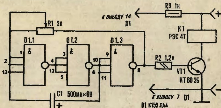
Рисунок 2. Принципиальная схема переключателя гирлянд.
