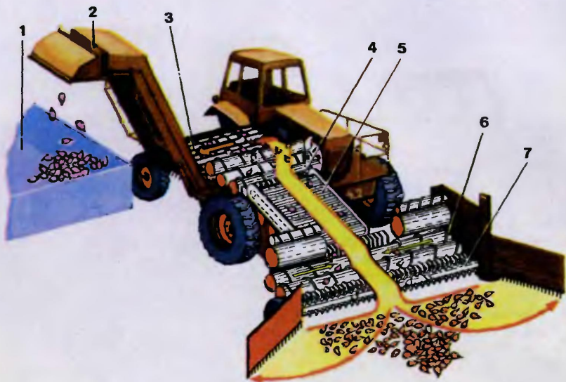
Технологическая схема свеклопогрузчика: 1 — кузов автомобиля; 2 — погрузочный транспортер; 3 — шнековый очиститель; 4 — битерный вал; 5 — продольный транспортер; 6 — приемные шнеки; 7 — ротационно-кулачковый вал.
