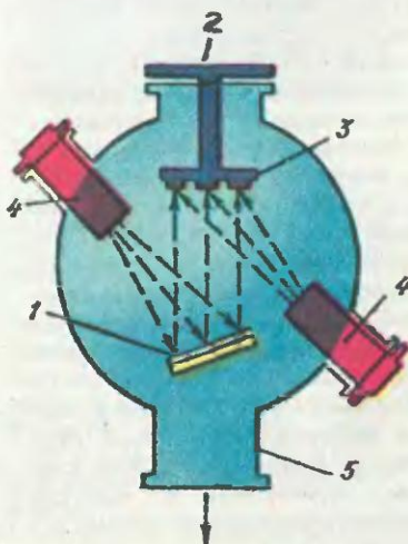
Схема одной из установок для получения алмазных пленок: 1 — катод; 2 — анод; 3 — подложка; 4 — источник излучения; 5 — корпус.
