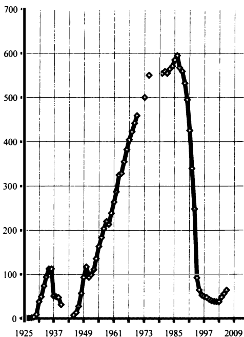
Рис.11. Производство тракторов в СССР и СНГ (в 2003—2006 гг. без Казахстана и Узбекистана, которые в 1997 г. дали около 4 тыс. тракторов). Экспорт тракторов из СССР в 1980 г. 50 тыс. штук, в 1986 г. 39 тыс. Импорт 5—6 тыс.
