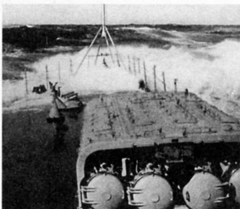
Вверху: 500-мм торпедный аппарат "Дойчланда", март 1933 г. В 1935 г. 500-мм аппараты заменены на 533-мм, защищенные легкой броней (справа).
