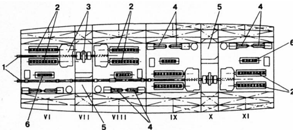
Схема энергетической установки "карманного линкора" "Адмирал граф Шлее": 1 — гребные валы; 2 — главные дизели; 3 — редукторы; 4 — дизель-генераторы; 5 — погреба 150-мм орудий; 6 — вспомогательные дизели.
