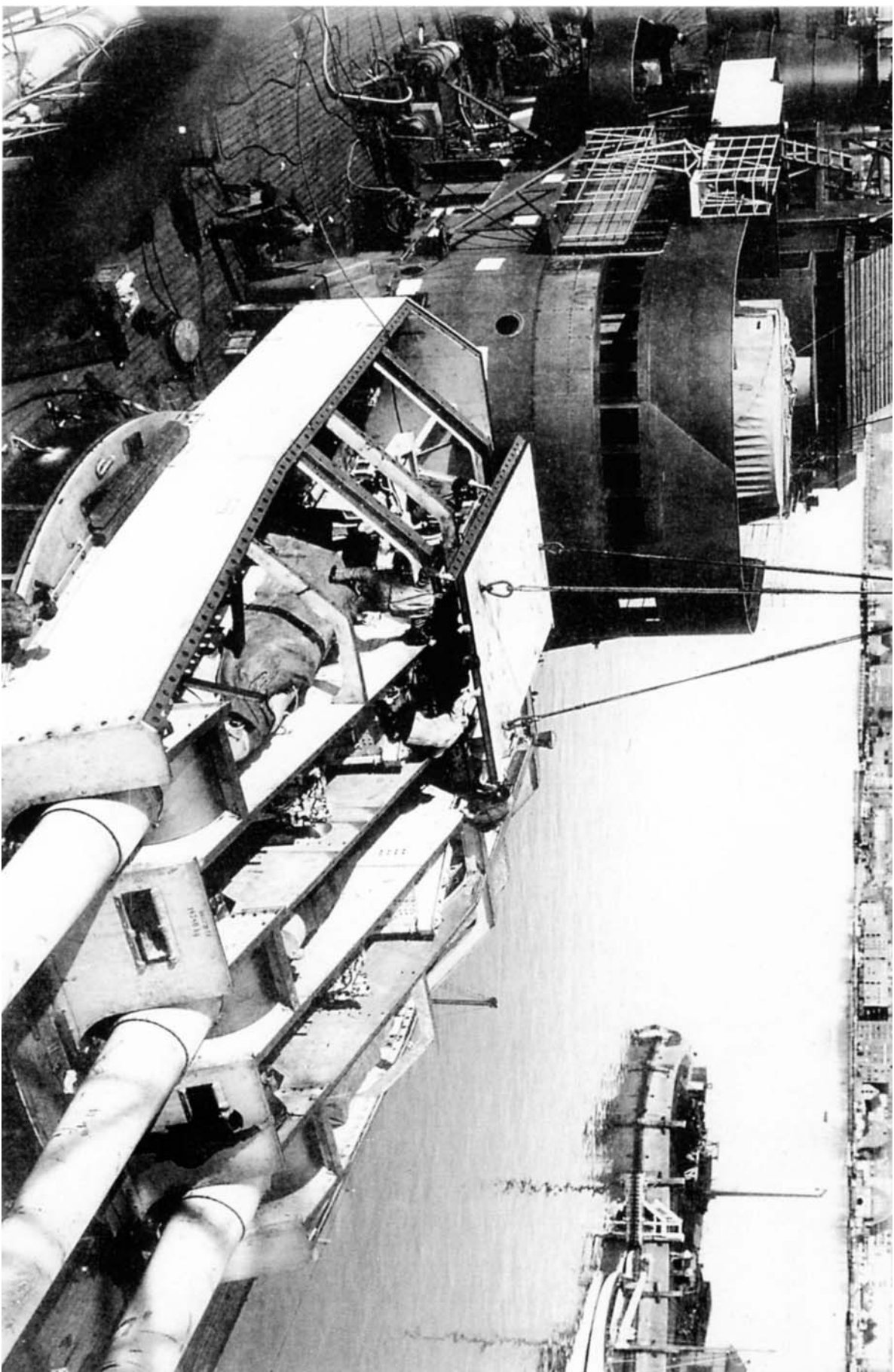
Носовая башня "Дойчланда" в процессе монтажа броневых плит крыши, 1932 г.
