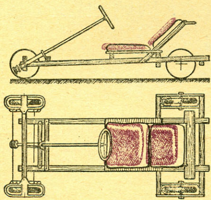
Рис. 1. Схема мини-кара класса (формулы А).
