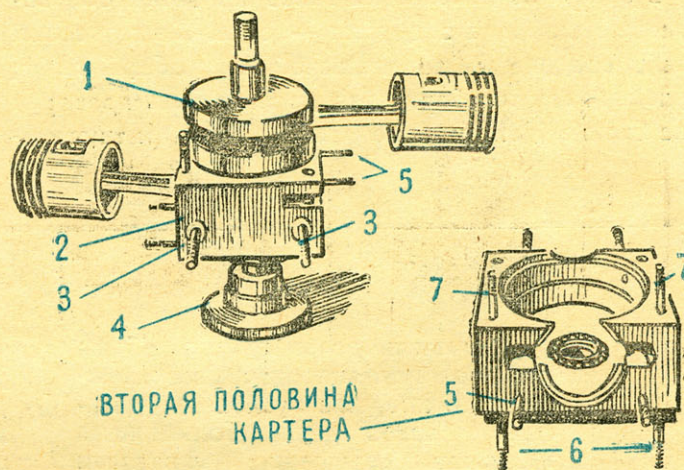
Рис. 6. Детали двигателя ББ-1: 1 — кривошип левого цилиндра, 2 — левая половина картера, 3 — болты крепления к подмоторной раме, 4 — шкив привода тахогенератора, 5 — болты крепления цилиндров к картеру, 6 — болты крепления к подмоторной раме, 7 — болты крепления половинок картера.
