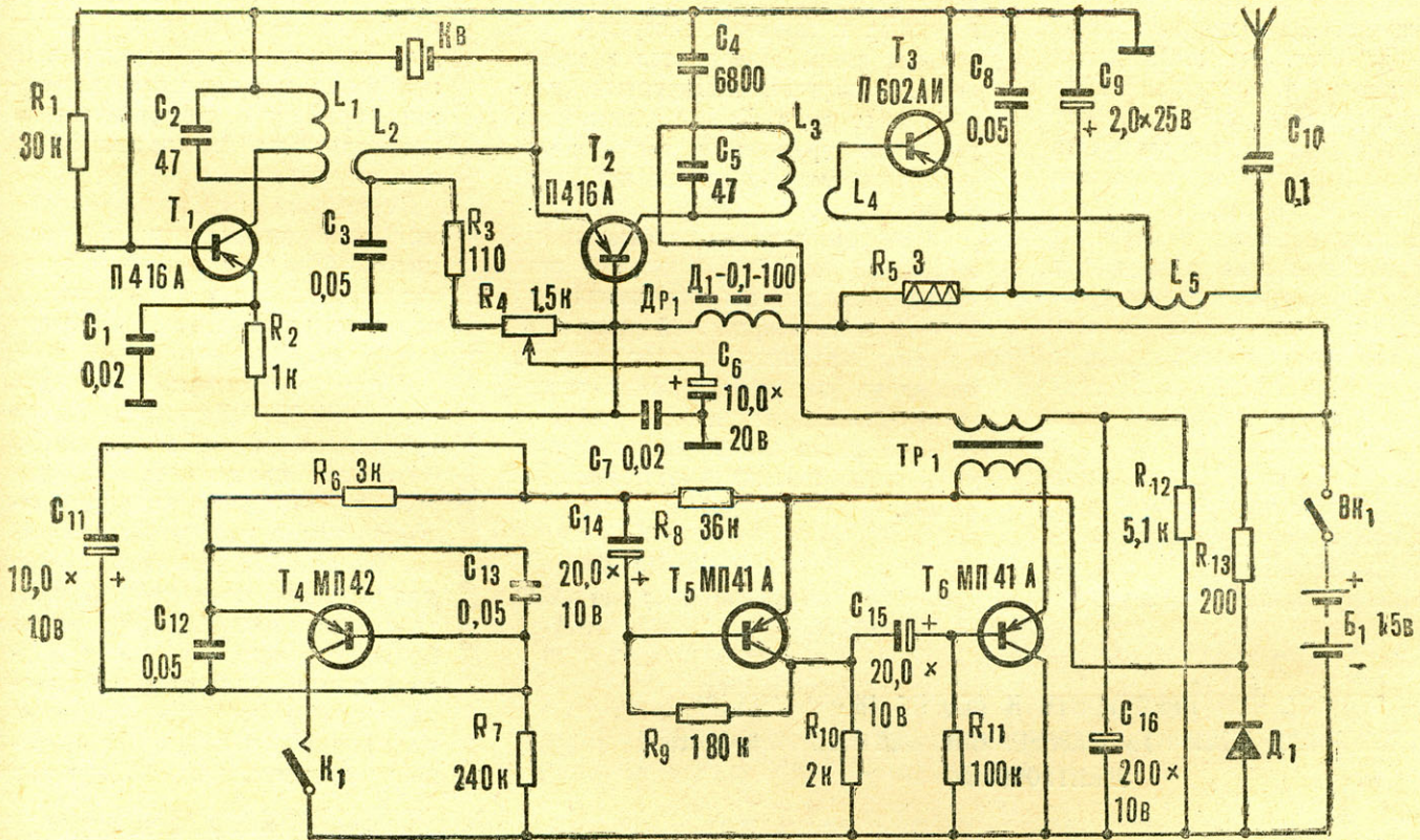
Рис. 3. Схема передатчика.
