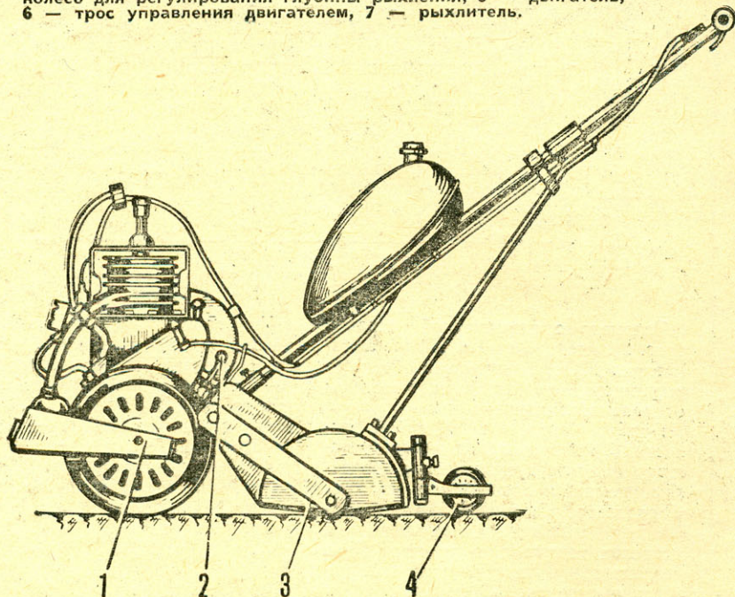
Р и с. 2. Проекции моторобота «Юннат»: 1 — рама, 2 — рычаг включения рыхлителя, 3 — ножух, 4 — колесо для регулирования глубины рыхления, 5 — двигатель, 6 — трос управления двигателем, 7 — рыхлитель.
