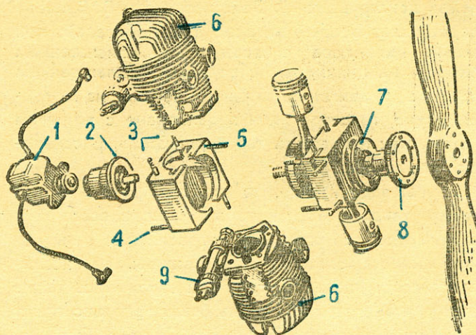
Рис. 5. Двухцилиндровый двигатель ББ-1 конструкции Г. Белошапкина и Б. Буянова в разобранном виде: 1 — магнето КАТЭК, 2 — станан крепления магнето, 3 — болты крепления цилиндров к картеру, 4 — болты крепления к подмоторной раме, 5 — болты крепления половинок картера, 6 — цилиндры ИЖ-56 с головками, 7 — шкив привода тахогенератора, 8 — фланец крепления воздушного винта, 9 — карбюратор.
