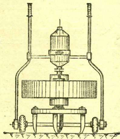
Р и с. 1. Электрорыхлитель: 1 — редуктор, 2 — диски, 3 — электродвигатель, 4 — ручка, 5 — колесо, 6 — рабочий орган.
