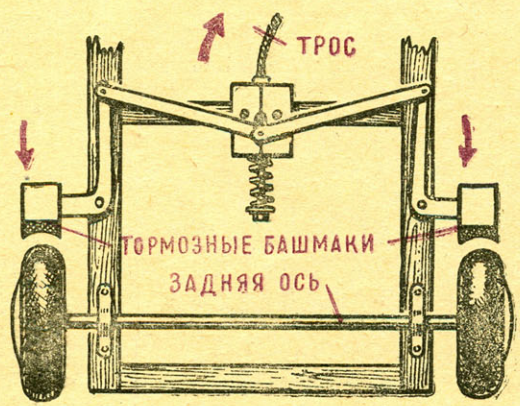
Рис. 3. Тормозное устройство.
