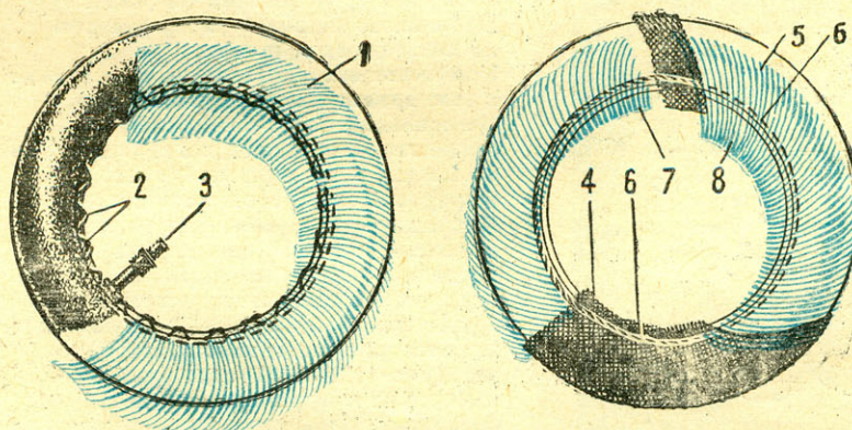
Рис. 3. Порядок сборки покрышки. 1 — участок с уложенным первым слоем, 2 — сшитые края покрышки, 3 — вентиль, 4 — прослойка из сырой резины (толщина = 0,5 мм), 5 — второй слой корда, 6 — бортовое кольцо, 7 — завернутые наружу концы корда, 8 — завертываемые внутрь края корда.
