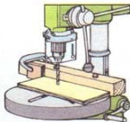
2 Воспользуйтесь упором с концевым ограничителем для изготовления одинаковых деталей
