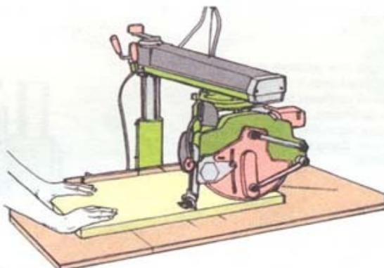
Поставьте полотно во внешнее (дальнее) положение по отношению к стойке станка, чтобы пилить широкую доску или панель
