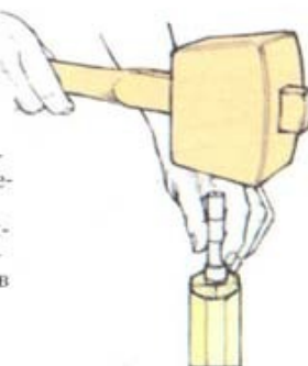
5 Вбейте приводной центр в заготовку
