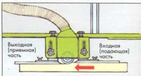
2 Выдвиньте выходную половину упора вперед, чтобы она служила опорой для уже срезанного (полностью) отрезка кромки.
