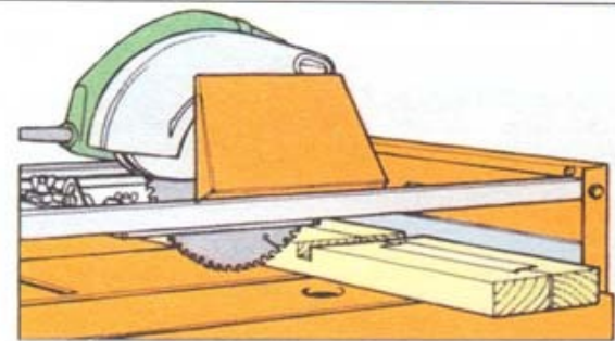
Поднимите пилу при выполнении паза для врубки
