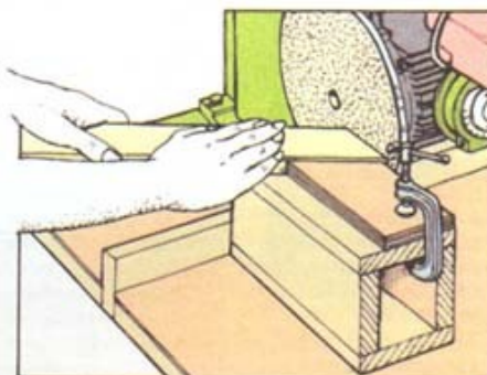
Для аккуратного шлифования диском используйте упор
