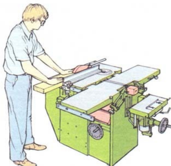
Продольное пиление в режиме отрезного станка
