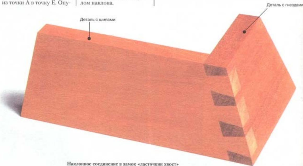
Наклонное соединение в замок «ласточкин хвост»
