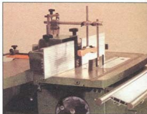
Универсальный станок в режиме фасонно-фрезерного станка
