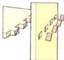
1 Диагональные клинья
