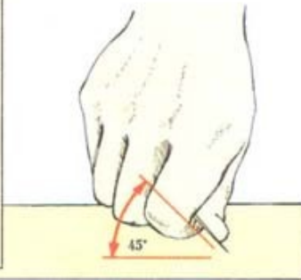
Держите режущий нож-косячок с постоянным углом наклона
