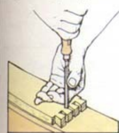
7 Срежьте остаток щепы
