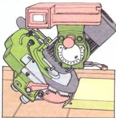
Сделайте прорез для усиленного углового соединения со скосом
