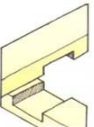
Поперечное соединение вполдерева
