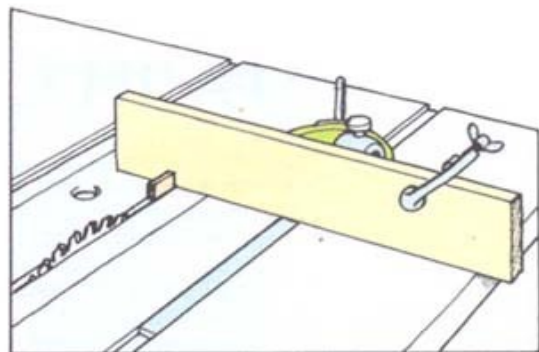
2 Приклейте в пропиле шип
