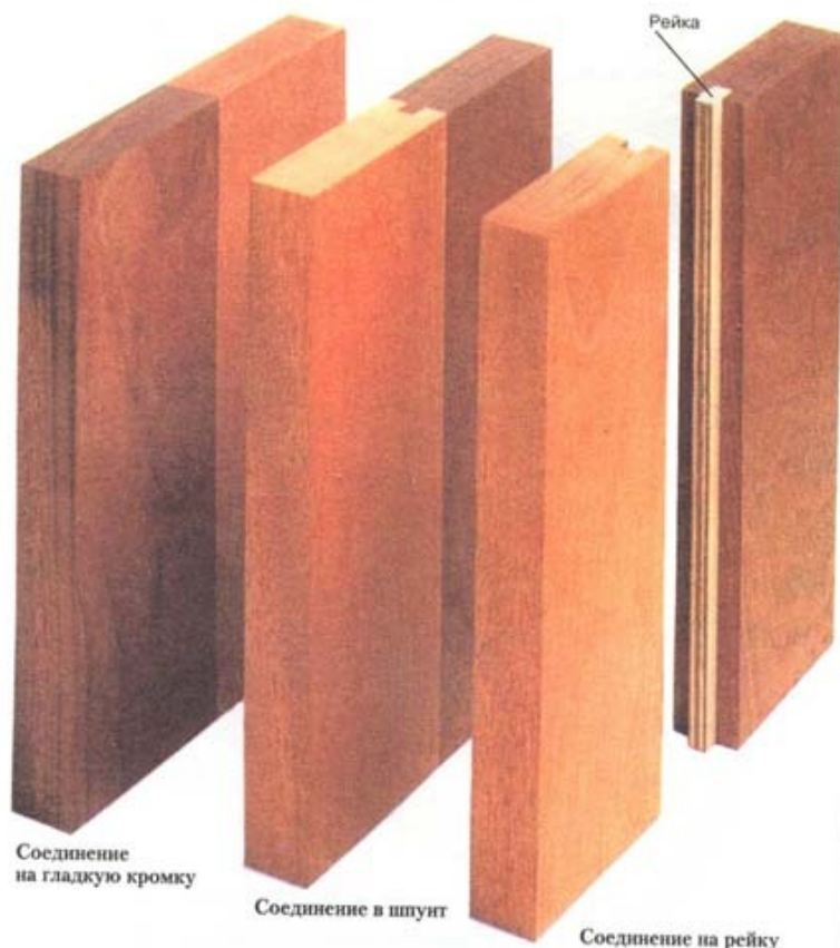
Соединение на рейку
