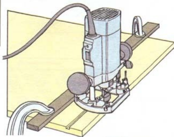
1 Вырезание паза с помощью направляющей рейки
