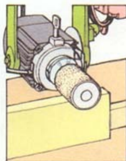
Шлифование прямой кромки Устанавливайте барабан горизонтально.
