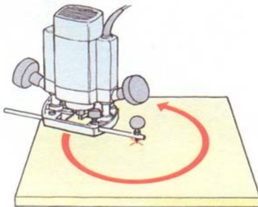
Вырезание кругового паза с помощью эллипсографа
