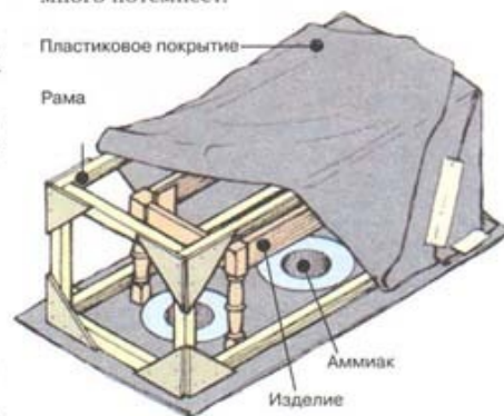
Самодельный испарительный шкаф
