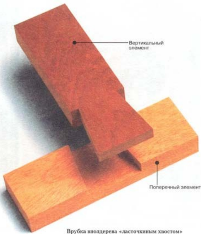
Врубка вполдерева «ласточкин хвостом»
