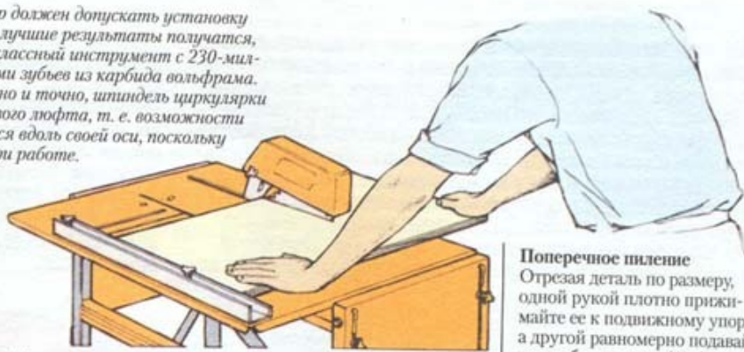
1 Распиловка широкой панели
