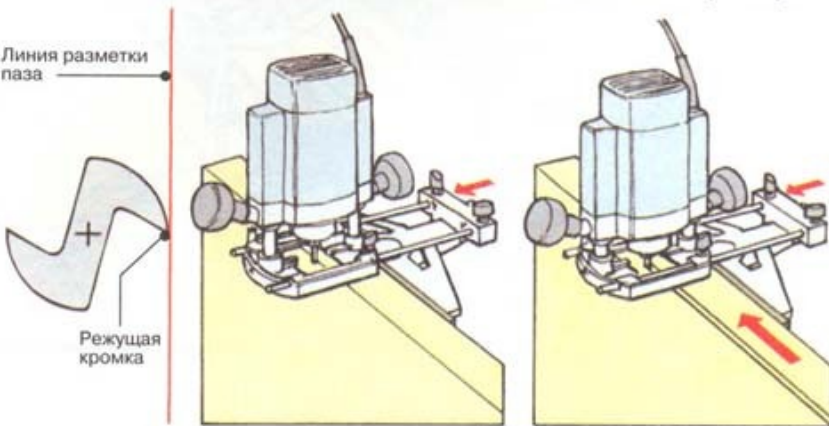
1 Выровняйте фрезу
