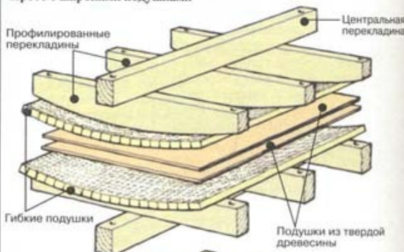
Пресс с изогнутыми подушками
