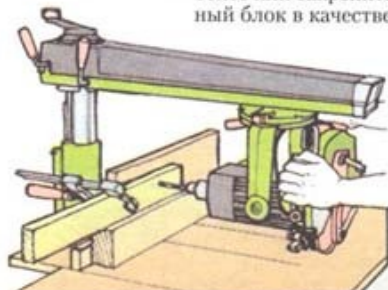
1 Подавайте сверло на боковую грань
