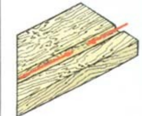
6 Меняйте направление резания в соответствии с расположением волокон
