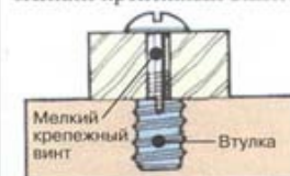
Резьбовая втулка под винт
