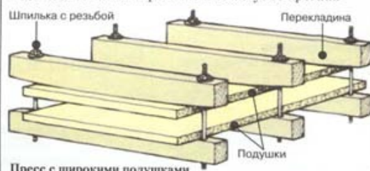
Пресс с широкими подушками
