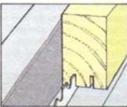
1 Вырежьте каждую сторону гребня
