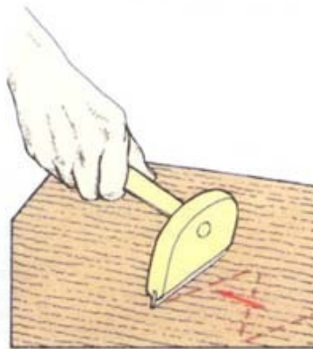
5 Придавите фанероальным молотком
