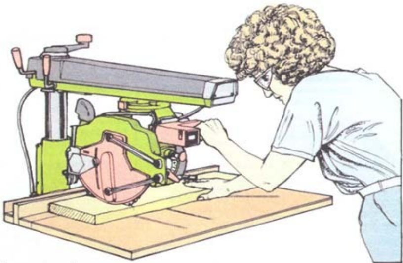
Плотно прижимайте заготовку к упору во время отрезания под прямым углом
