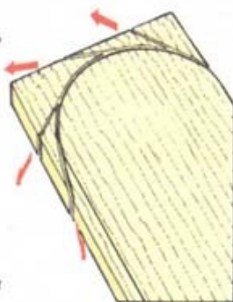
2 Вырезание крутого изгиба Удаляйте обрезки частями.
