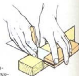
1 Разметьте линию заплечиков
