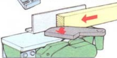
Некоторые ограждения сдвигаются в сторону самой заготовки
