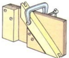
Выпиливание прорезей в детали рамы со скосом
