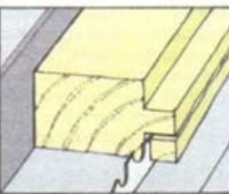
2 Затем удалите обрезок
