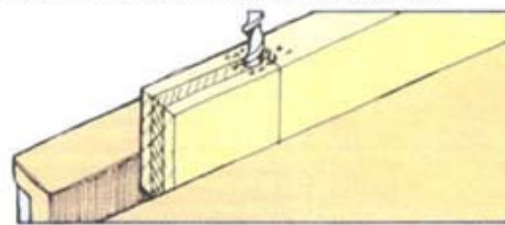
2 Просверлите отверстие рядом с линией заплечиков
