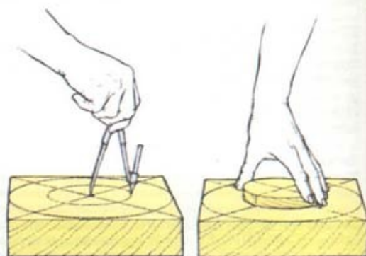
1 Циркулем начертите дно заготовки
