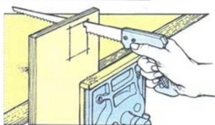
Работа выкружной пилой
