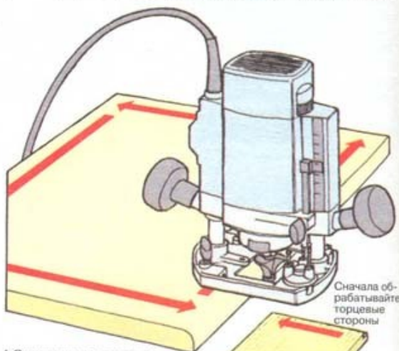
1 Округление края искусственной панели
