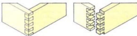
1 Сделайте ровные прямоугольные торцы
