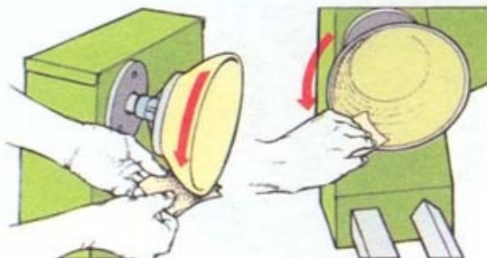
1 Шлифование внешней поверхности
