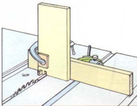
5 Наденьте гнездо (паз) на шип шаблона и сделайте второй пропил
