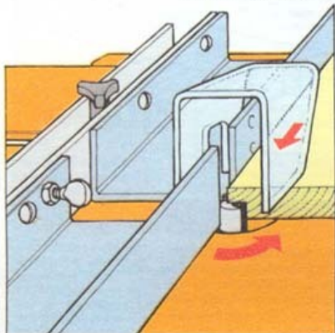
Обрабатывающий центр в строгально-калевоочном варианте
