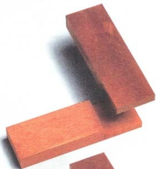
Угловое соединение вполдерева
