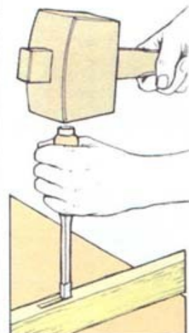
5 Вырубайте отход до ленты-индикатора
