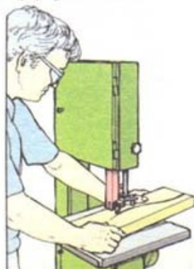
1 Свободный режим пиления «от руки» Ведите заготовку двумя руками.
