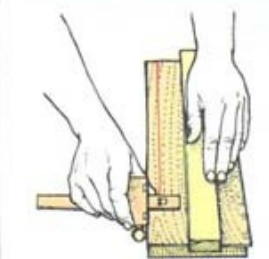
3 Постучите для уменьшения размера
