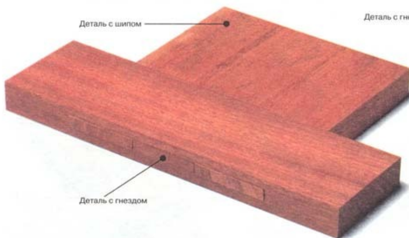
Соединение на парный шип
