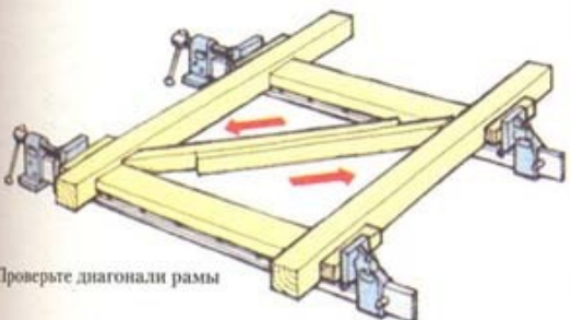
3 Выровняйте струбцины и элементы рамы
