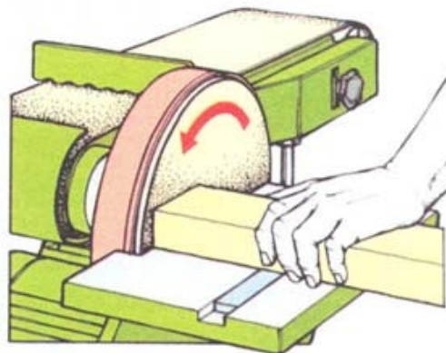
Шлифуйте торцы на части диска, двигающейся вниз.
