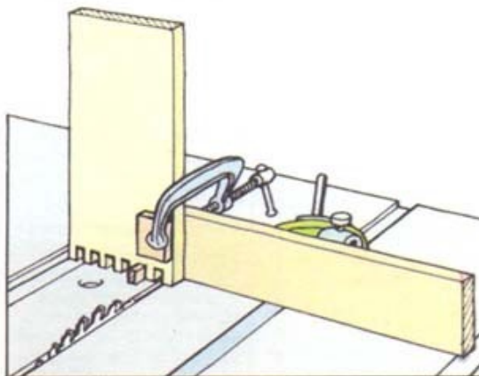
6 Выполните ряд шипов до конца заготовки
