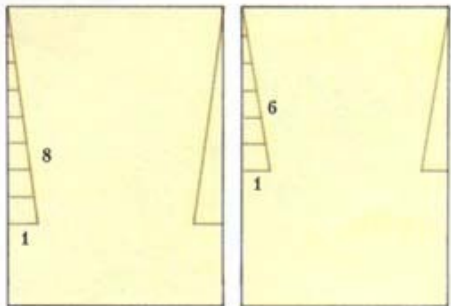
Уклон для твердых пород
