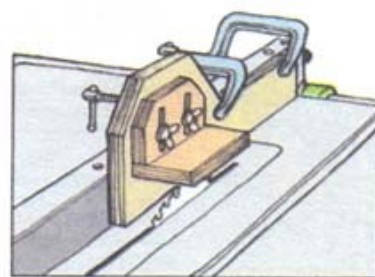
Самодельное ограждение – другой вариант защитного устройства
