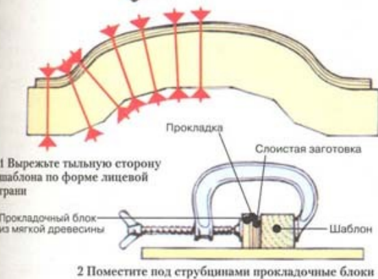
Шаблон из массива
