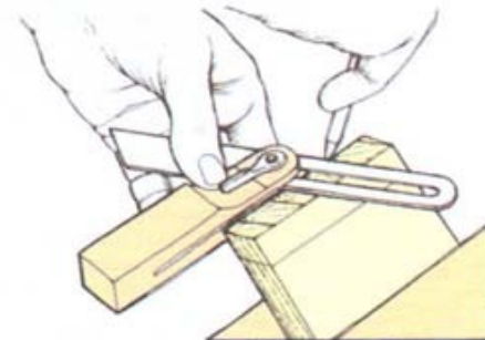
9 Держите колодку малки ровно по отношению к торцевой грани
