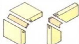
2 Пользуйтесь двумя разделительными брусками при выполнении поперечного соединения вполдерева
