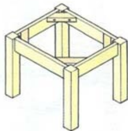
Прочные соединения и угловые блоки жестко закрепляют раму
