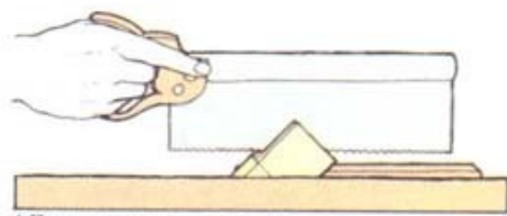
1 Пилите вдоль линии разметки шипа
