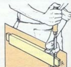
Работа стамеской с внутренней кромкой Эта стамеска обтачивает заплечики
