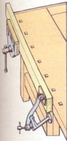
Использование зажима для фиксации длинной заготовки
