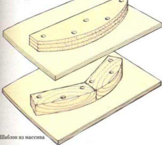
Шаблон из ДСП
