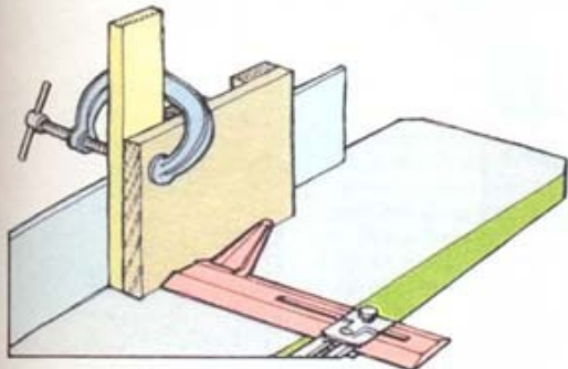
Закрепите заготовку на шаблоне перед строганием торца
