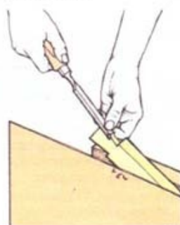
2 Срежьте отход
