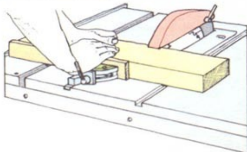
Производите поперечное пиление, перемещая упор
