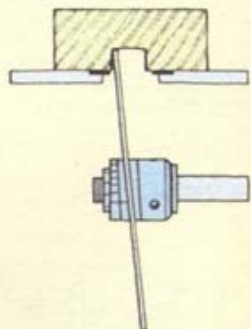
Сборка с качающими шайбами
