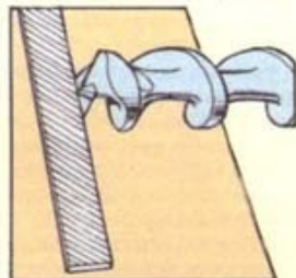
Заточите каждый зубец маленьким напильником, или надфилем
