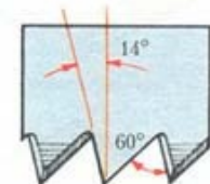
2 Зубья для поперечного пиления
