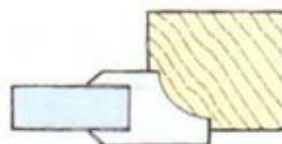
2 Обработка кромки из нижнего положения (снизу заготовки)
