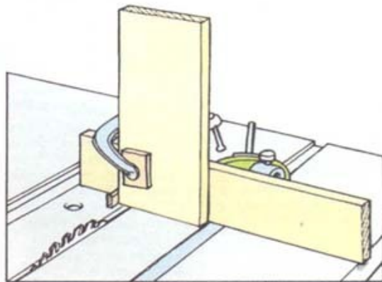
4 Прижмите заготовку к шипу шаблона
