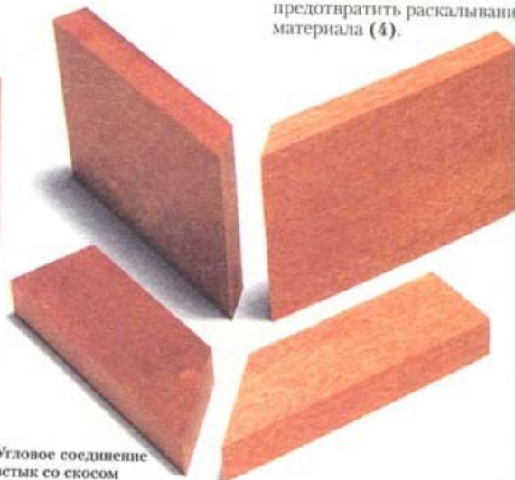
Усушка может привести к появлению щели внутри углового соединения
