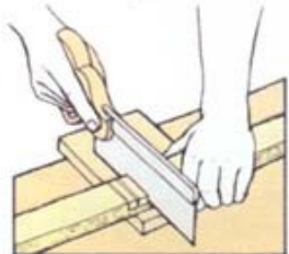
4 Сделайте пропилы в отходе
