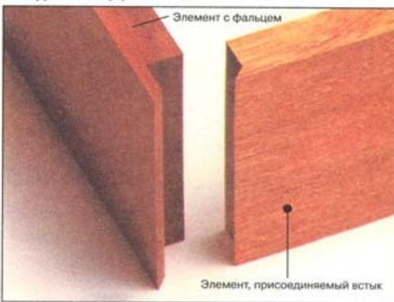
Соединение внахлест со скосом
