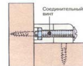
Колодочное соединение в собранном виде
