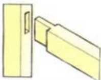
Гнездо и шпих
