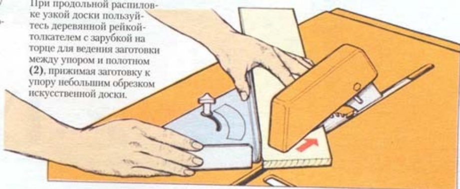
2 Выполнение детали для углового соединения со скосом
