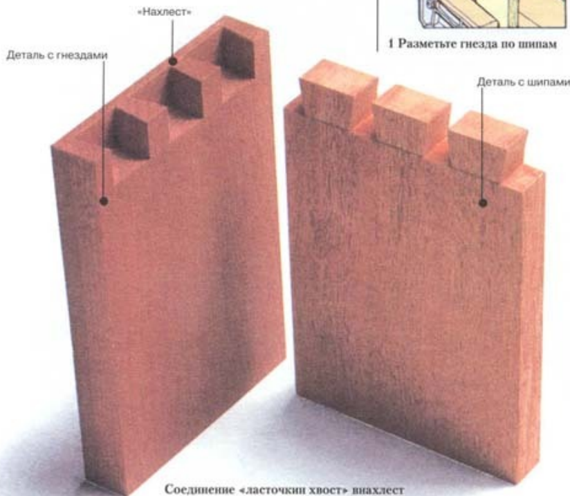
Соединение «ласточкин хвост» внахлест
