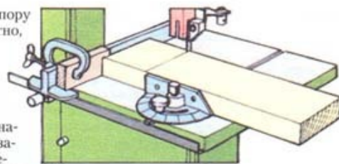
1 Отпиливание одинаковых отрезков
