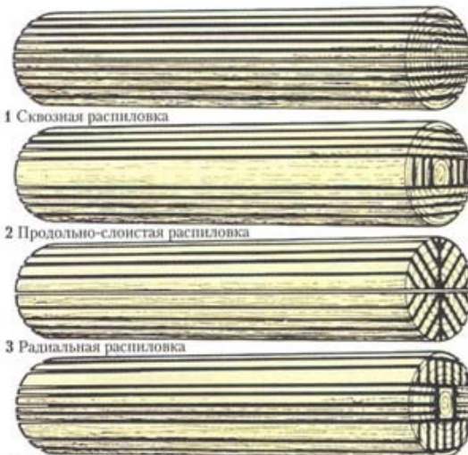
4 Поперечно-слоистая распиловка
