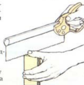
3 Сделайте узкие пропилы
