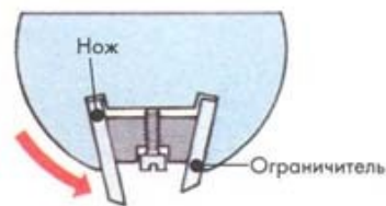
2 В качестве альтернативы перед ножом устанавливается ограничитель
