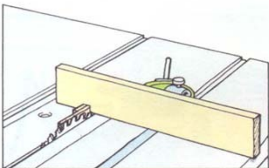
3 Поместите планку между шипом и полотном
