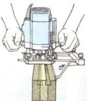
Выполнение центрального паза
