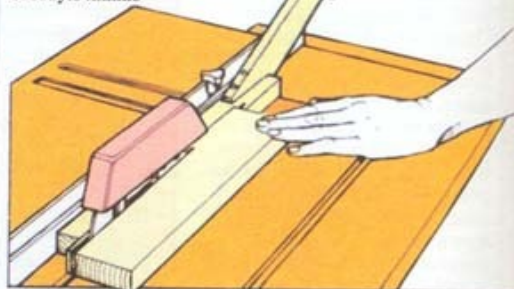
2 Сделайте направляющий брусок с концевым упором для подачи заготовки
