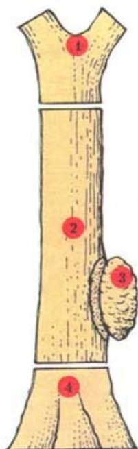
Части дерева, используемые для изготовления шпона 1 Разветвление 2 Ствол 3 Кап, или наплыв 4 Комель, или пенёк
