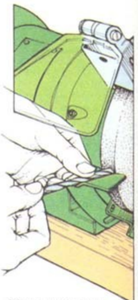
3 Заточка спирального сверла
