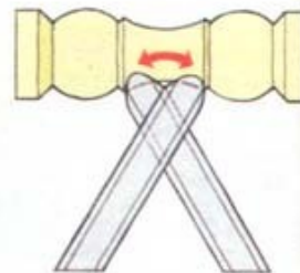
1 Снимите полукруглым резцом часть материала между валиками
