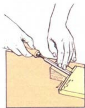
3 Срезайте скос «ласточкина хвоста»
