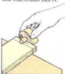
1 Разметьте заплечики малых шипов
