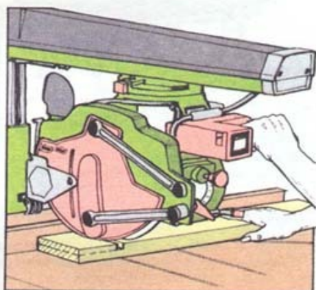
Сначала вырезайте заплечик соединения вполдерева, а потом выбирайте отход
