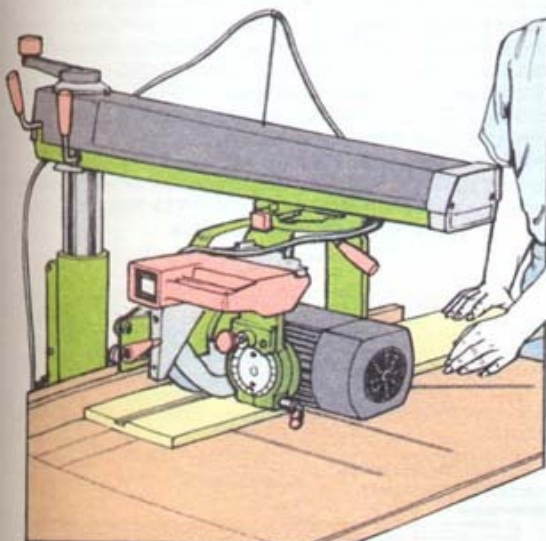
Головка для пазов вырезает широкий паз за один проход
