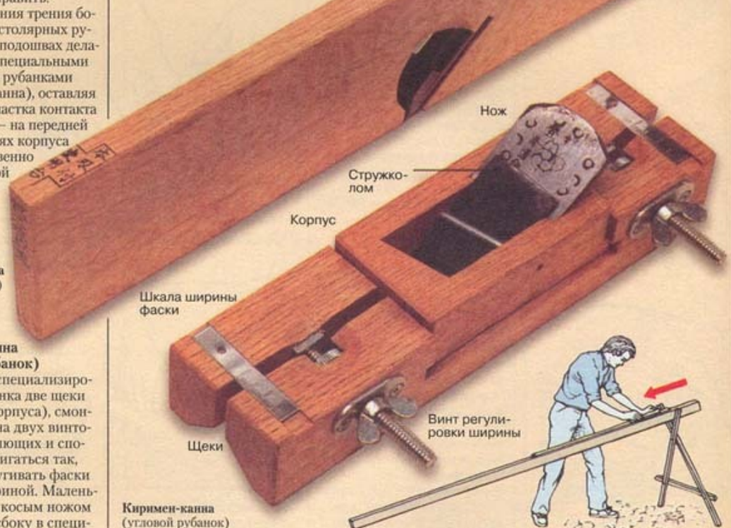
Канна (столярный рубанок)
