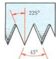
4 Универсальные зубья
