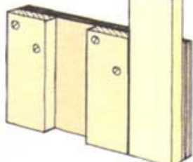
2 Оставьте место для заготовки
