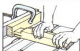
5 Вырежьте запяточники
