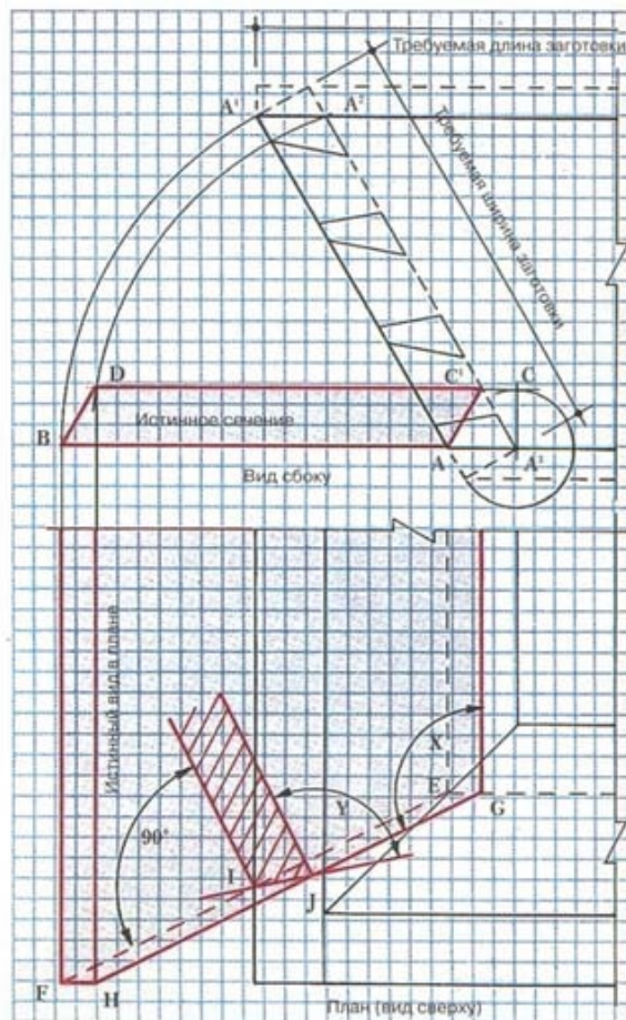
1 Сделайте чертеж проекций и истинного вида соединения
