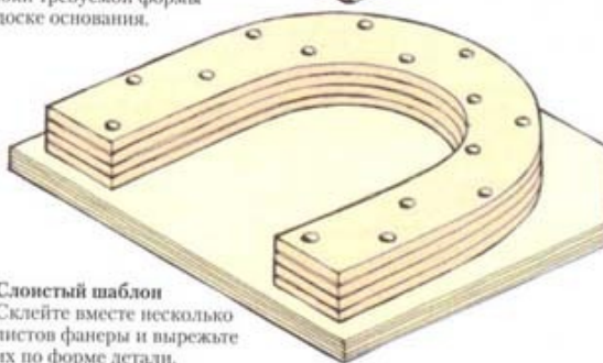
Шаблон из массива Приклейте и приверните шурупами цельнодеревянные блоки требуемой формы к доске основания.
