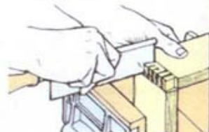
5 Наметьте гнезда (перегородки) наградкой
