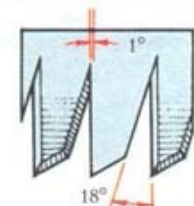
3 Японские зубья
