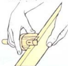
3 Разметьте рейсмусом линии на кромках
