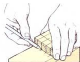
3 Отметьте линии шипов
