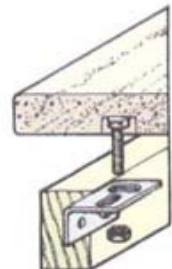
2 Металлический кронштейн
