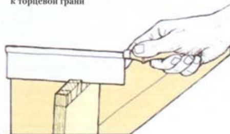
10 Установите линии пиления вертикально
