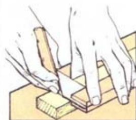
2 Разметьте линии заплечиков
