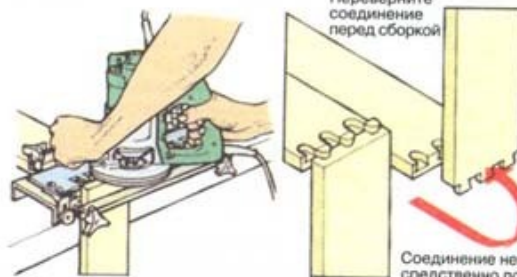
2 Фрезеруйте соединение
