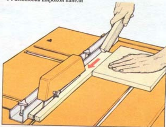
2 Продольное пиление узкой заготовки
