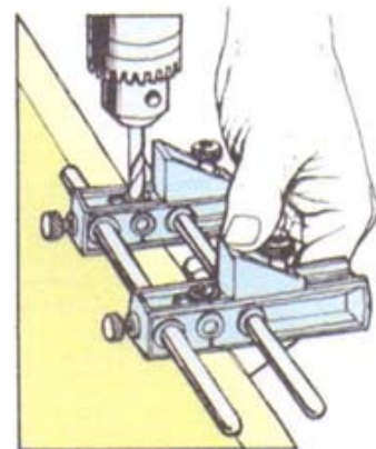
Нагельный кондуктор
