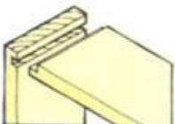
Односторонняя врубка
