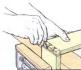
1 Разметьте гнезда по шипам
