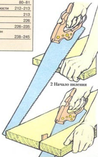
3 Держите пропил открытым с помощью клина
