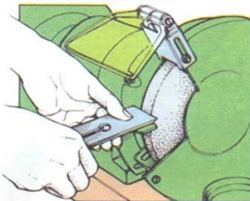
2 Заточка кромки ножа
