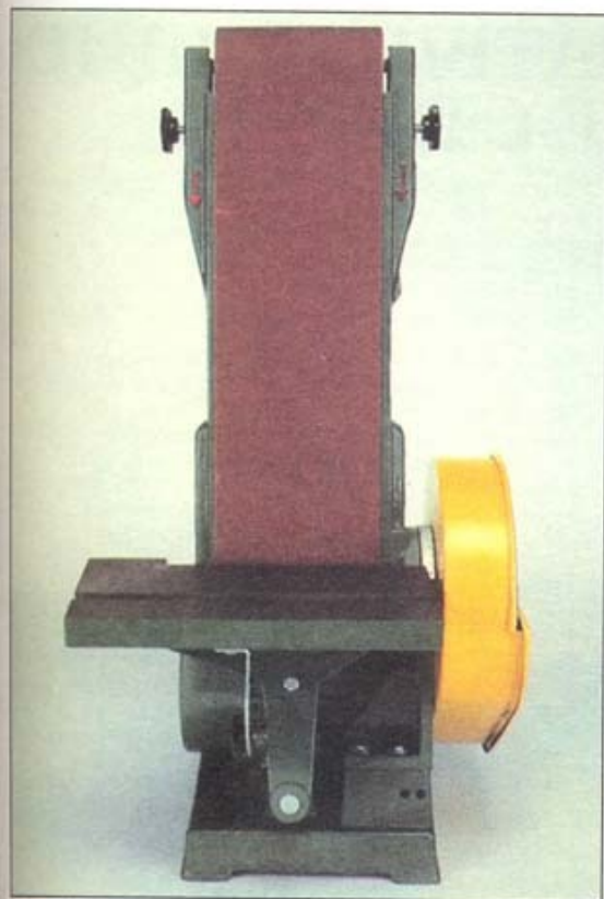
Ленту можно поставить в вертикальное положение
