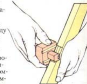
3 Рейсмусом прочертите линии разметки гнезда
