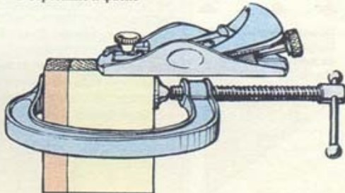
3 Укрепление края бруском
