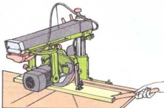
Пользуйтесь толкателем при продольном пиленнии узких заготовок
