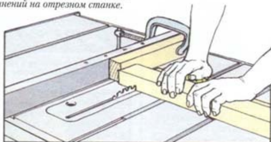
1 Выполнение углового соединения вполдерева
