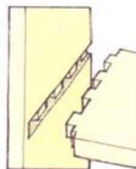
2 Комбинация с непроходной врубкой
