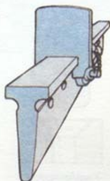
Тавровое сечение реечной струбцины
