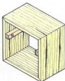
3 Поперечные рейки сдерживают усыхание, пока трещины не снимут напряжение в материале
