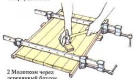
1 Установите струбцины сверху деланки
