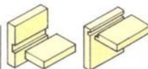
Проходной паз для врубки Угловая врубка заподлицо
