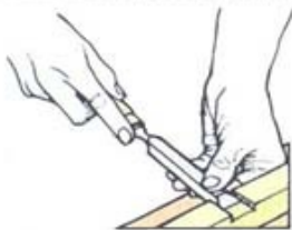
1 Придание стамеске устойчивости
