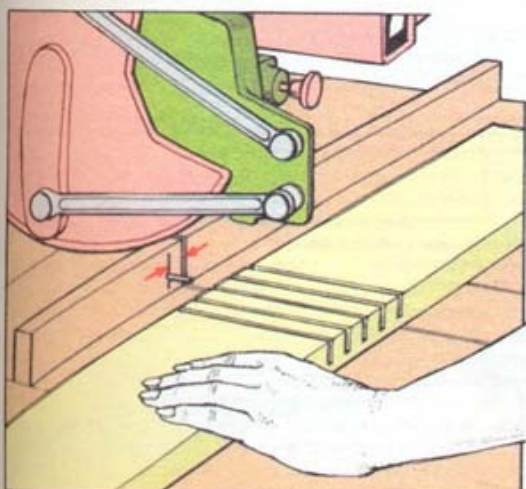
Используйте гвоздь без головки для обеспечения равномерного расположения пропилов для изгиба
