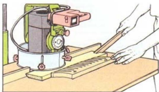
Обработка кромки узкой доски Пользуйтесь прижимной гребенкой, чтобы удерживать заготовку, прижатой к упору.
