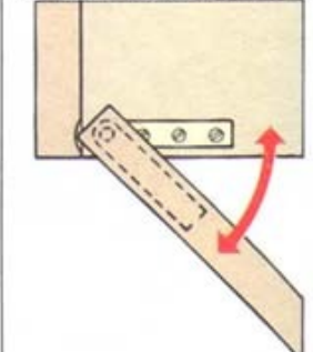
Дверца на боковой петле открыта
