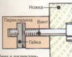
Винт с цилиндрической поперечной гайкой
