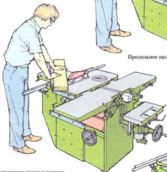
Выполнение скоса в режиме отрезного станка
