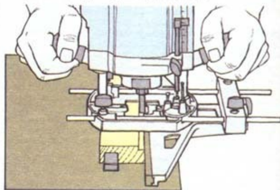
Изготовление фальца прямой фрезой с помощью линейки
