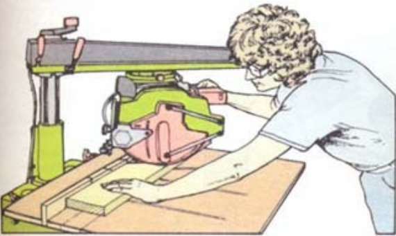
Выполняйте скос, придерживая заготовку одной рукой
