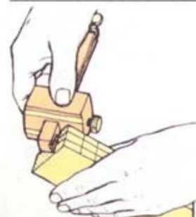
5 Разметьте рейсмусом кромку и торец
