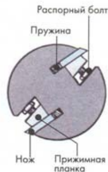
Типовой ножевой блок поперечно-строгального станка
