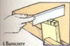
4 Выпилите боковые грани шипов
