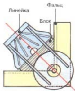
2 Центровка треугольного блока по центру фрезы
