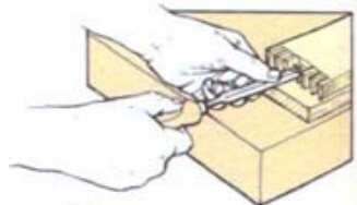
7 Срежьте излишек
