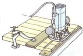
2 Зафиксируйте их упорной рейкой
