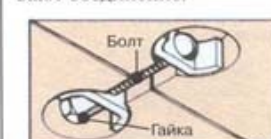
Панельная стяжка
