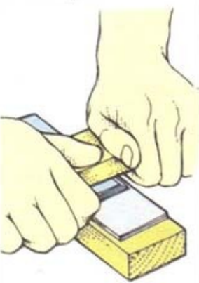
Выравнивание полотна Точите тыльную сторону полотна, оказывая на него нажим через деревянный брусок.
