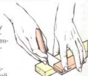
1 Прочертите линии разметки заплечиков
