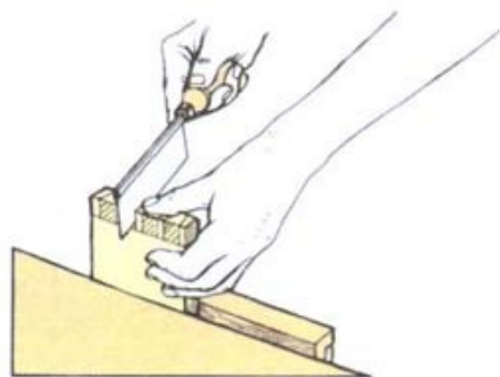
11 Выпилите боковые грани гнезд
