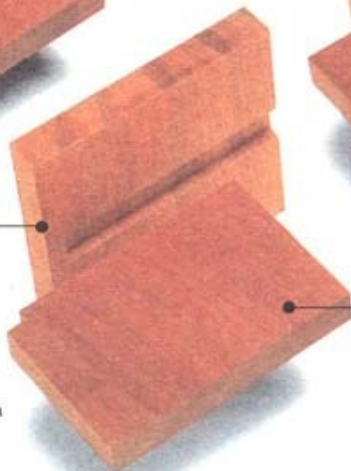
Непроходная врубка
