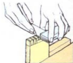
3 Разметьте концы шипов
