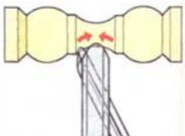
3 При вытачивании желобка ведите полукруглый резец от края вниз к центру
