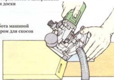
3 Выборка пазов в центральной части доски
