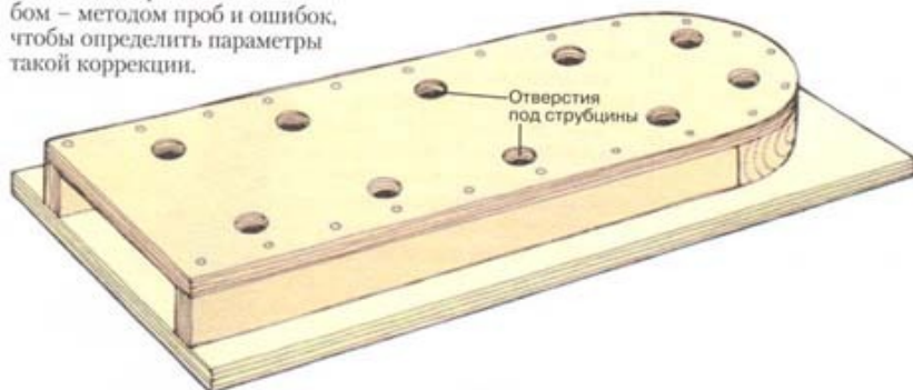
Слоистый шаблон Склейте вместе несколько листов фанеры и вырежьте их по форме детали.
