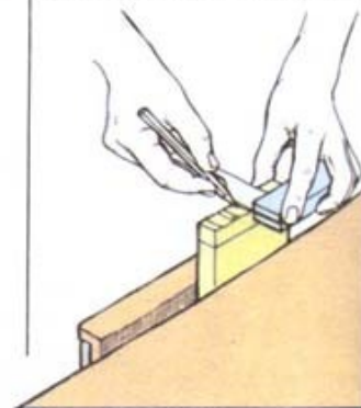
3 Разметьте концы шипов
