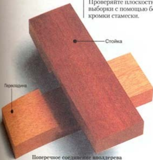
Поперечное соединение вполдерева
