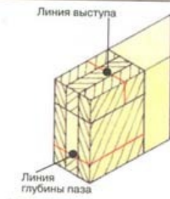
1 Разметьте линии резания
