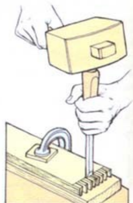
6 Прорежьте поперек волокон
