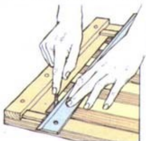
2 Подровняйте края полос
