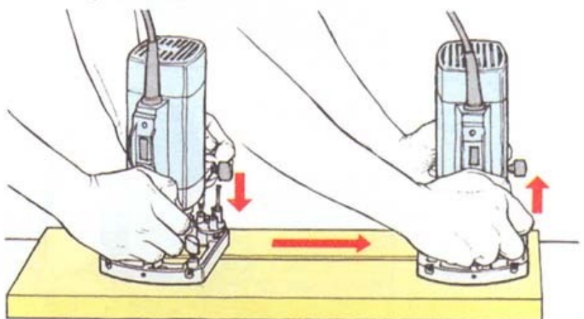
1 Опустите на максимальную глубину
