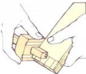
2 Рейсмусом разметьте шипы
