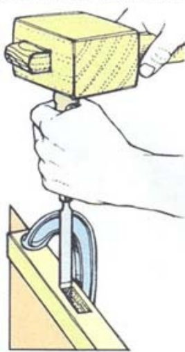
Легкие удары боковой стороной для киянки
