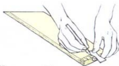
2 Разметьте шипы
