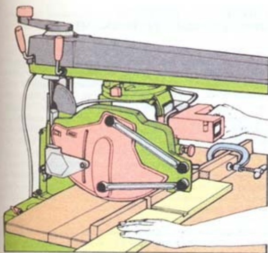
Пользуйтесь концевым ограничителем, чтобы правильно расположить паз для врубки
