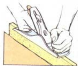
1 Фуганком или длинным рубанком выровняйте кромку
