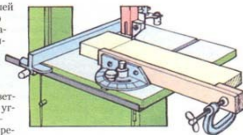
2 Отпиливание одинаковых по длине деталей
