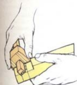
7 Рейсмусом разметьте толщину гнезда под клин
