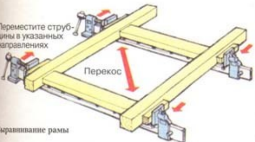
4 Проверьте диагонали рамы
