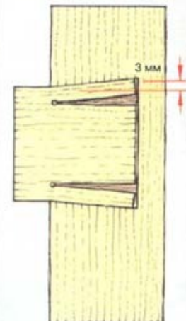
Расклинивание двойным клином. Потайные клинья распирают шип внутри гнезда и запирают его там.
