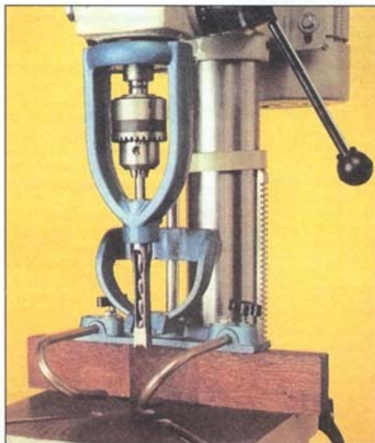
Долбежная насадка с полым долотом
