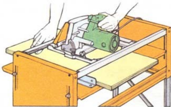
Распиловка широкой доски или панели Прижмите заготовку к упору и равномерно ведите пилу.
