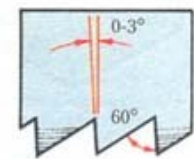
1 Зубья для продольного пиления
