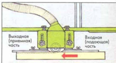
1 Если часть кромки изделия остается нетронутой при обработке, обе половины упора ставьте по одной линии
