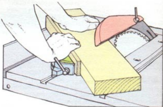
2 Наклоните полотно для сложного скоса
