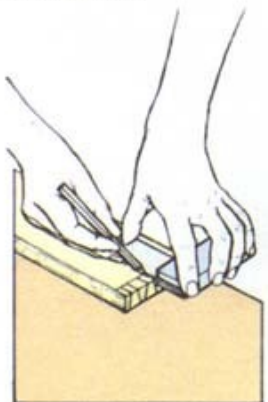
10 Разметьте бока гнезд
