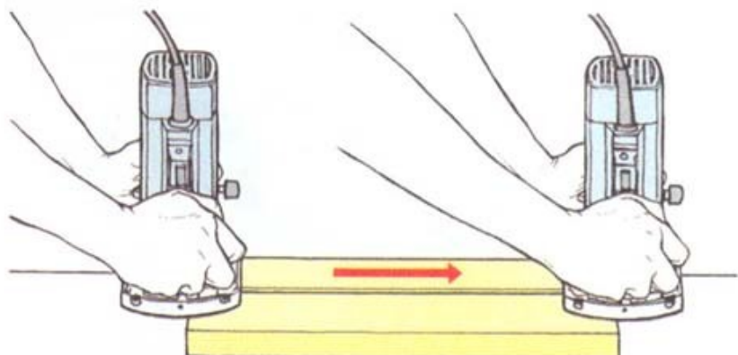
Выполните проходного паза
