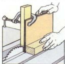
3 Выполните одну грань шипа
