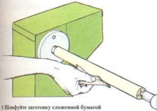
1 Шлифуйте заготовку сложенной бумагой
