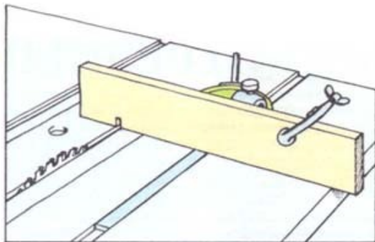
1 Сделайте пропил в шаблоне
