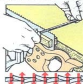
5 Заточка зубьев продольной пилы
