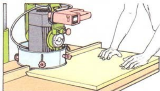
1 Обработка кромки из верхнего положения (сверху заготовки)
