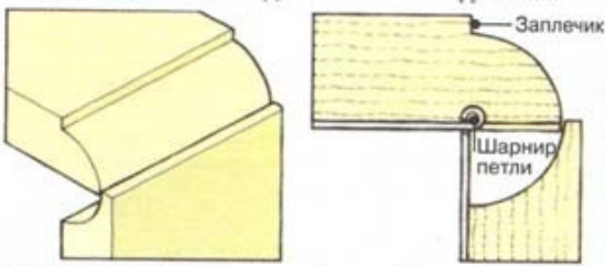
Выровняйте шарнир петли с заплечиком
