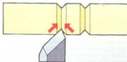
1 Выточите V-образные желобки с каждой стороны валика
