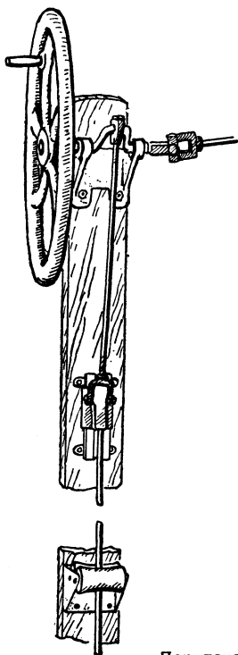
Передающий механизм к насосу.
