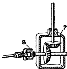
Схема передачи от ветроколеса к насосу:
