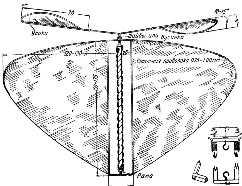
Фиг. 20а. Общий вид «бабочки».
