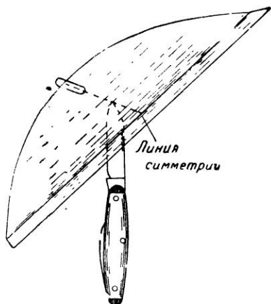
Фиг. 28. Определение центра тяжести модели.
