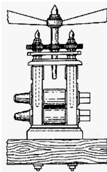
Система валов для плющения цанов; верхним рычагом регулируется расстояние между валами, зубчатыми колесами и шпинделями
