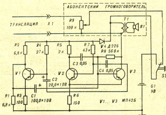
Рис. 1. Принципиальная схема звонка.
