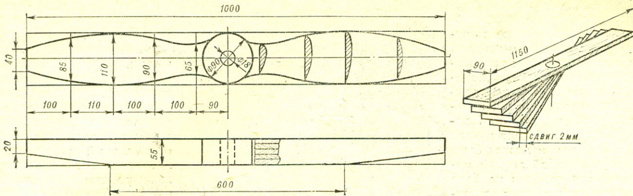
Рис. 3. Основные размеры воздушного винта.
