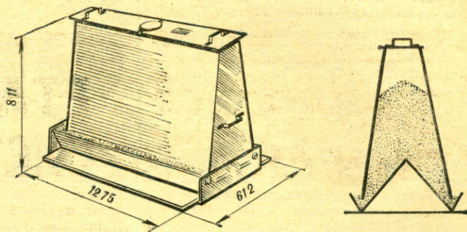
Рис. 7. Самокормушка для птицы и ее схема.
