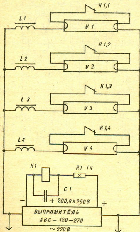
Принципиальная схема пускорегулирующего устройства на реле.
