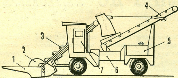
Рис. 1. Схема переоборудованного погрузчика: 1 — самоподающий лоток, 2 — винтовой шнек, 3 — ковшый элеватор, 4 — ленточный транспортер, 5 — двигатель, 6 — топливный бак, 7 — кабина.
