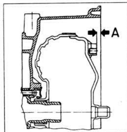
5.29 Схема установки гидротрансформатора А = 9 - 10 мм
