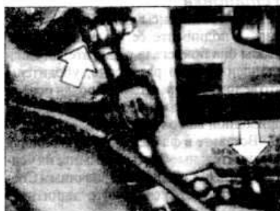
5.17 Отверстие регулировки и стяжной болт - отмечены стрелками
