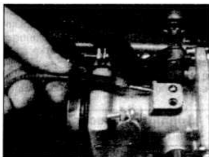
11.2 Отсоедините вакуумный шланг распределителя от кожуха дроссельной заслонки
