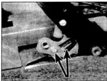
18.1 Месторасположение выключателя контрольной лампы ручного тормоза и болт крепления (отмечен стрелкой)
