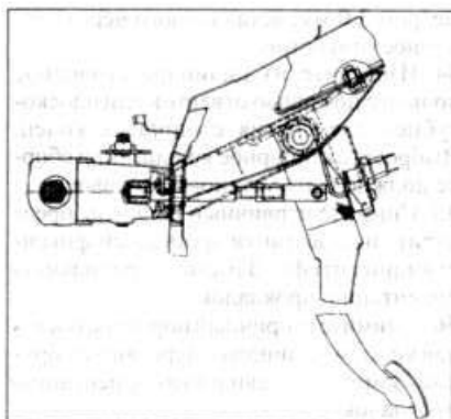
13.37 Схема установки тормозной педали - ранние модели. Стрелкой отмечен резиновый ограничитель
