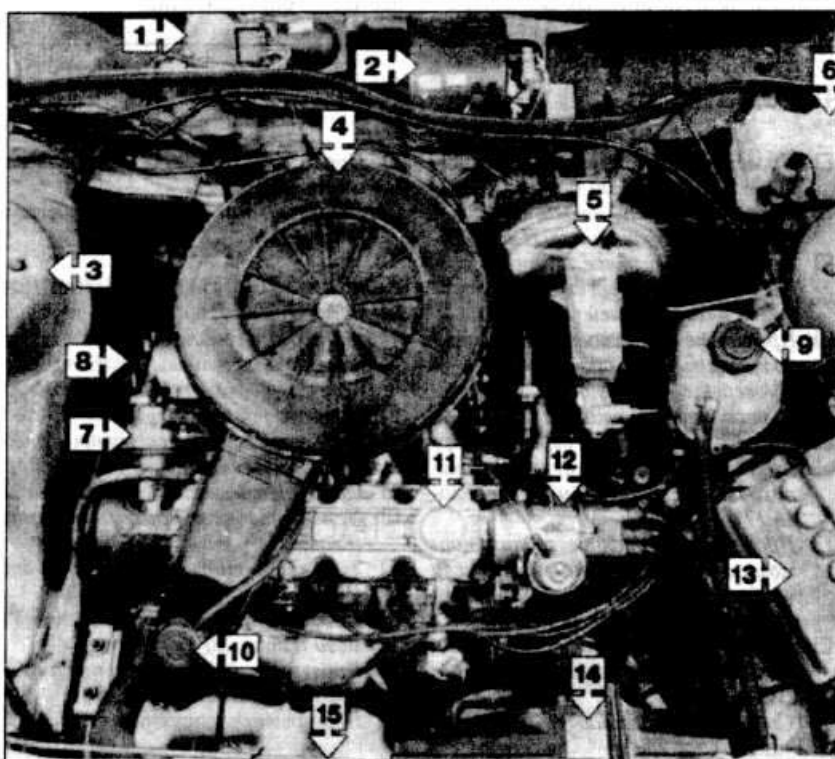
Вид моторного отсека - модели 1.3 л
