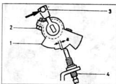
14.14 Карбюратор Pierburg: регулировка кулачка повышенной частоты холостого хода
