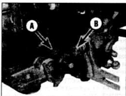
10.3a Ограничитель дросселя (А) и винт регулировки частоты холостого хода (В) - карбюратор GM Varajet
