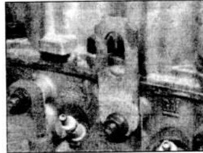
34.61b Расположение подъемной скобы двигателя на стойке выпускного коллектора
