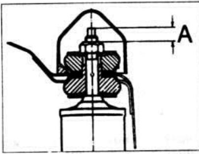
12.12a Верхнее крепление заднего амортизатора - стандартный тип A = 9 мм
