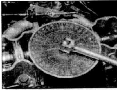
8.26б Использование углового указателя крутящего момента
