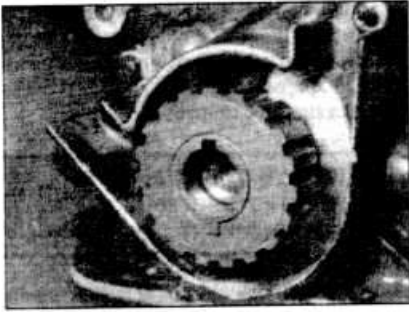
34.57 Звездочка коленвала
