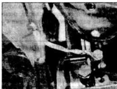
19.17 Ремень заземления двигателя к днищу
