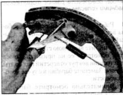
5.31а Установка рычага регулятора (Универсал)
