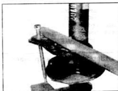
4.9a Метод откручивания поджимной гайки набивного сальника стойки
