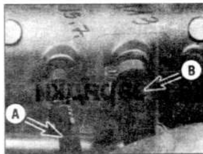
12.2 Отсоедините шланг усилителя тормоза (А) и шланг дополнительного воздуха (В)
