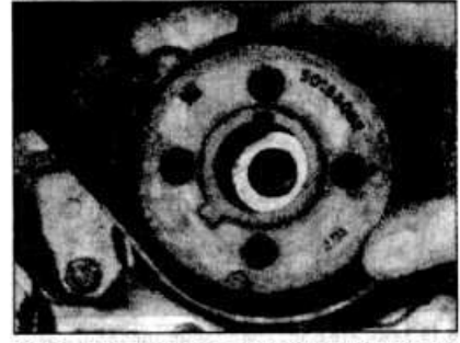
6.12b... затем снимите звездочку с коленвала
