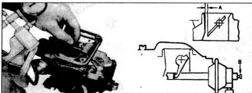
13.29 Проверка зазора между пластиной клапана и карбюратором
