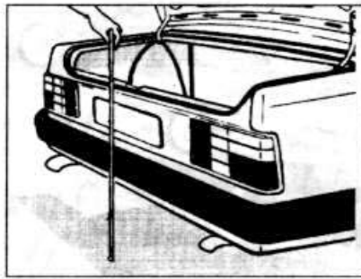
19.2 Измерение уровня задней подвески
