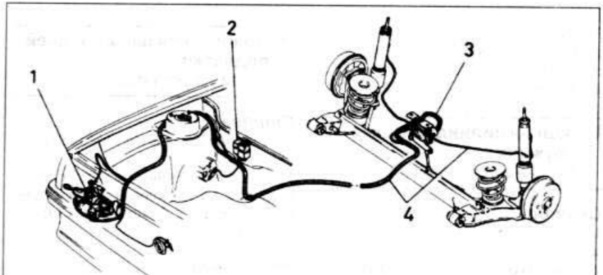
18.4 Компоненты автоматической системы управления уровнем
