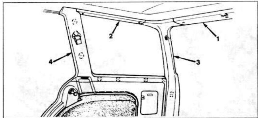
28.3 Панели отделки багажного отделения (Универсал)
