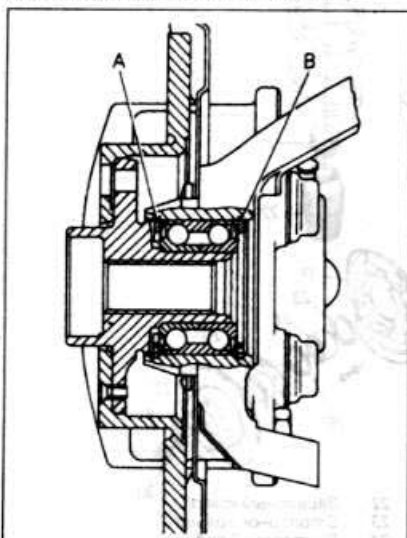
3.5a Передняя ступица в разрезе A и B - Стопорные кольца
