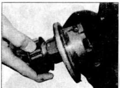
5.4a Снятие насоса системы охлаждения (ранние модели)
