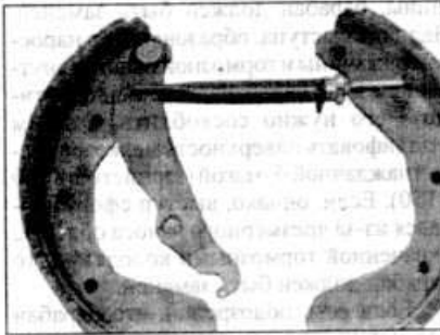
5.31д Правильно установленная саморегулирующаяся разжимная планка (Седан/Хэтчбек)
