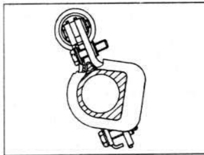
25.3b Положение зажима амортизатора относительно картера рулевого механизма
