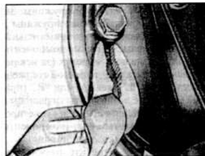
5.7 Сжатие пружины, удерживающей скобу - ранние модели
