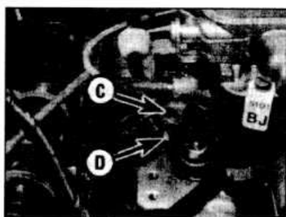
10.3b Дополнительные винты смеси (С) и (D) - карбюратор GM Varajet
