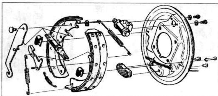
5.24b Вид компонентов саморегулирующегося заднего тормоза - поздний Универсал
