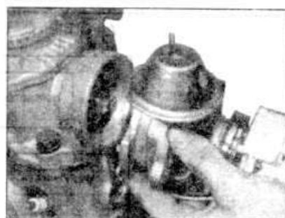
3.5 Снятие распределителя из кожуха распределителя
