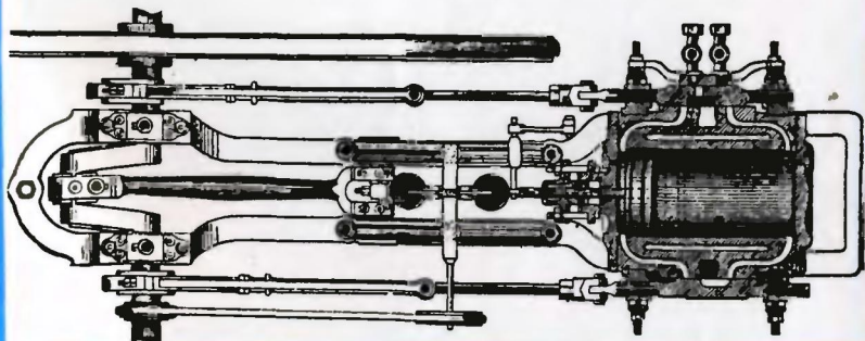
Двигатель Ленуара.
