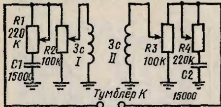
темброблок
