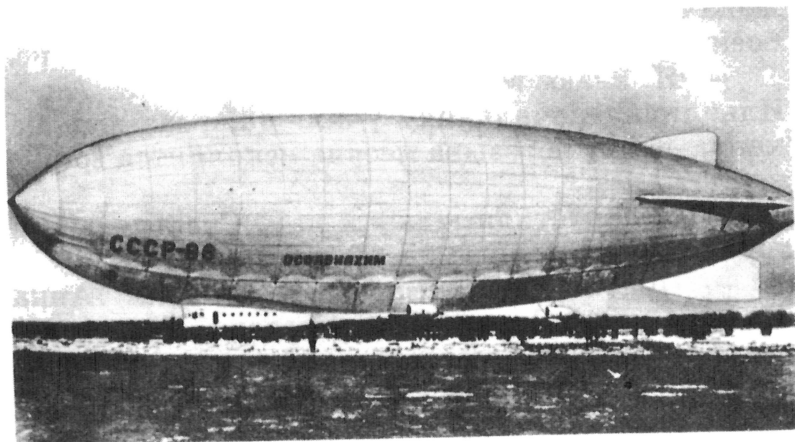
Дирижабль.
