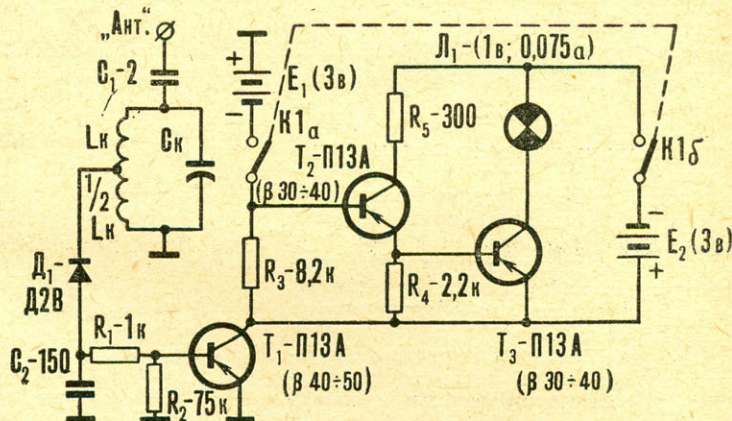
Р И С. 2. ИНДИКАТОР ИЗЛУЧЕНИЯ УКВ-ПЕРЕДАТЧИКА.
