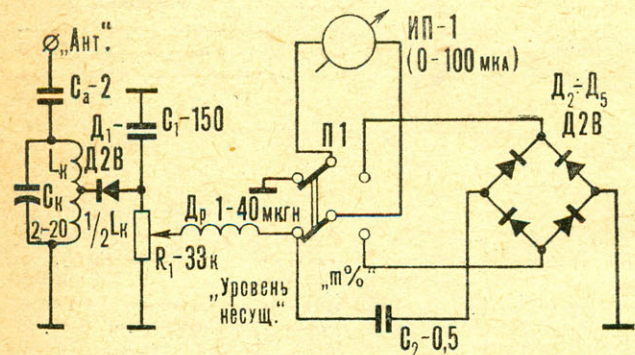
Р И С. 1. ИНДИКАТОР НАПРЯЖЕННОСТИ ПОЛЯ.
