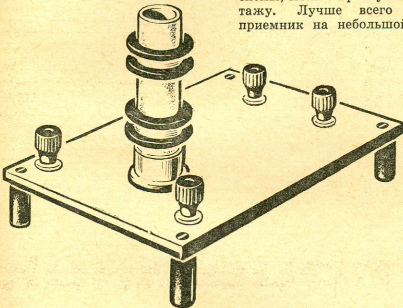
РИС. 3. КОНСТРУКЦИЯ ПРИЕМНИКА.
