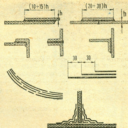
РИС. 4. ТИПЫ СОЕДИНЕНИЙ ПАНЕЛЕЙ.
