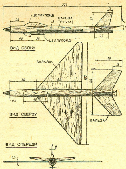
РИС. 3. МОДЕЛЬ ИСТРЕБИТЕЛЯ № 1.
