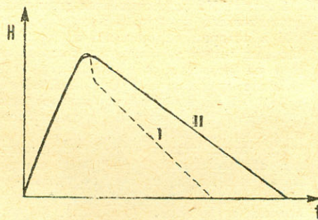
РИС. 2. ЗАВИСИМОСТЬ ВРЕМЕНИ ПОЛЕТА ОТ ВЫСОТЫ ПОДЪЕМА МОДЕЛИ: Н — высота полета; t — время полета; I — без автомата перебалансировки; II — с автоматом перебалансировки.
