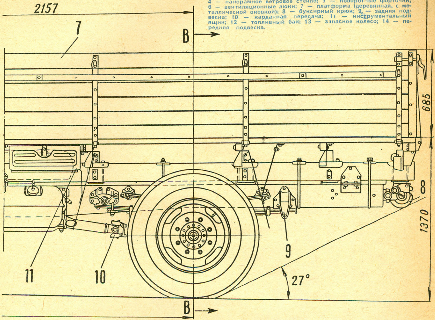
РИС. 1. АВТОМОБИЛЬ ЗИЛ-130 (ВИДЫ СВЕРХУ И СБОКУ. ВИД СПЕРЕДИ И СЕЧЕНИЯ ПО А-А, Б-Б, В-В ДАНЫ НА СТРАНИЦЕ 22).
