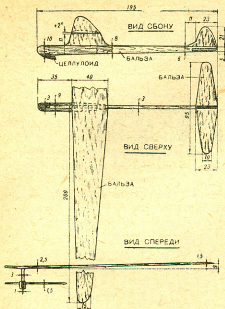
РИС. 2. МОДЕЛЬ ПЛАНЕРА.
