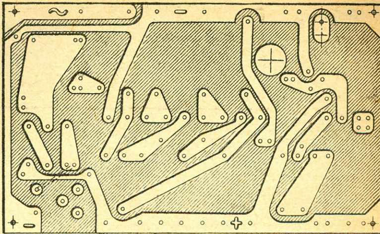
РИС. 2. ПЛАТА № 1.
