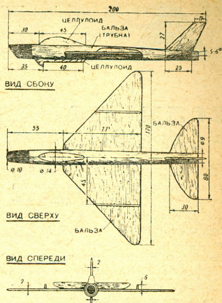
РИС. 4. МОДЕЛЬ ИСТРЕБИТЕЛЯ № 2.
