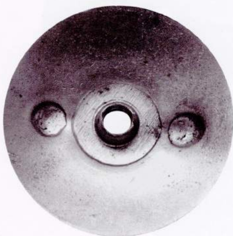
Гайка типа 4, варианта 1, разновидности 3 без конусообразного углубления с выпуклой стороны гайки и с круглым, кольцеобразным углублением большого диаметра вокруг ниппеля.
