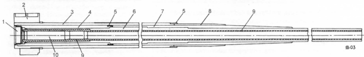
Ствол 406-мм орудия Mk-7: 1 — казенник; 2 — хомут; 3 — кожух; 4, 7, 8 — скрепляющие цилиндры; 5 — скрепляющие кольца; 6 — внутренняя труба; 9 — лейнер; 10 — зарядная камера.
