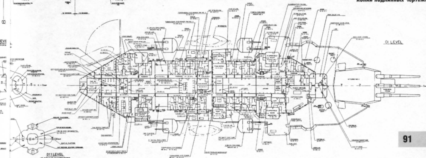
Линейный корабль ВВ-62 «Нью-Джерси», 1982 г. Копии подлинных чертежей
