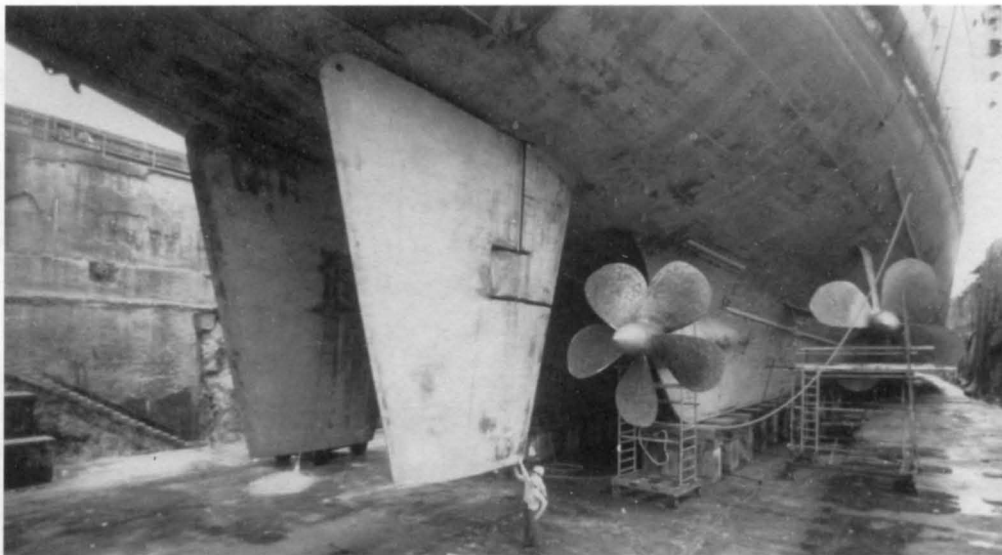
Винторулевая группа «Айовы»: двойные рули, пятилопастные внутренние винты и четырехлопастные внешние
