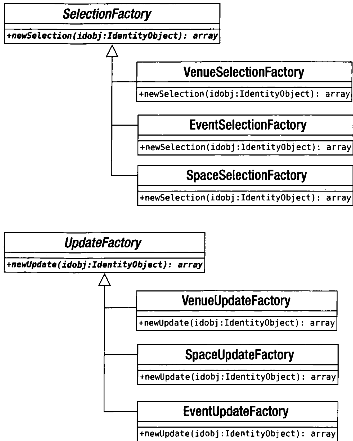
Рис. 13.10. Шаблоны Selection Factory и Update Factory
