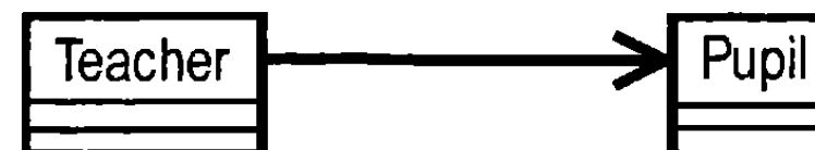
Рис. 6.10. Однонаправленная ассоциация
