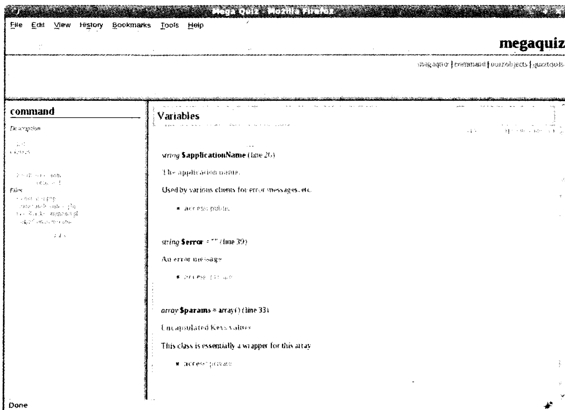
Рис. 16.5. Документирование свойств
