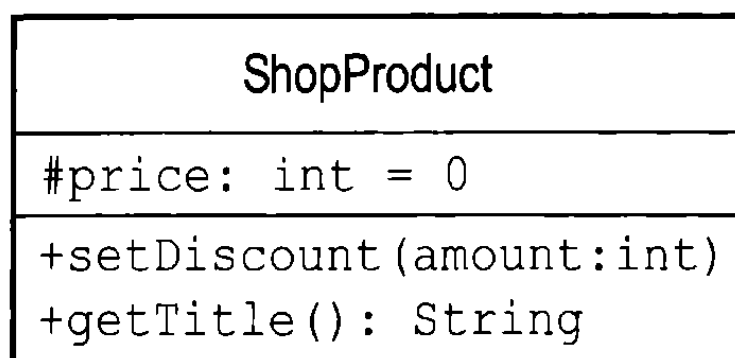
Рис. 6.6. Представление операций
