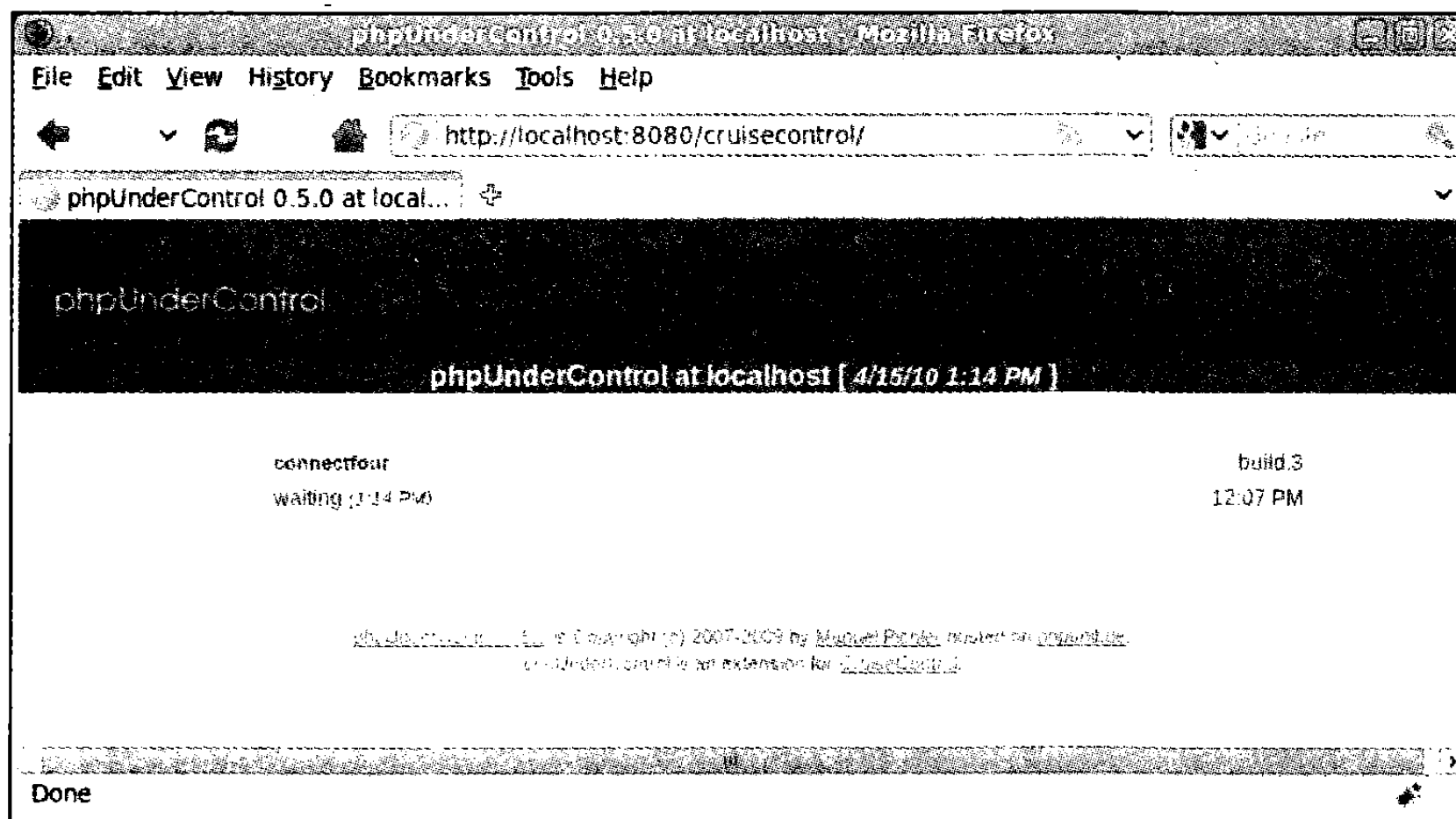
Рис. 20.5. Интерфейс phpUnderControl
