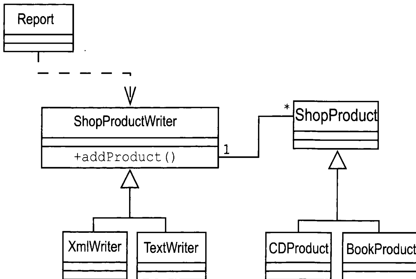
Рис. 6.16. Отношение использования
