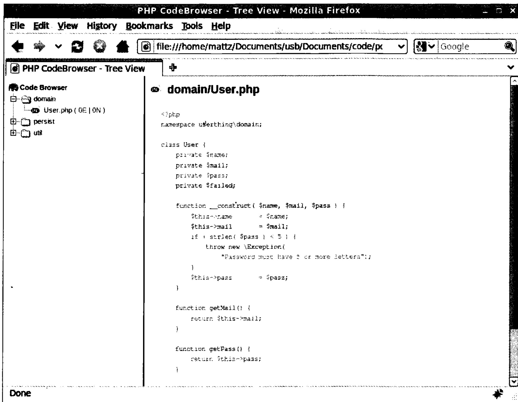
Рис. 20.3. Браузер PHP-кода
