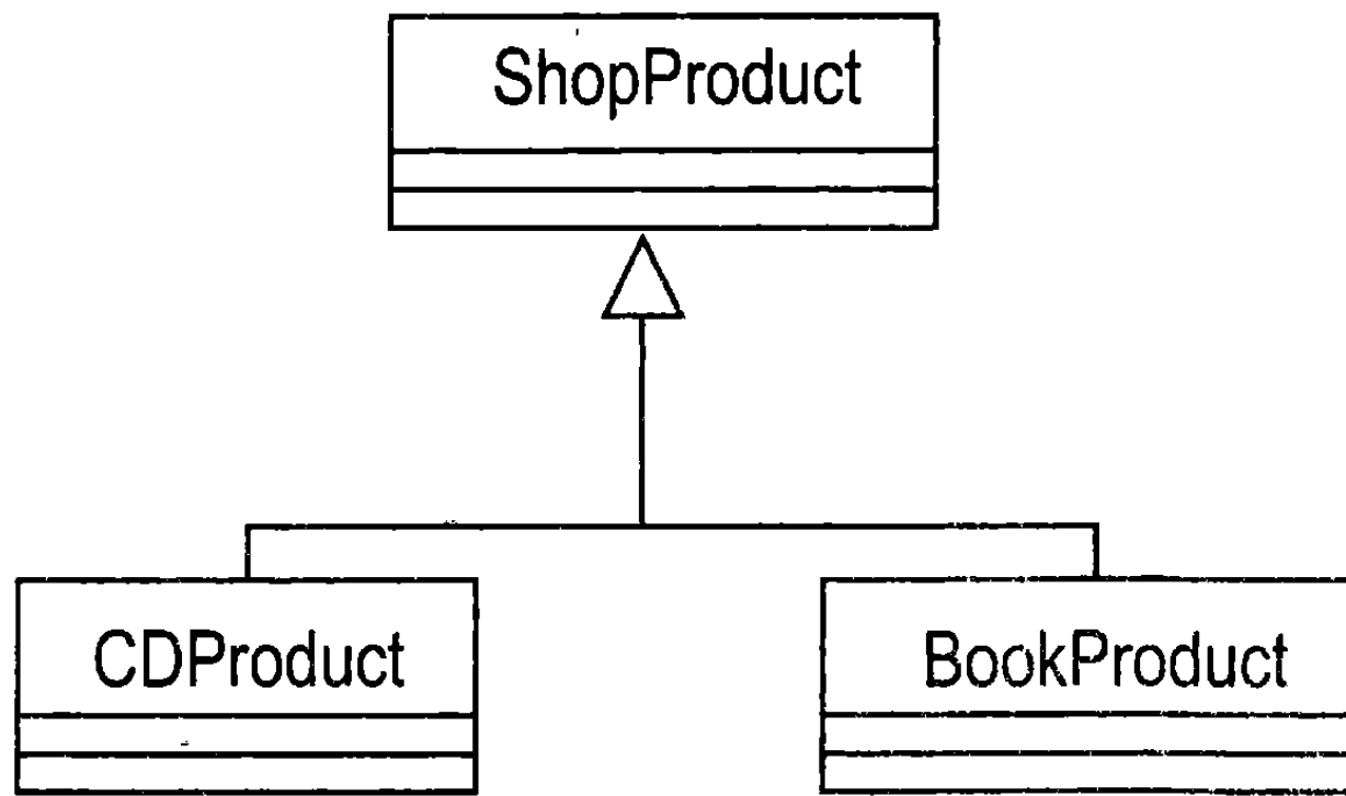
Рис. 6.7. Описание наследования
