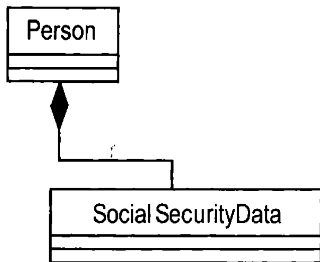
Рис. 6.15. Композиция
