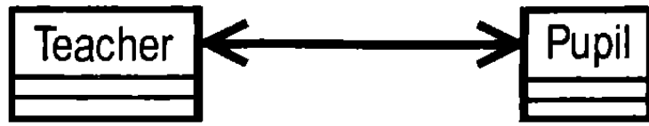
Рис. 6.11. Двухнаправленная ассоциация
