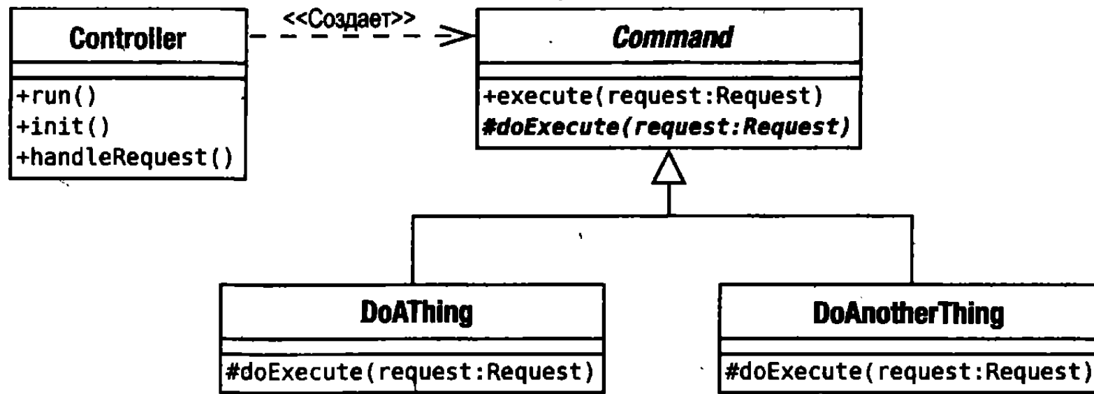
Рис. 12.4. Класс Controller и иерархия команд
