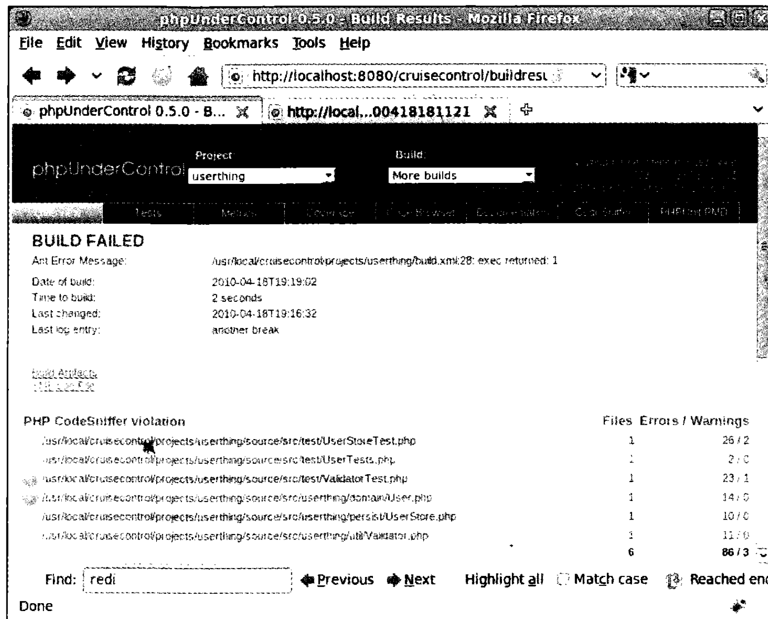
Рис. 20.10. Уведомление об ошибке в процессе построения проекта
