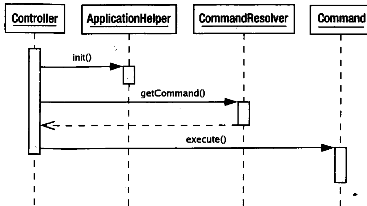
Рис. 12.5. Шаблон Front Controller в действии
