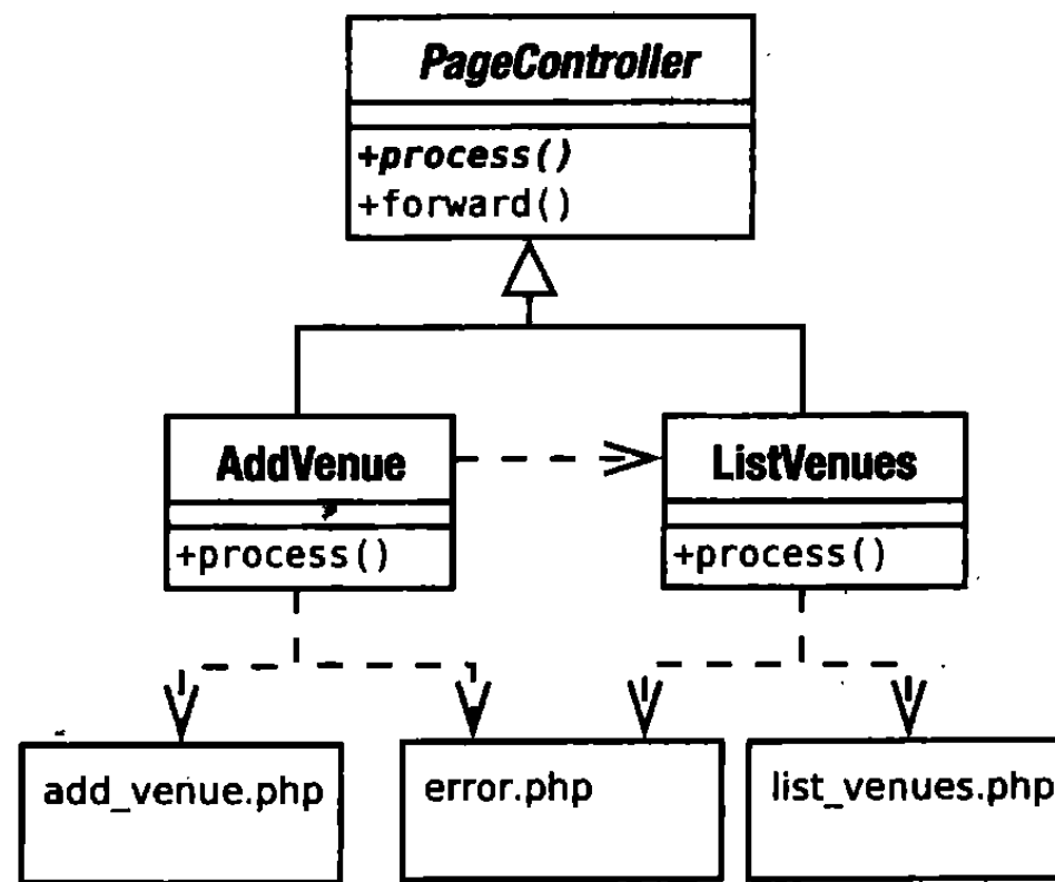
Рис. 12.9. Иерархия класса PageController и его включаемые взаимосвязи
