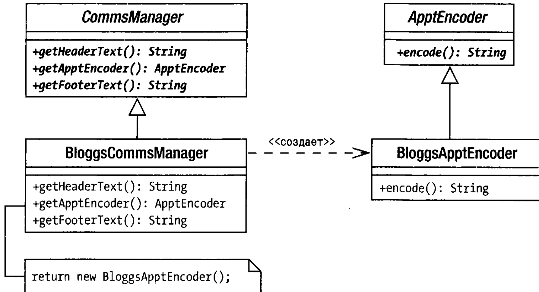
Рис. 9.4. Конкретные классы создателя и продукта
