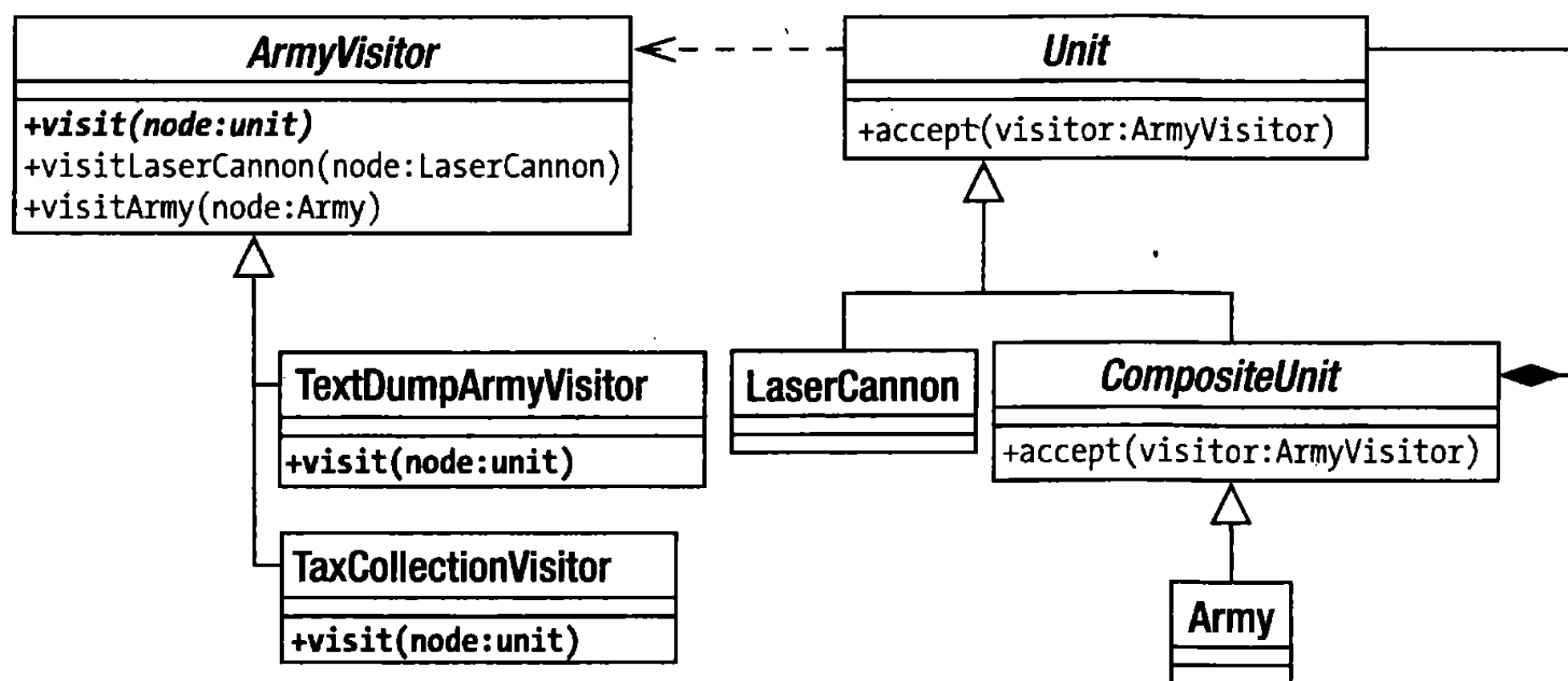
Рис. 11.7. Шаблон Visitor
