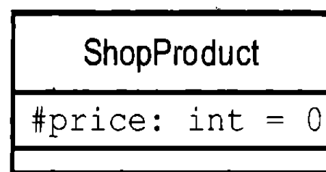
Рис. 6.5. Представление атрибута
