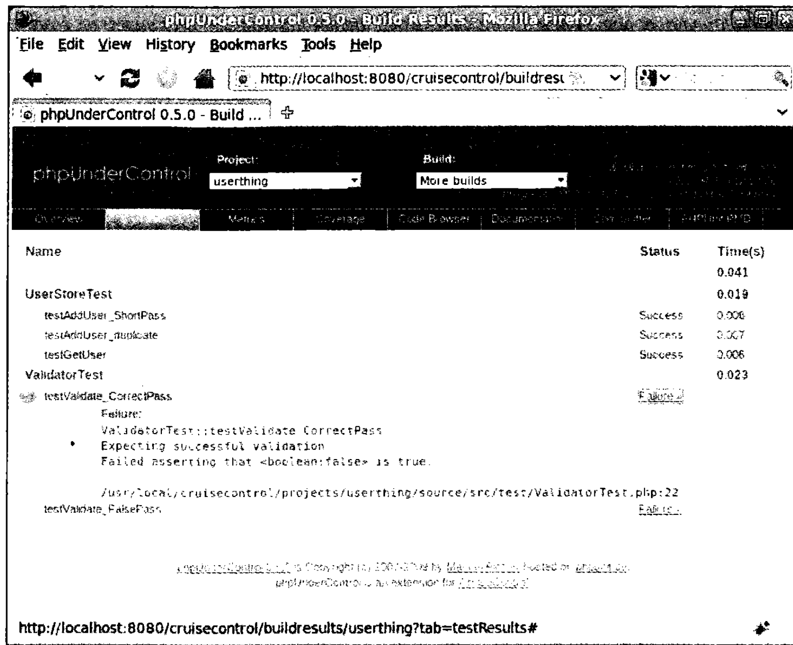
Рис. 20.9. Неудачное тестирование
