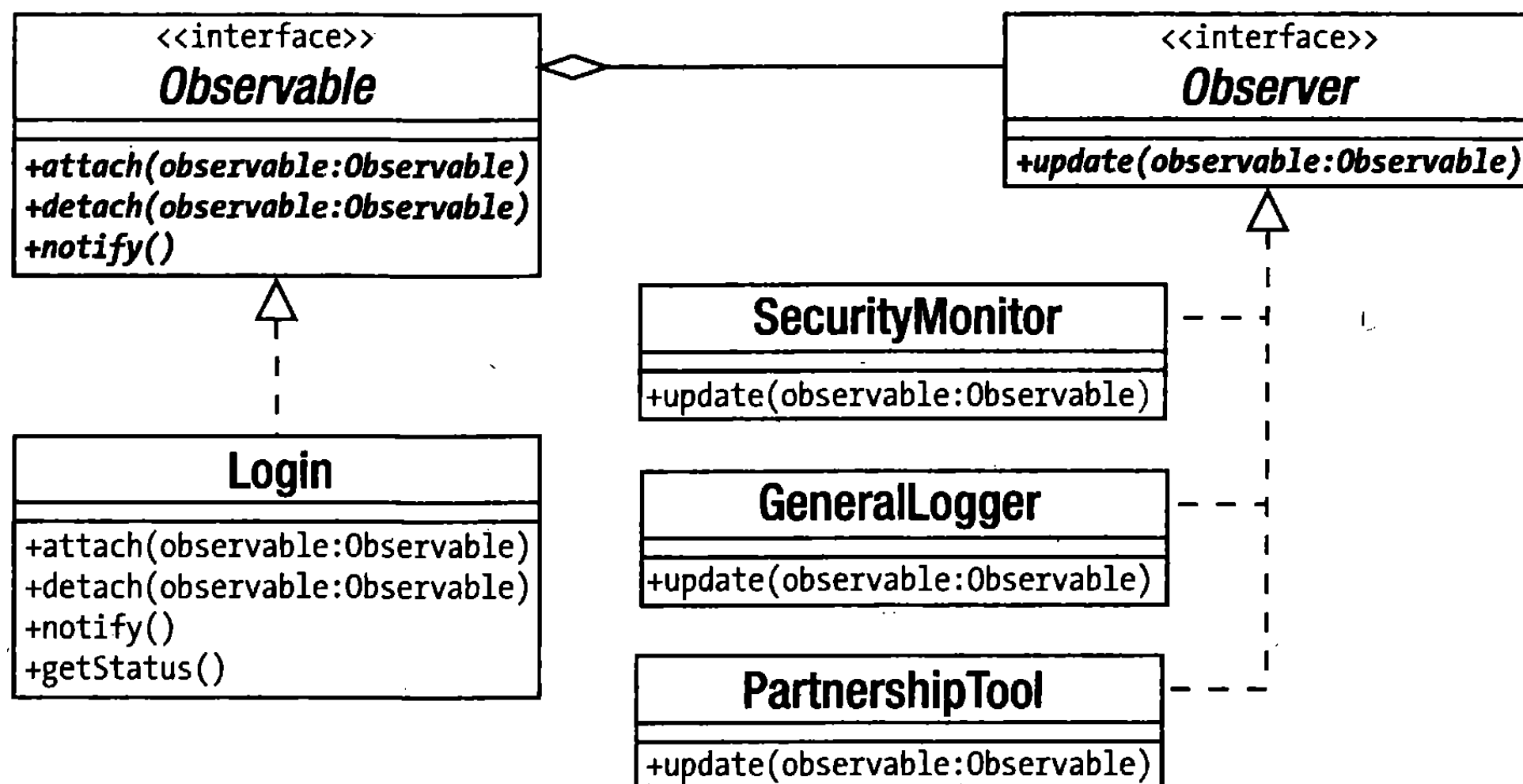
Рис. 11.6. Шаблон Observer
