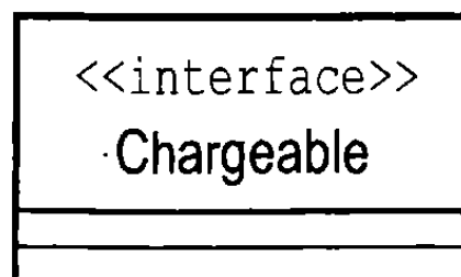
Рис. 6.4. Представление интерфейса
