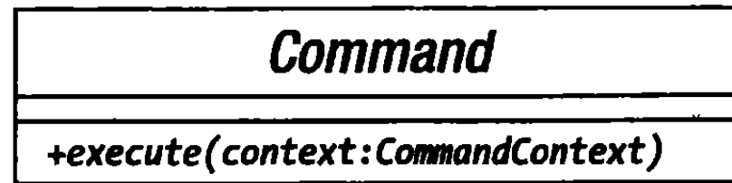
Рис. 11.8. Класс Command
