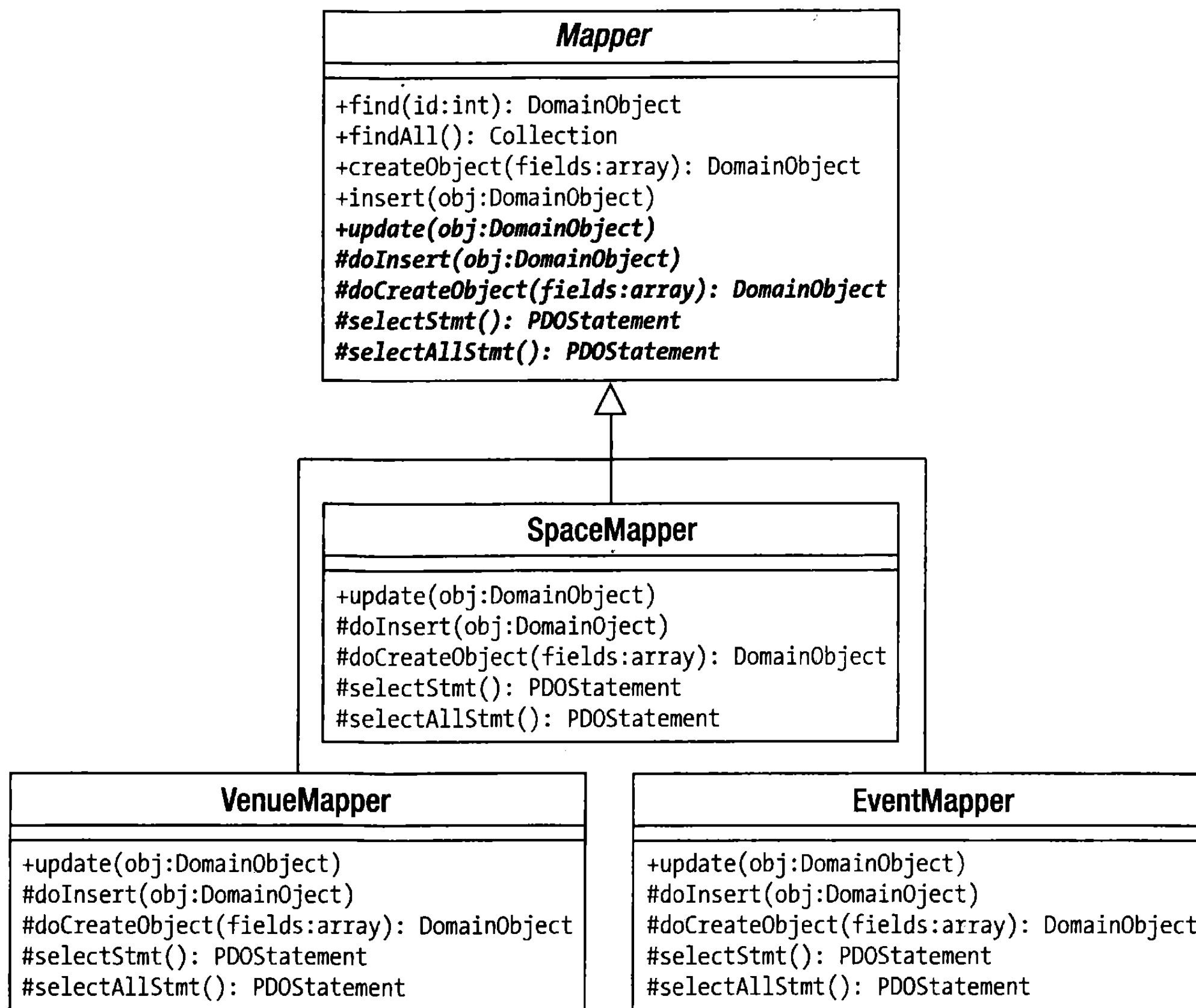
Рис. 13.1. Классы Mapper
