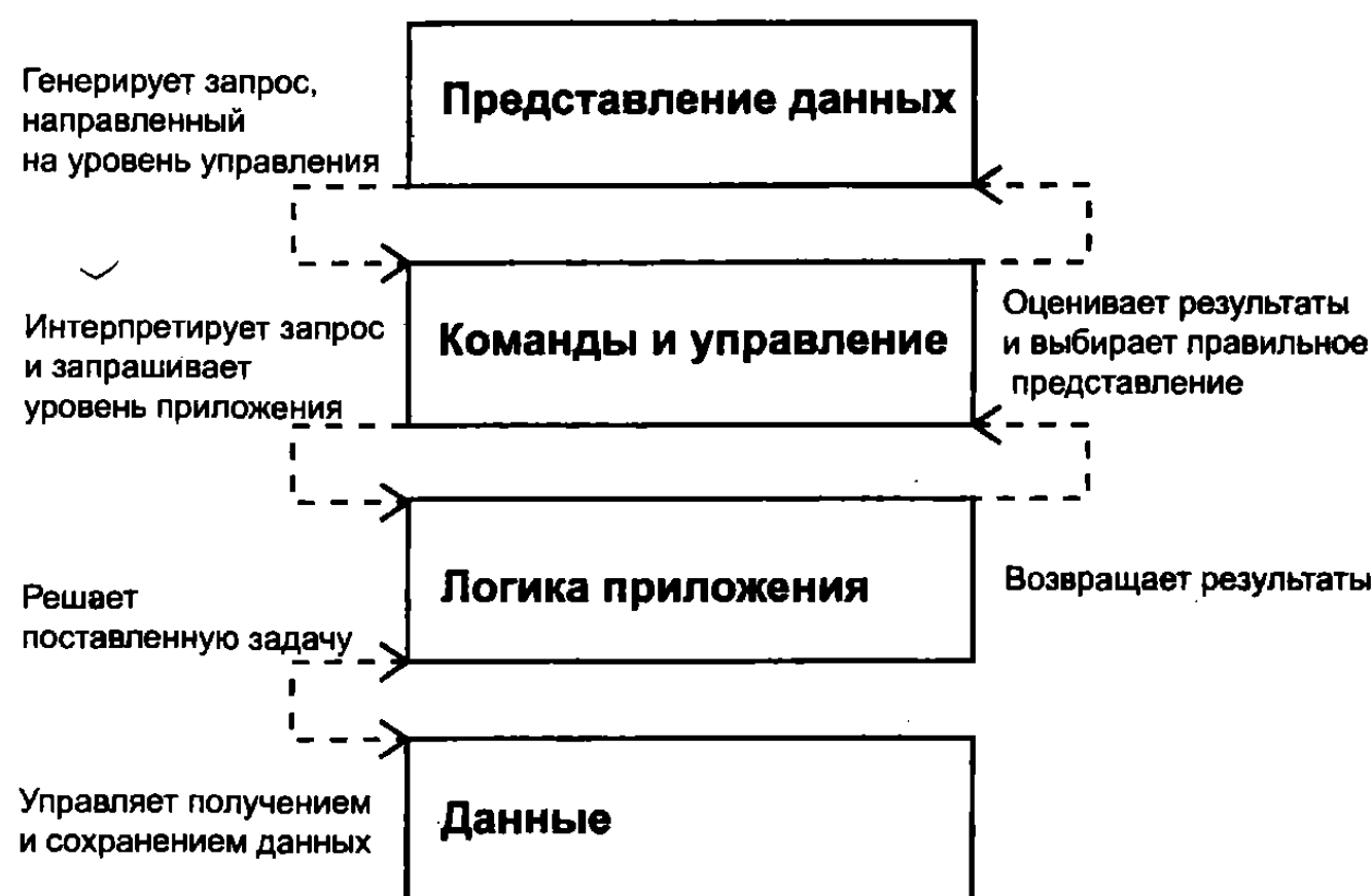
Рис. 12.1. Уровни типичной корпоративной системы
