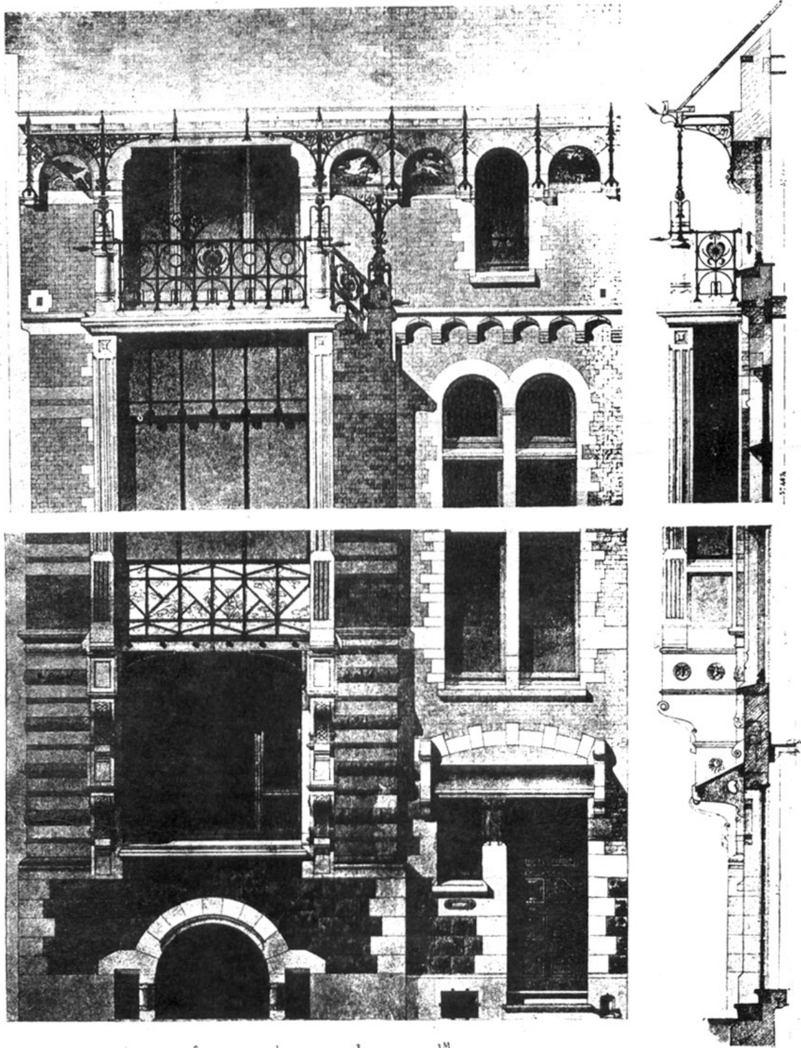
Разрѣзъ и деталь фасада.
