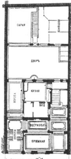
Планъ 2-го этажа.
