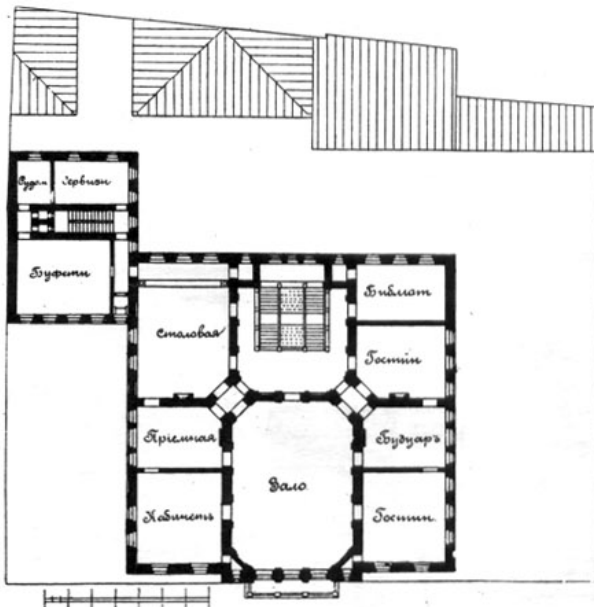
Планъ 2-го этажа.
