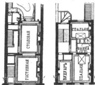
Планъ 1-го этажа. Планъ 2-го этажа.
