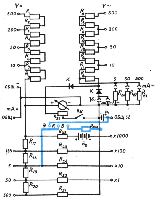
Рис. 4. Авометр «Школьный». Его «новая» схема.
