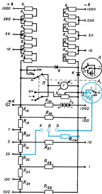
Рис. 1. Схема переделанного авометра ТТ-1.
