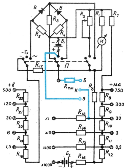
Рис. 3. Подключение гнезд к схеме прибора Ц-20.
