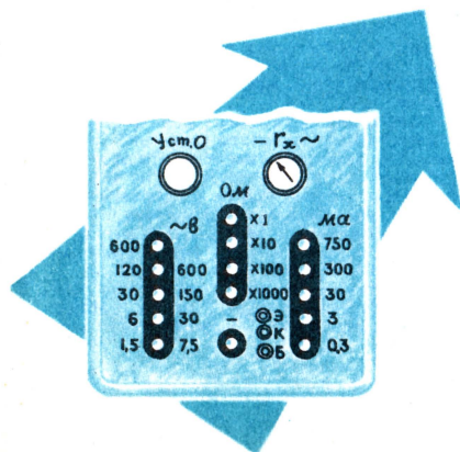
Рис. 2. Расположение гнезд проверки транзисторов на приборе Ц-20.
