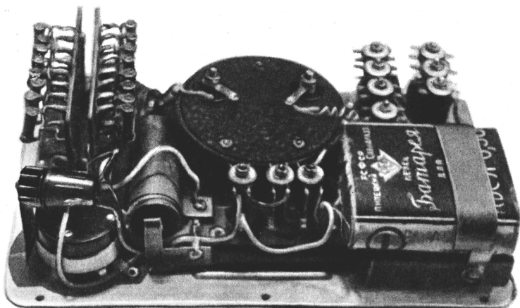
Рис. 5. Расположение детали после переделки.
