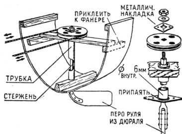
Подводный руль.
