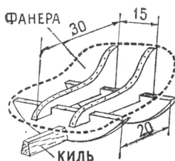
Построение кокпита.
