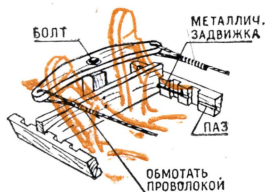
Планочное управление.
