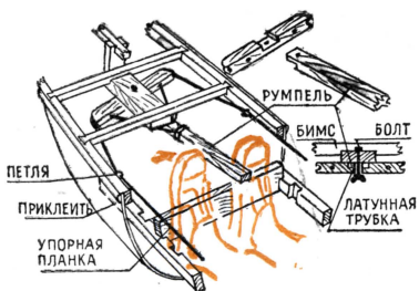
Румпельное управление.
