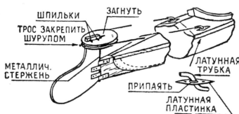
Надводный руль.
