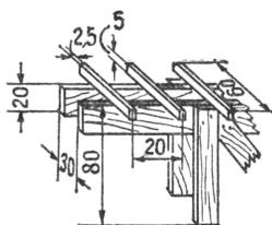
Стапель.
