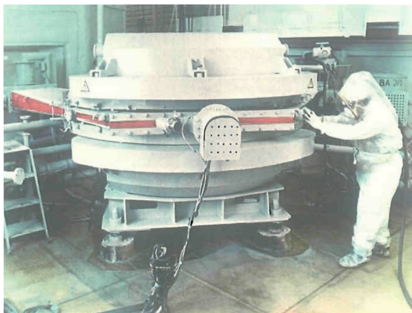
Уникальный электромагнитный масс-сепаратор С-2 для получения высокообогащенных радиоактивных изотопов (ВНИИЭФ)
