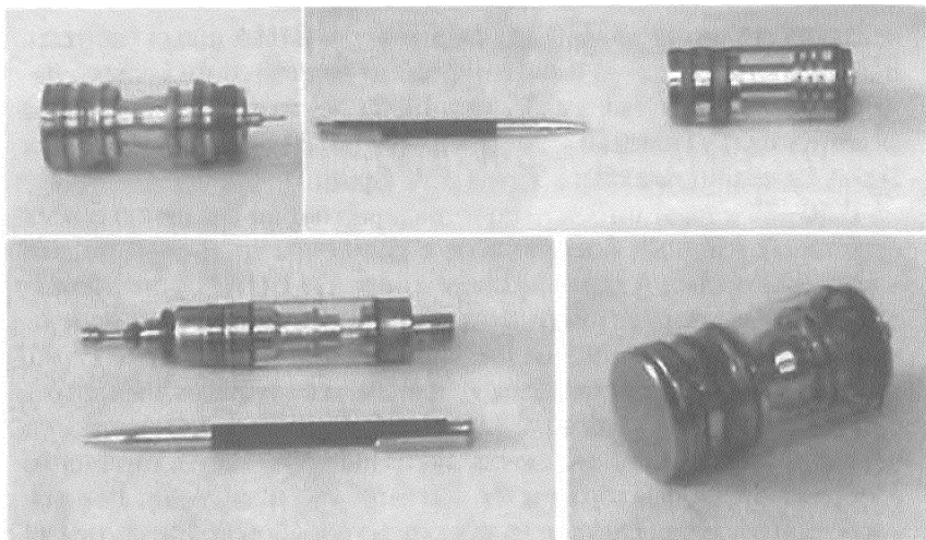
Нейтронные трубки для ядерно-физической и геофизической аппаратуры
