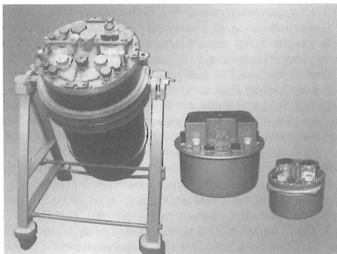
Автоматика подрыва и нейтронного иницирования первых трех поколений
