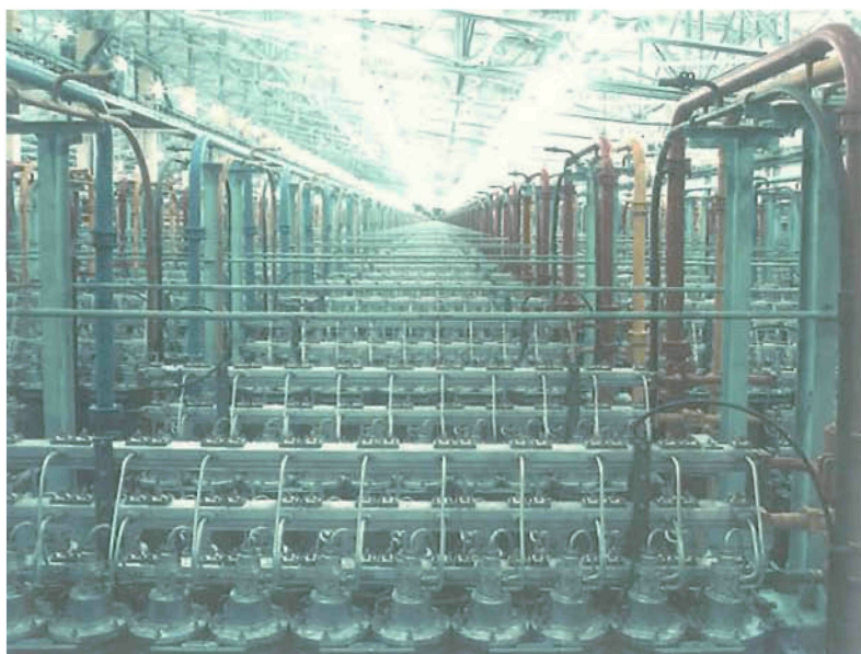
Один из центрифужных модулей обогатительного производства
