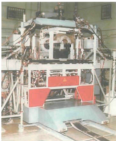
Быстрый атомный реактор самогасящийся «БАРС-5» (ВНИИТФ)
