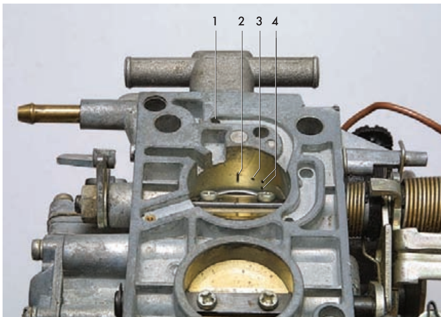
Вид на карбюратор 21073-1107010 со стороны дроссельных заслонок:
