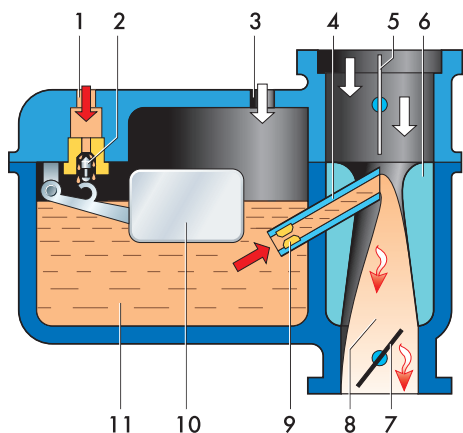
Схема простейшего карбюратора:
