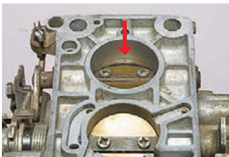
Выходное отверстие переходной системы второй камеры
