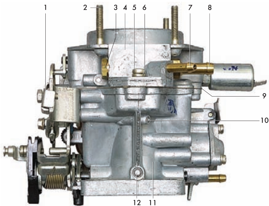
Вид на карбюратор со стороны второй камеры:
