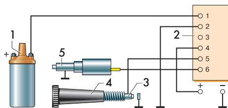
Схема подключения ЭПХХ:
