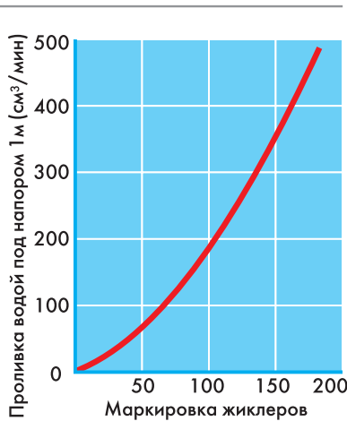
Зависимость пропускной способности жиклеров при проливке водой (в см 3 /мин) от численной маркировки
