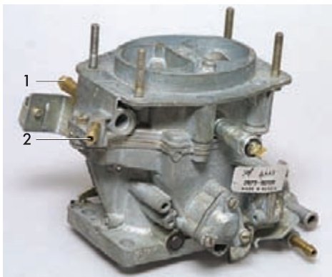
Карбюратор 21073-1107010: 1 – топливоподводящий штуцер; 2 – топливоотводящий штуцер
