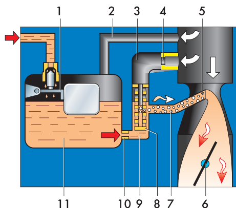
Схема главной дозирующей системы:
