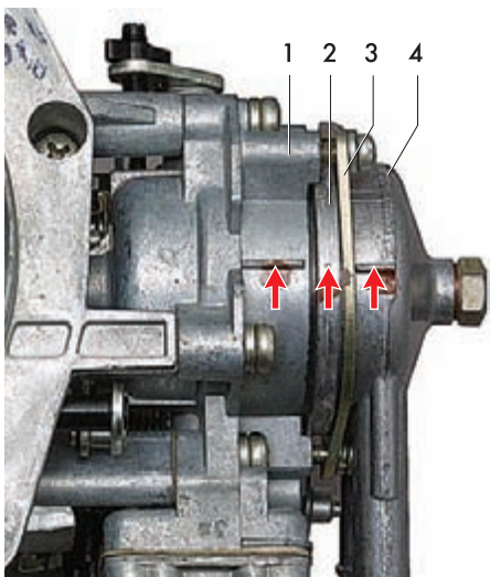
Установка биметаллической пружины пускового устройства: 1 – корпус пускового устройства; 2 – корпус биметаллической пружины; 3 – хомут; 4 – жидкостная камера
