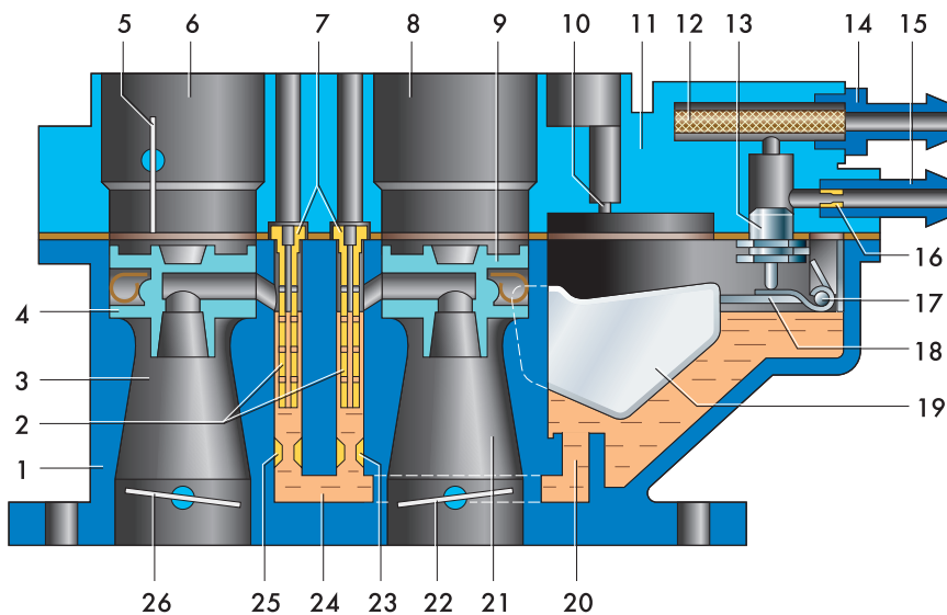
Схема главных дозирующих систем:
