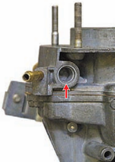
Карбюратор 21073-1107010: Неиспользуемое глухое отверстие
