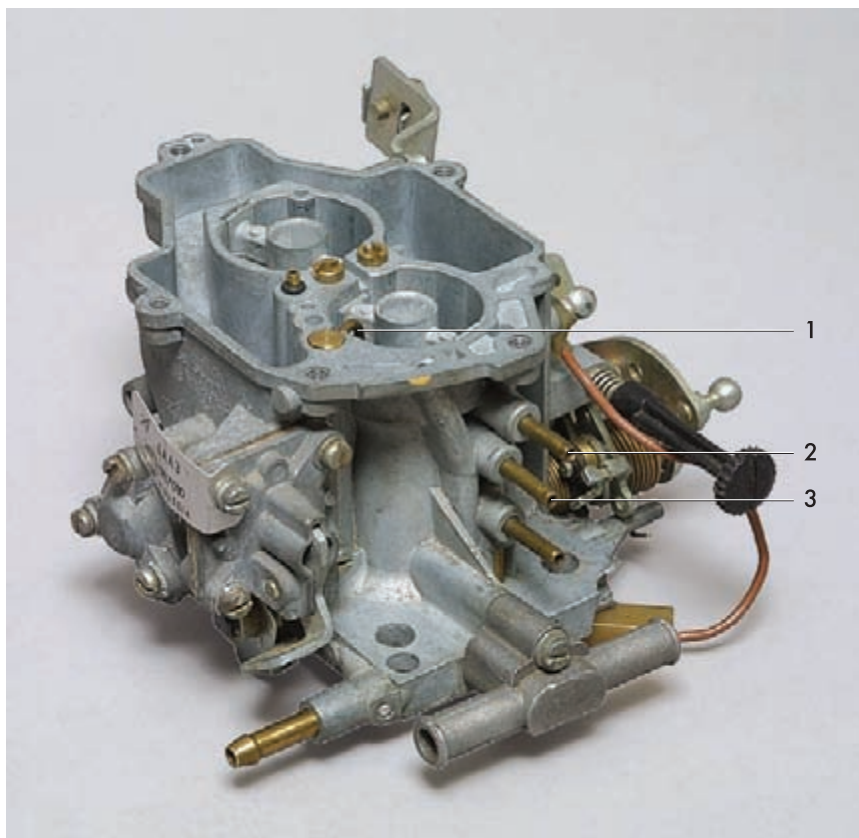
Вид на карбюратор 21073-1107010 со снятой крышкой:
