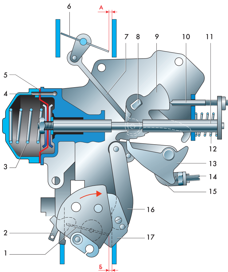
Схема автоматического пускового устройства карбюратора:
