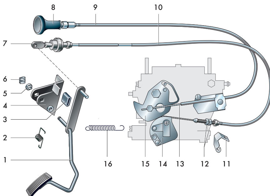
Привод управления карбюратором автомобилей «Самара»:
