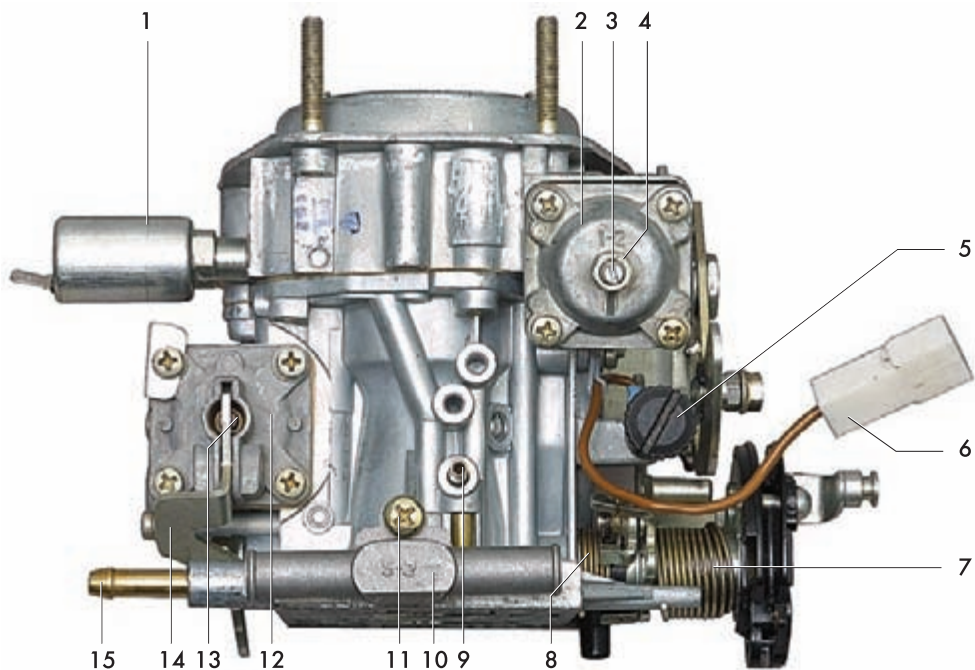
Вид на карбюратор со стороны первой камеры:
