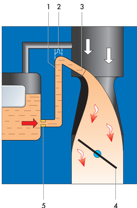
Схема экономайзера:
