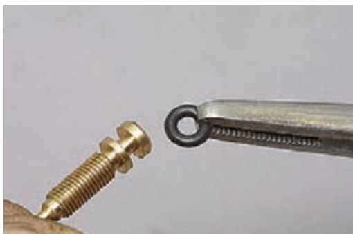
Снимаем с иглы резиновое уплотнительное кольцо.
