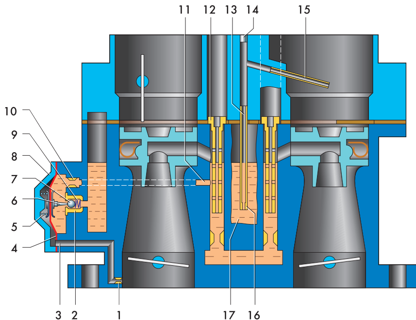
Экономат и экономайзер мощностных режимов:
