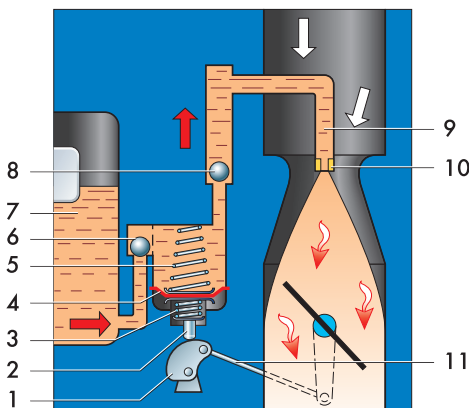
Схема диафрагменного ускорительного насоса:
