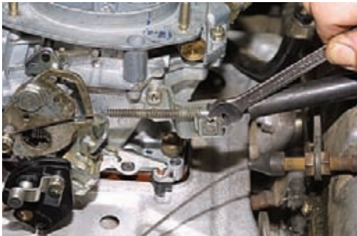
Ключом «на 8» отворачиваем болт крепления оболочки тяги.
