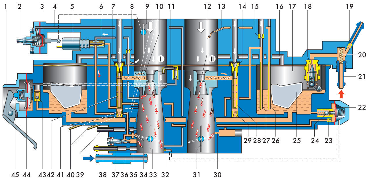
Схема устройства карбюратора 21073-1107010:
