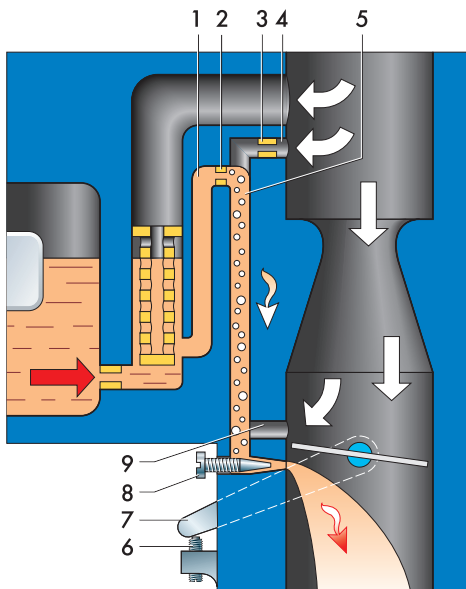
Схема системы холостого хода и переходной системы:
