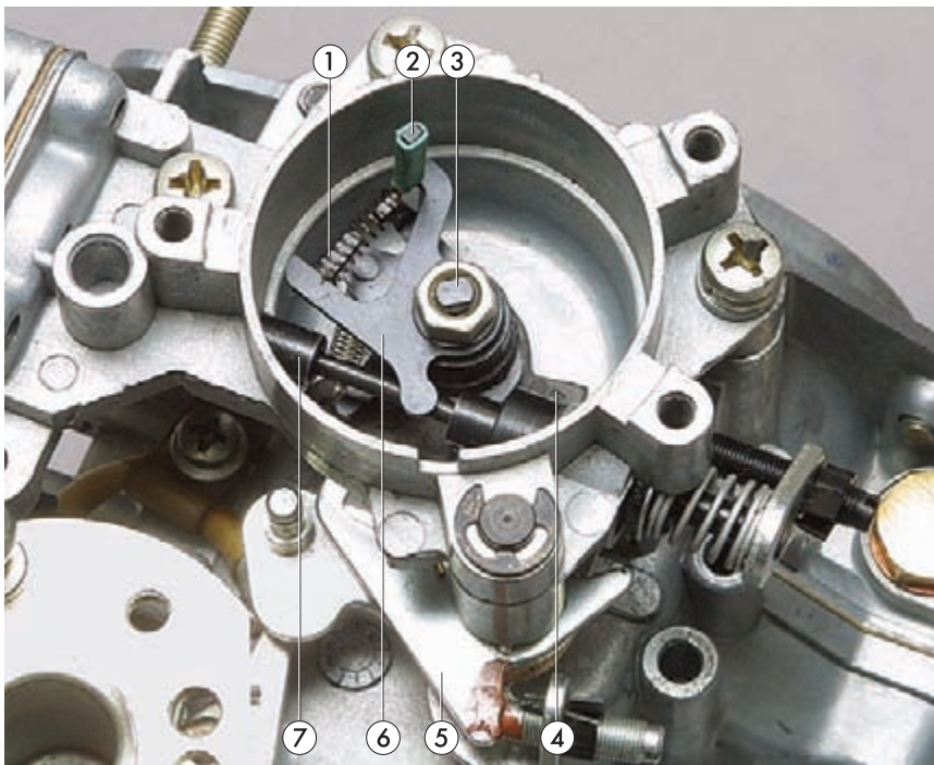
Автоматическое пусковое устройство со снятым нагревательным элементом: 1 – пружина; 2 – рычаг управления пусковым устройством; 3 – ось блока рычагов автоматического пускового устройства; 4 – кулачок; 5 – рычаг-упор; 6 – трехплечий рычаг (рычаг привода пускового устройства); 7 – шток диафрагмы
