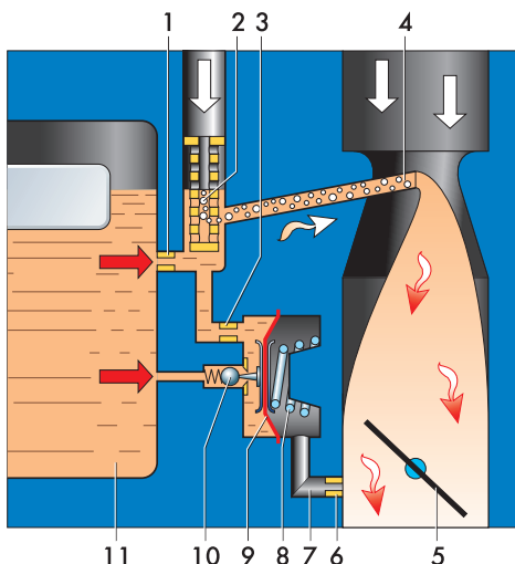
Схема экономайзера мощностных режимов с пневмоприводом:
