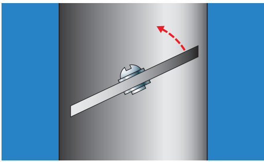
Положение заслонки в смесительной камере карбюратора
